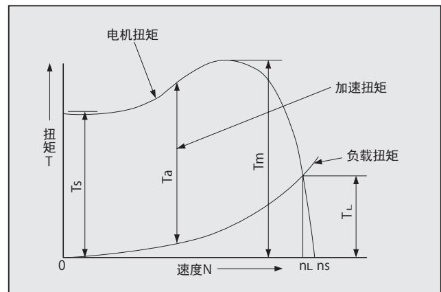
图 E1 扭矩曲线图
