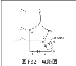
普通制动电路
