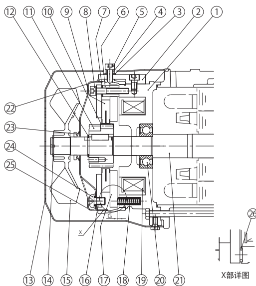
图 G16 FB-1E (室外型、释放螺栓方式)
