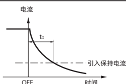
图 G9 电流衰减曲线
