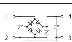
图 G12 面向美国·加拿大 230/460V、面向韩国 220/380V
