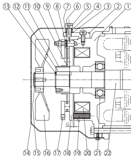
图 F42 FB-5E、FB-8E (室内型)
