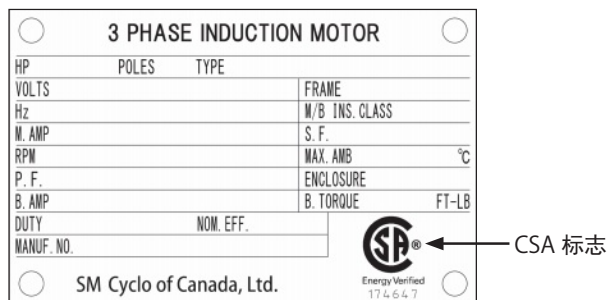
CSA 规格 铭牌例
