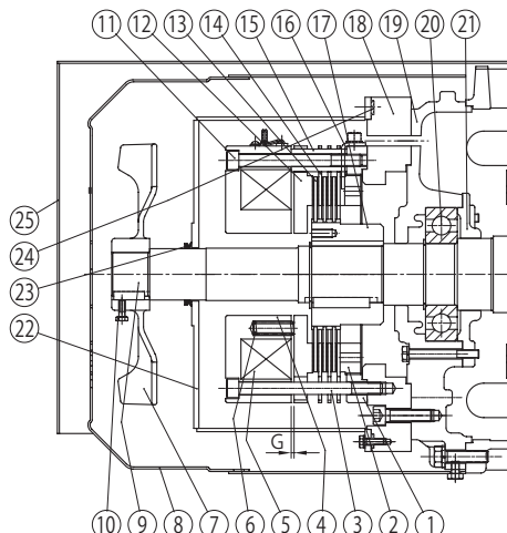
图 G27 ESB-250、ESB-250-2 (室外型)
