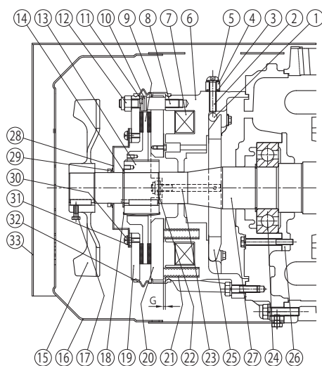
图 G26 FB-30 (室外型、释放螺栓方式)
