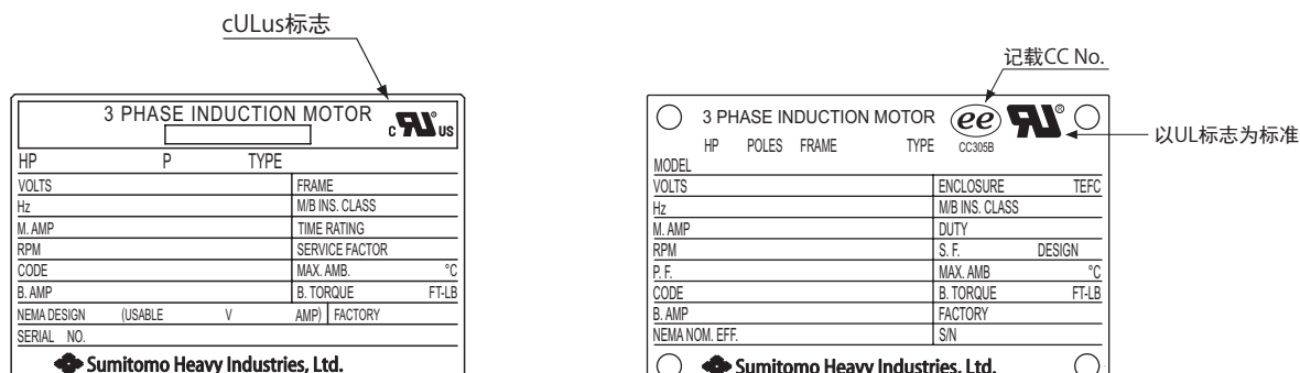
UL·NEMA 规格 铭牌例
