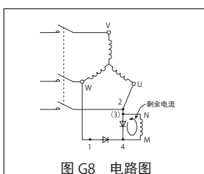
图 G8 电路图
