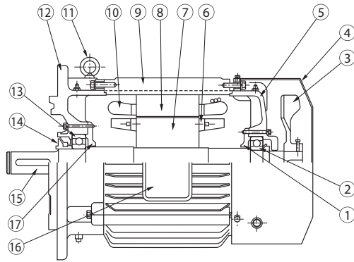
图F6 180机座以上的结构例
