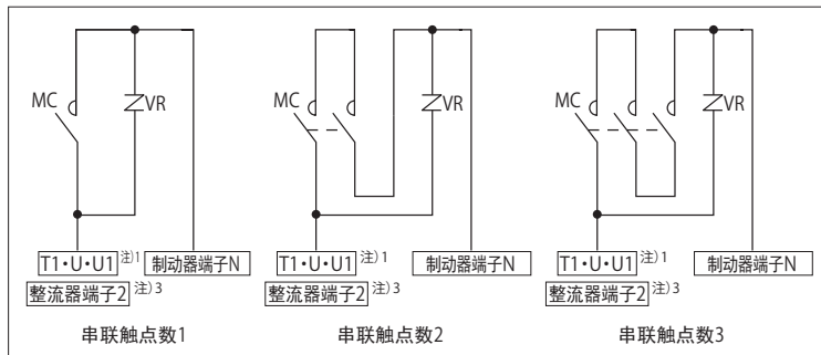
图 G7 紧急制动电路中的触点连接例
