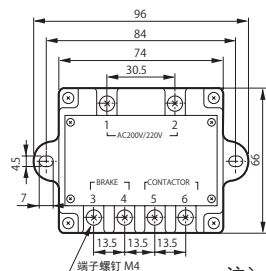
图 G28 附属整流器(直流电源装置) HD-110M3 型
