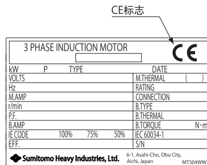
面向新加坡 CE 规格 铭牌例
