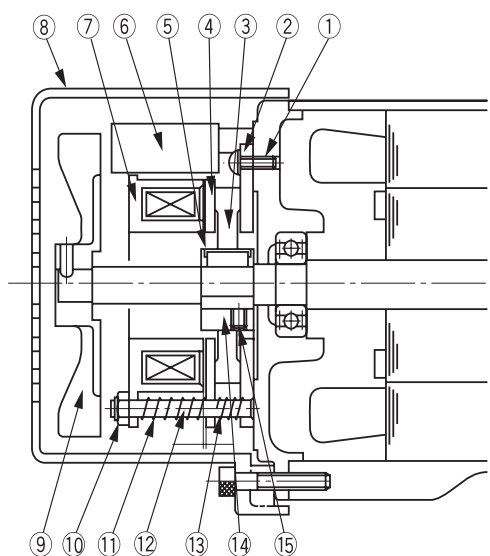
图 G14-2 MB-003、005 (40W~90W×4P)
