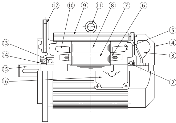
图F5 80-112M机座的结构例
