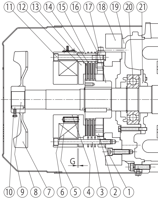
图 F46 ESB-250、ESB-250-2 (室内型)
