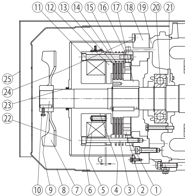
图 F57 ESB-250、ESB-250-2 (室外型)
