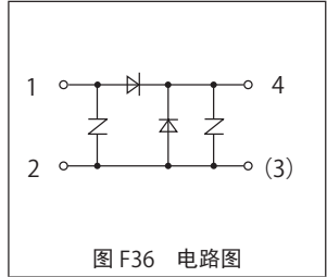
整流器内部电路图（参考）
