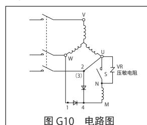
图 G10 电路图
