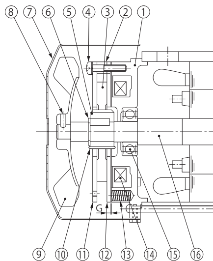
图 F37 FB-01A1、FB-02A1、FB-05A1 (室内型) (FB-01A1 无风扇)
