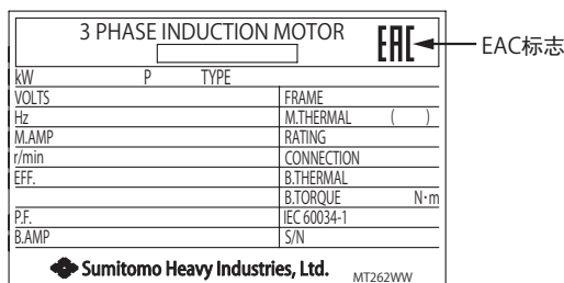
EAC 规格 铭牌例
