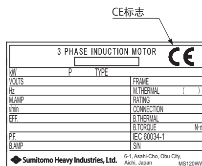
CE 规格 铭牌例
