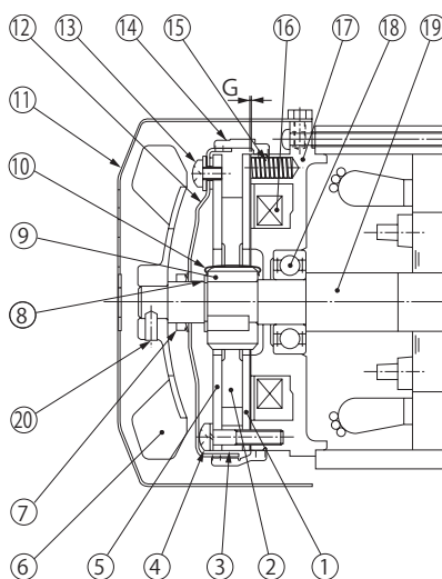
图 F48 FB-01A1、FB-02A1、FB-05A1 (室外型) (FB-01A1 无风扇)
