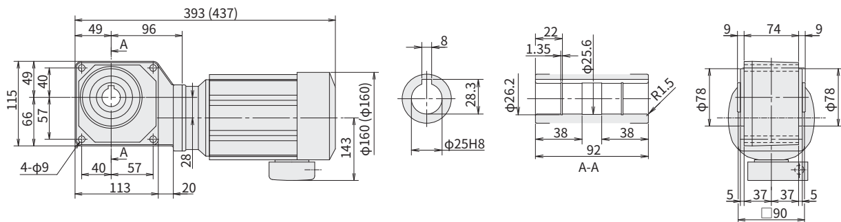
图 E159 RNYM05-1220-EP-5~30 (RNYM05-1220-EP-B-5~30) 重量 9.5kg (重量 11kg)
