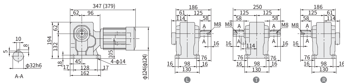
图 E394 RNHM02-40-AV-80~120 (RNHM02-40-AV-B-80~120) 重量 14kg (重量 15kg)
