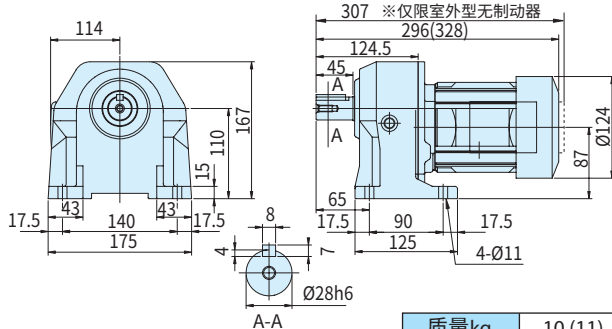
图C10 ZNHM02-1280-100~200 (ZNHM02-1280-B-100~200)
