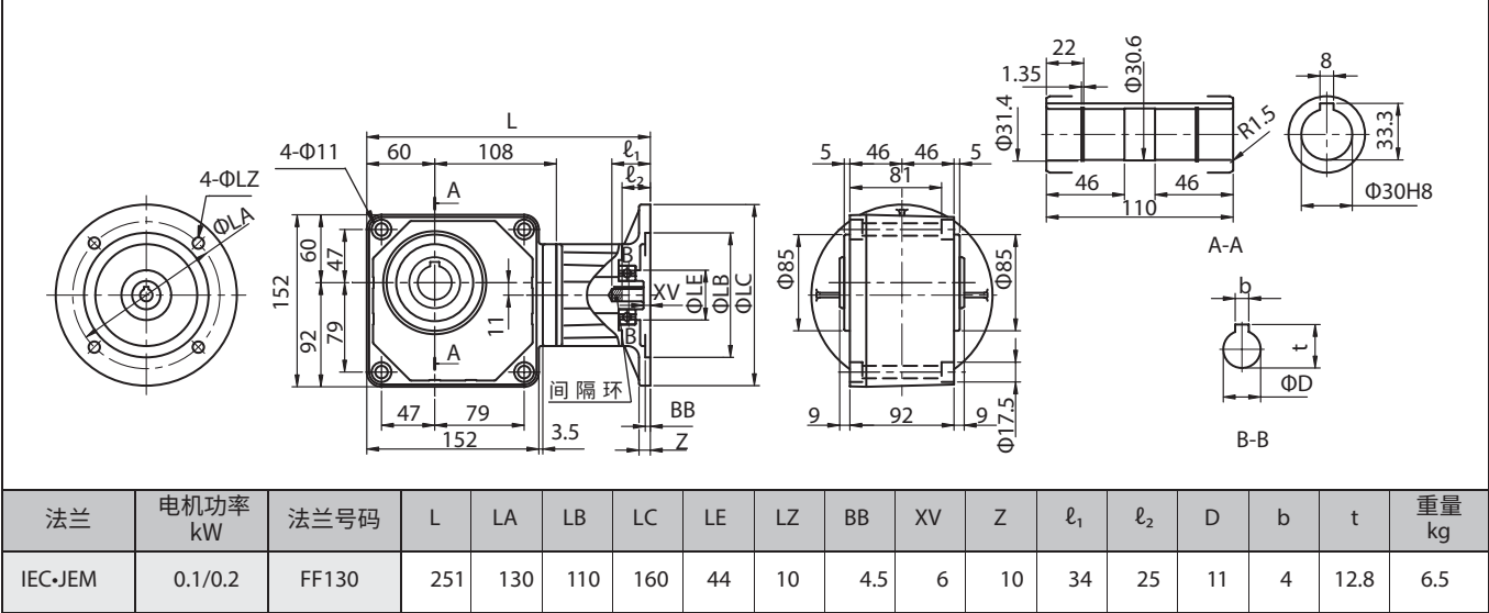
图 E409 RNYX - 1340 - [ 减速比 ]
