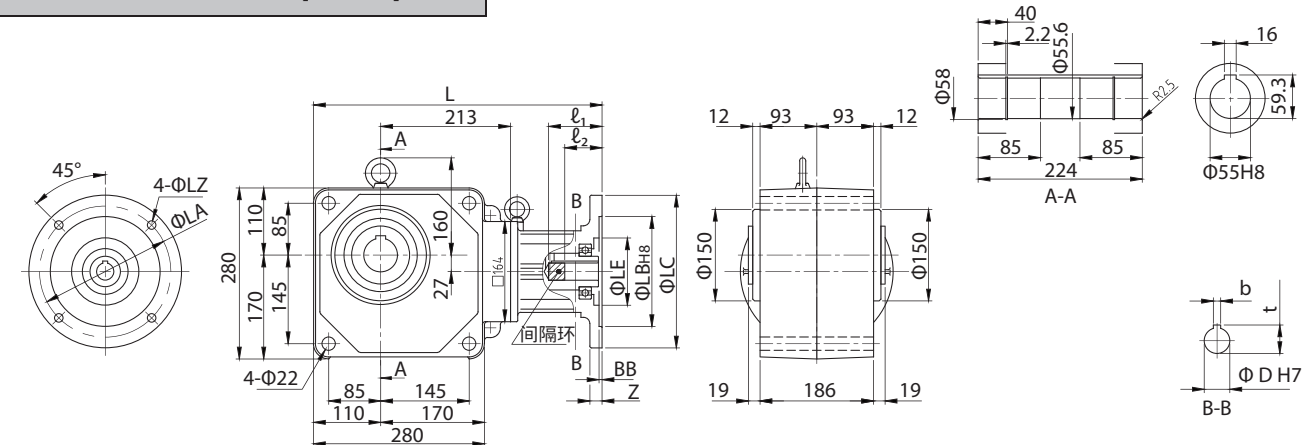
图 E417 RNYX - 1630 - [ 减速比 ]
