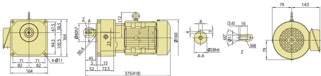
图 C87 ZNFM05-1281-AV-30~100 (ZNFM05-1281-AV-B-30~100)
