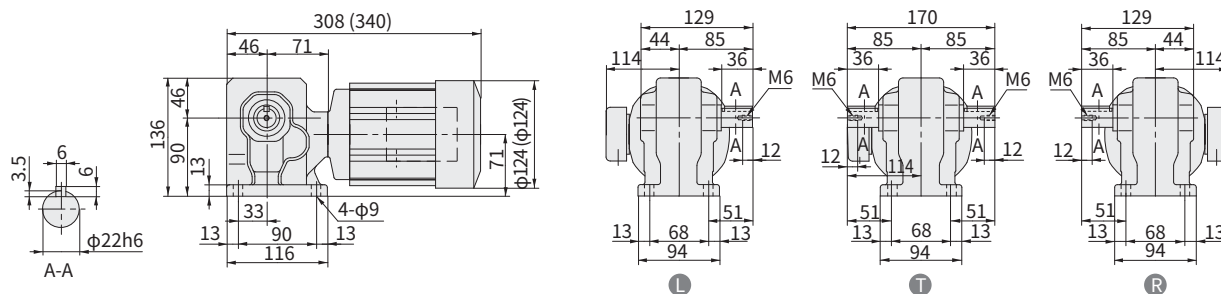
图 E392 RNHM02-270-AV-5~30 (RNHM02-270-AV-B-5~30) 重量 8.5kg (重量 10kg)
