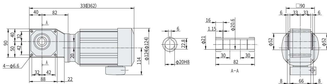
图 E140 RNYM02-1120-EP-5~15 (RNYM02-1120-EP-B-5~15)
