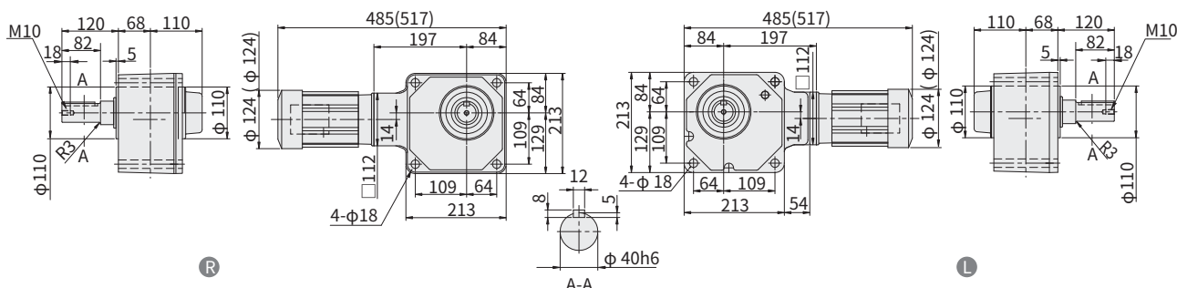
图 E248 RNFM05-1540 \frac{h}{B} -X1-300~480 重量 29kg (重量 30kg) • 安装本机器时请使用内六角螺钉 (M16)。
