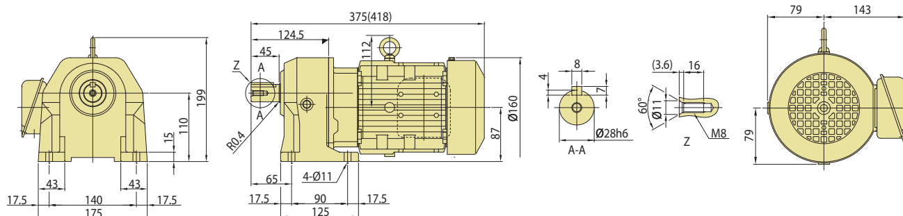
图 C46 ZNHM05-1281-EP-30~100 (ZNHM05-1281-EP-B-30~100)
