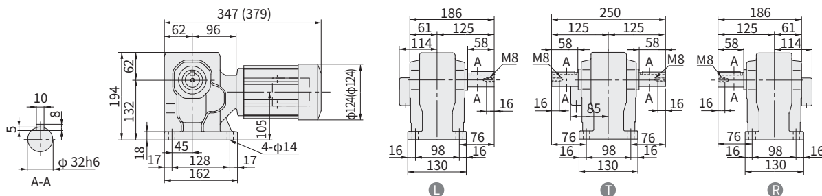
图 E362 RNHM05-40 h6 -80~120 (RNHM05-40 h6 -B-80~120) 重量 14kg (重量 15kg)
