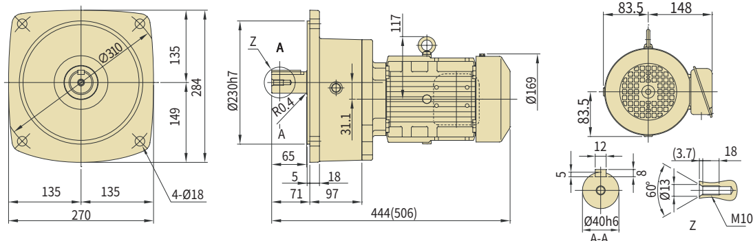
图 C95 ZNHM2-1320-AV-3~30 (ZNHM2-1320-AV-B-3~30)
