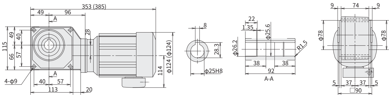
图 E32 RNYM05-1220-5~12 (RNYM05-1220-B-5~12) 重量 9.5kg (重量 11kg)
