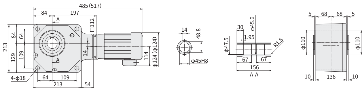
图 E30 RNYM03-1540-300~1440 (RNYM03-1540-B-300~1440) 重量 26kg (重量 27.5kg)
