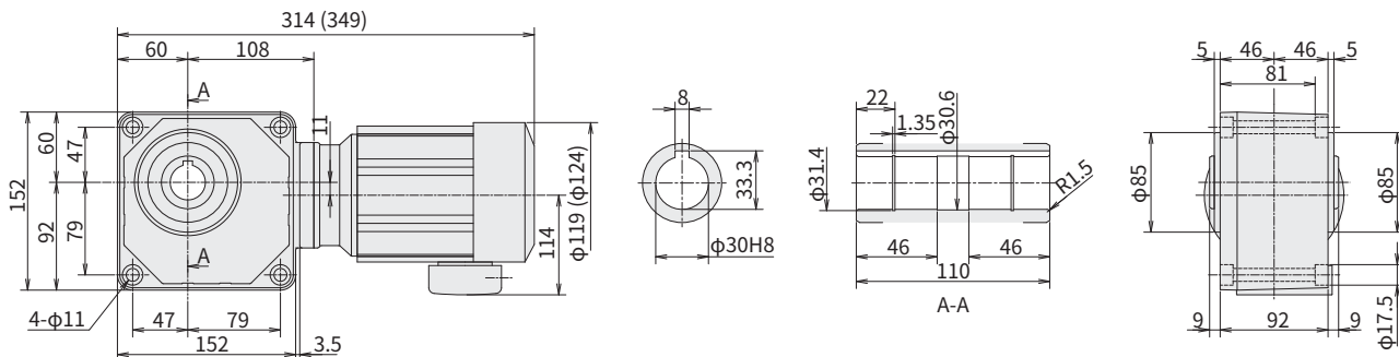
图 E13 RNYM01-1330-80~240 (RNYM01-1330-B-80~240) 重量 9.0kg (重量 10kg)
