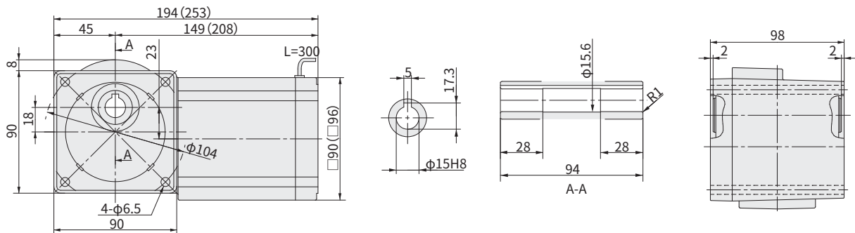
图 E7 RNYM009-17-5~240 (RNYM009-17-B-5~240) 重量 4.2kg (重量 4.6kg)
