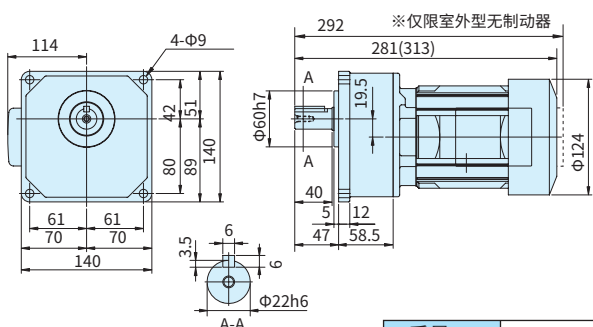
图C7 ZNFM02-1221-30~100 (ZNFM02-1221-B-30~100)
