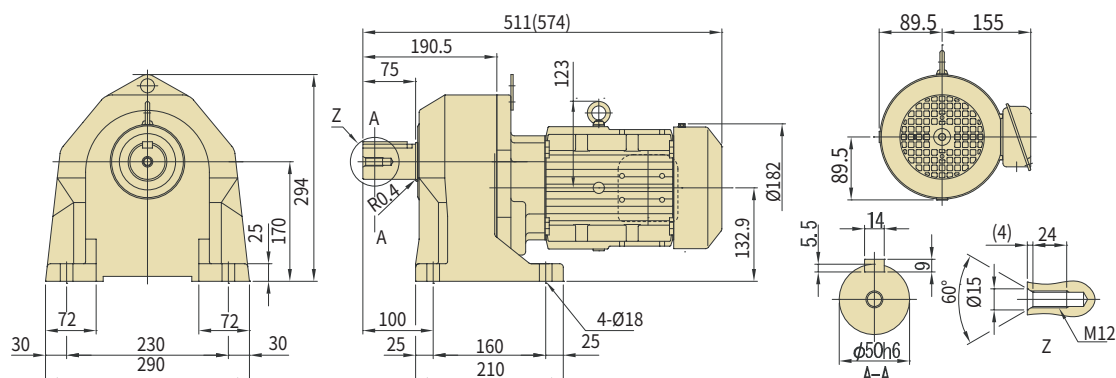
图 C97 ZNHM2-1500-AV-100~200 (ZNHM2-1500-AV-B-100~200)
