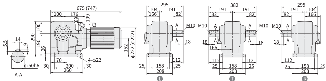
图 E383 RNHM8-64 \frac{1}{2} -10~40 重量 92kg (RNHM8-64 \frac{1}{2} -B-10~40) (重量 101kg)
