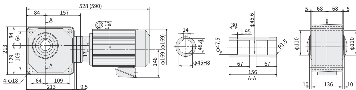
图 E125 RNYM1-1531-AV-80 重量 30kg (RNYM1-1531-AV-B-80) (重量 34kg)
