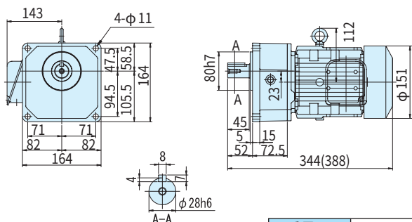
图C23 ZNFM1-1280-3~30 (ZNFM1-1280-B-3~30)
