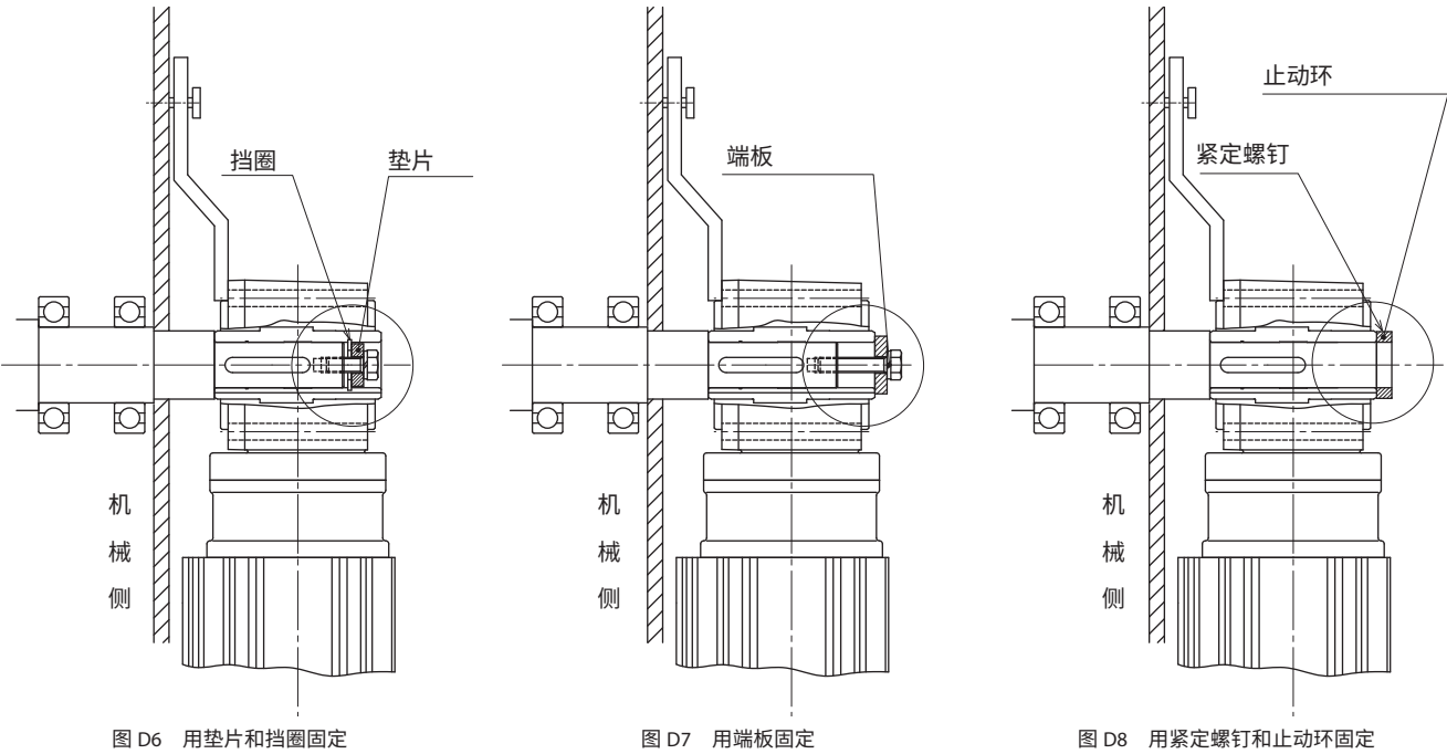
b) 防止减速机向机械相反侧移动的固定方法（例 图 D6~图 D8）
