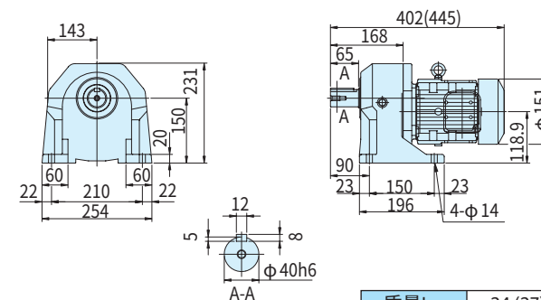
图C28 ZNFM1-1400-100~200 (ZNFM1-1400-B-100~200)
