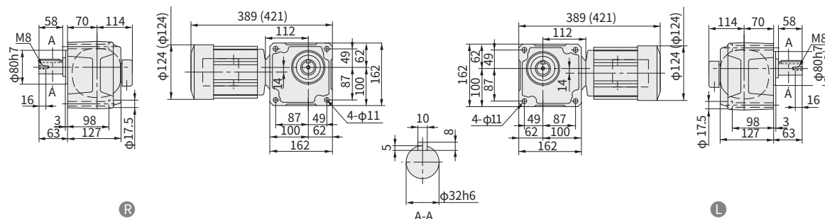
图 E312 RNFM03-45 L R -EP-150~240 重量 15kg (RNFM03-45 L R -EP-B-150~240) (重量 16kg) • 安装本机器时请使用内六角螺钉 (M10)。
