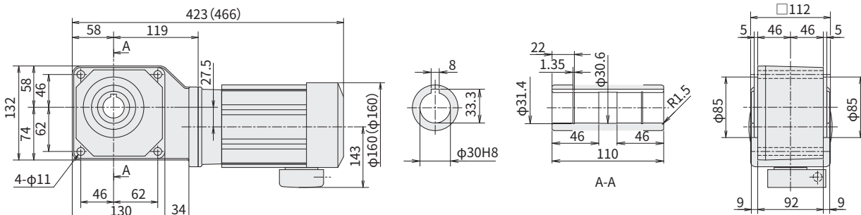
图 E161 RNYM05-1320-EP-40~60 (RNYM05-1320-EP-B-40~60) 重量 11kg (重量 13kg)
