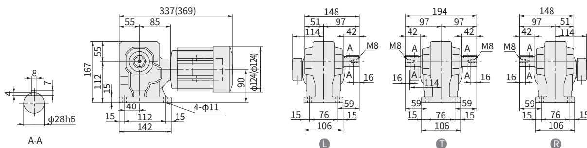
图 E393 RNHM02-33-AV-40~60 (RNHM02-33-AV-B-40~60) 重量 11kg (重量 12kg)
