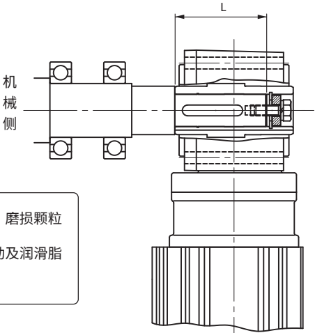
图D1 从动轴插入长度L
