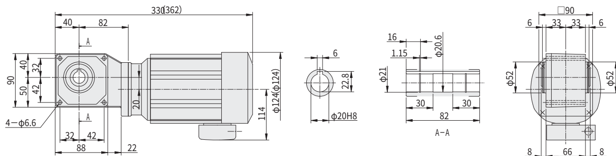
图 E142 RNYM02-1120-EP-20~30 (RNYM02-1120-EP-B-20~30)
