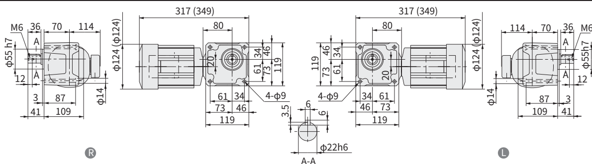
图 E309 RNFM03-270 L R -EP-5~30 重量 9.0kg (RNFM03-270 L R -EP-B-5~30) (重量 10.5kg) • 安装本机器时请使用内六角螺钉 (M8)。
