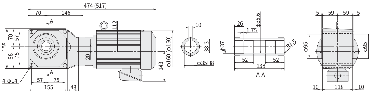
图 E162 RNYM05-1420-EP-40~60 (RNYM05-1420-EP-B-40~60) 重量 18kg (重量 20kg)
