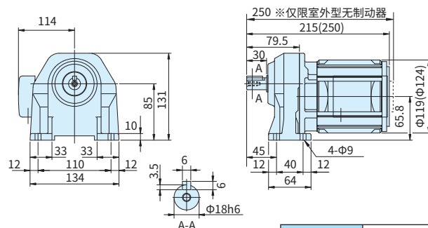
图C2 ZNHM01-1180-3~50 (ZNHM01-1180-B-3~50)
