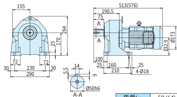
图C38 ZNHM3-1501-30~100 (ZNHM3-1501-B-30~100)
