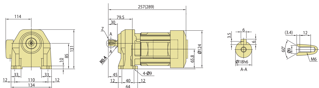
图 C73 ZNHM01-1180-AV-3~50 (ZNHM01-1180-AV-B-3~50)
