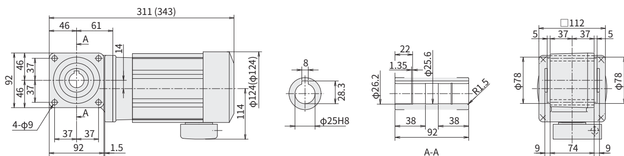
图 E105 RNYM02-1210-AV-5~10 (RNYM02-1210-AV-B-5~10) 重量 9.0kg (重量 10kg)
