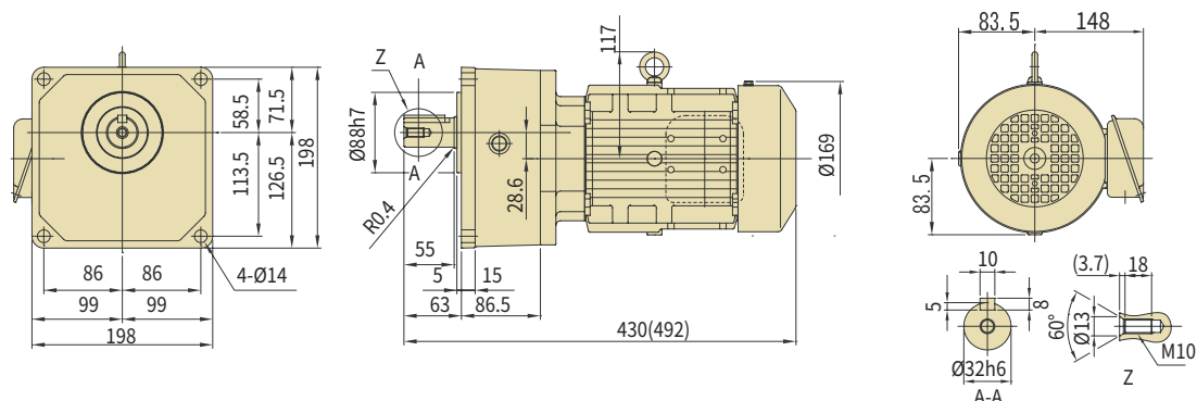
图 C93 ZNFM1-1321-AV-30~100 (ZNFM1-1321-AV-B-30~100)
