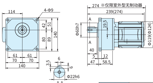
图C3 ZNFM01-1220-60~200 (ZNFM01-1220-B-60~200)
