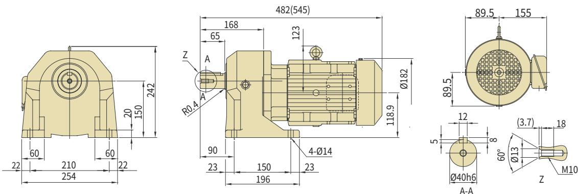
图 C96 ZNHM2-1401-AV-30~100 (ZNHM2-1401-AV-B-30~100)
