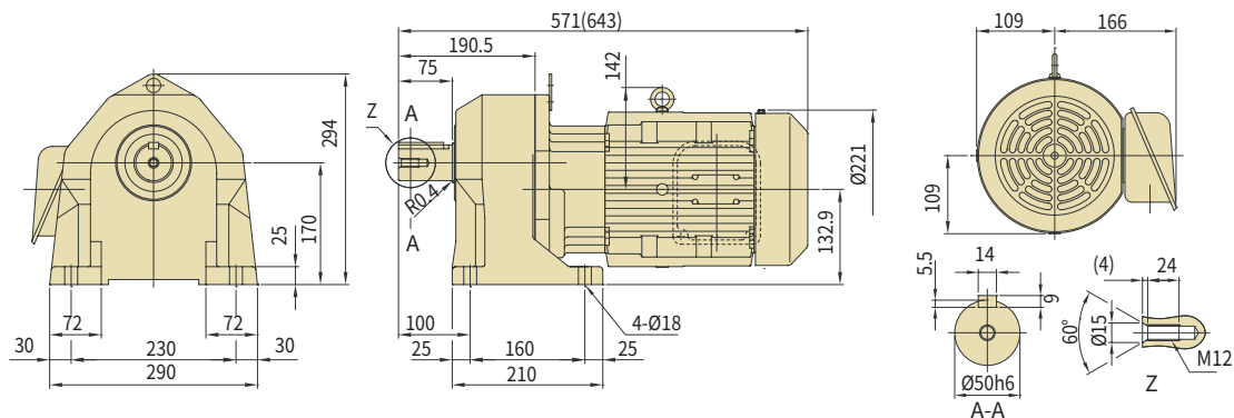
图 C102 ZNHM3-1501-AV-30~100 (ZNHM3-1501-AV-B-30~100)
