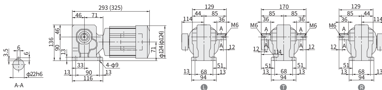
图 E385 RNHM01-23-AV-40~60 (RNHM01-23-AV-B-40~60) 重量 7.5kg (重量 9.0kg)
