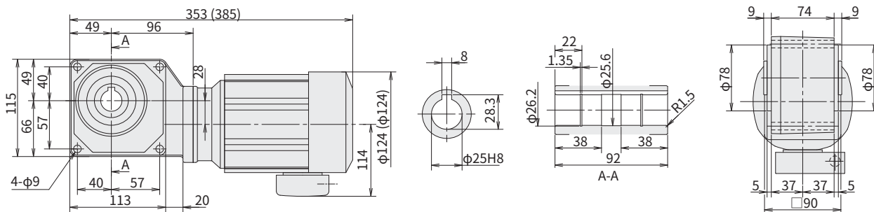
图 E34 RNYM05-1220-15~30 (RNYM05-1220-B-15~30)
