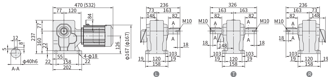
图 E374 RNHM1H-53 1 -40~80 (RNHM1H-53 1 -B-40~80) 重量 30kg (重量 34kg)
