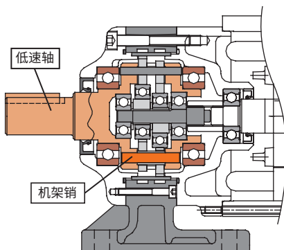
双支承结构
