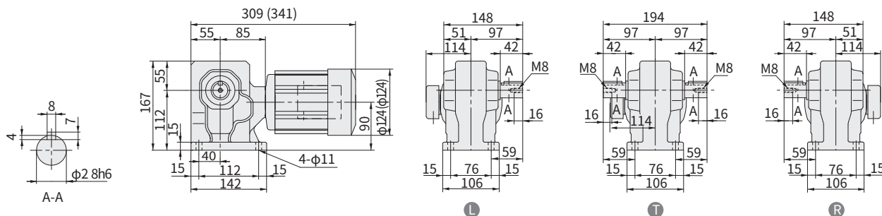
图 E386 RNHM01-30-AV-80~120 (RNHM01-30-AV-B-80~120) 重量 9.5kg (重量 11kg)
