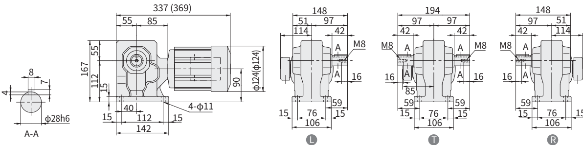
图 E361 RNHM05-33 h -40~60 重量 11kg (RNHM05-33 B -B-40~60) (重量 12kg)
