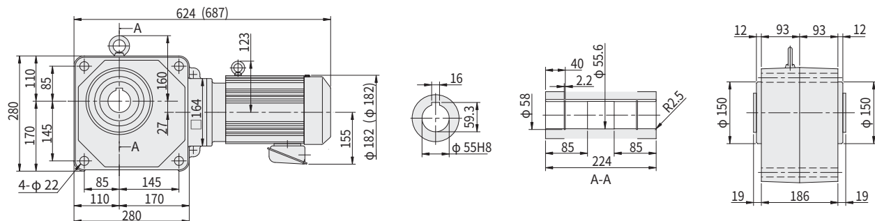
图 E132 RNYM2-1631-AV-150~240 (RNYM2-1631-AV-B-150~240)
