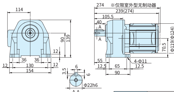
图C4 ZNHM01-1220-60~200 (ZNHM01-1220-B-60~200)
