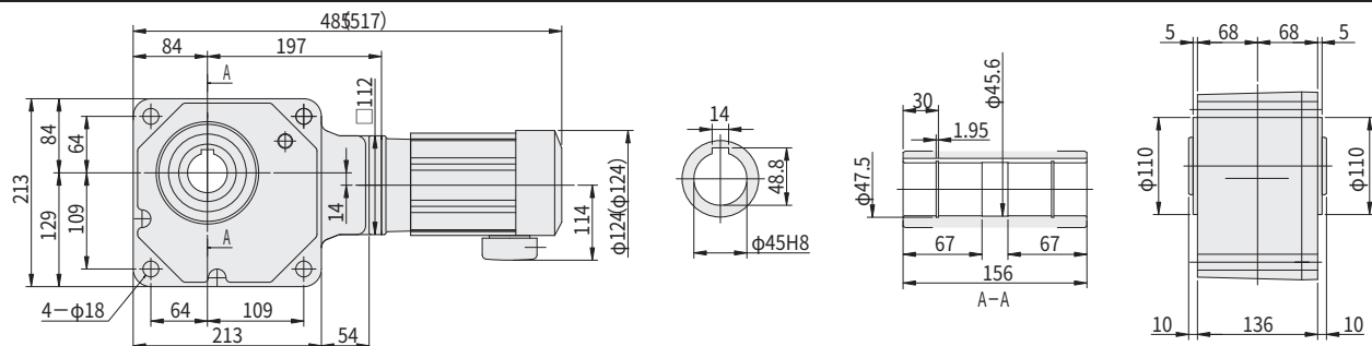
图 E116 RNYM02-1540-AV-720~1440 (RNYM02-1540-AV-B-720~1440) 重量 26kg (重量 27.5kg)
