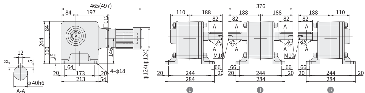
图 E352 RNHM02-1540-J1-300~480 (RNHM02-1540-J1-B-300~480) 重量 39kg (重量 40kg)
