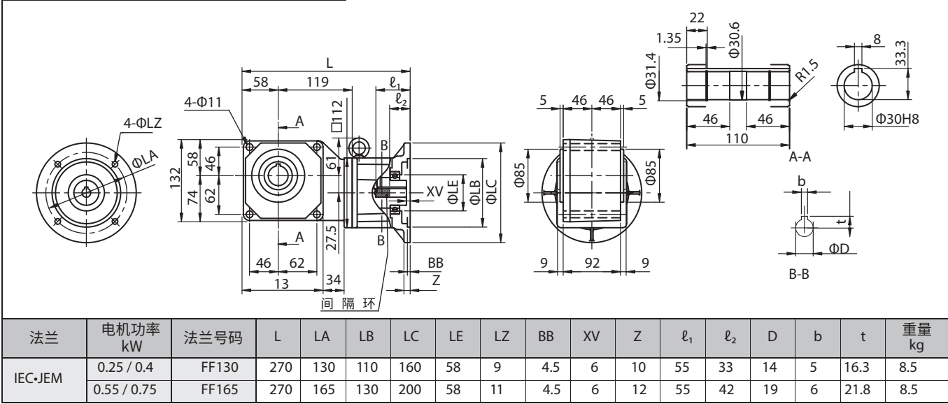
图 E408 RNYX - 1330 - [ 减速比 ]
