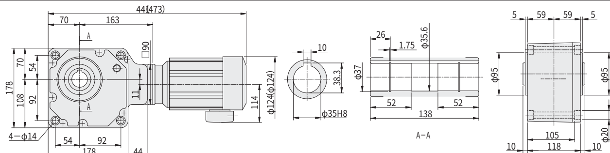
图 E115 RNYM02-1440-AV-720~1440 (RNYM02-1440-AV-B-720~1440) 重量 17kg (重量 18kg)
