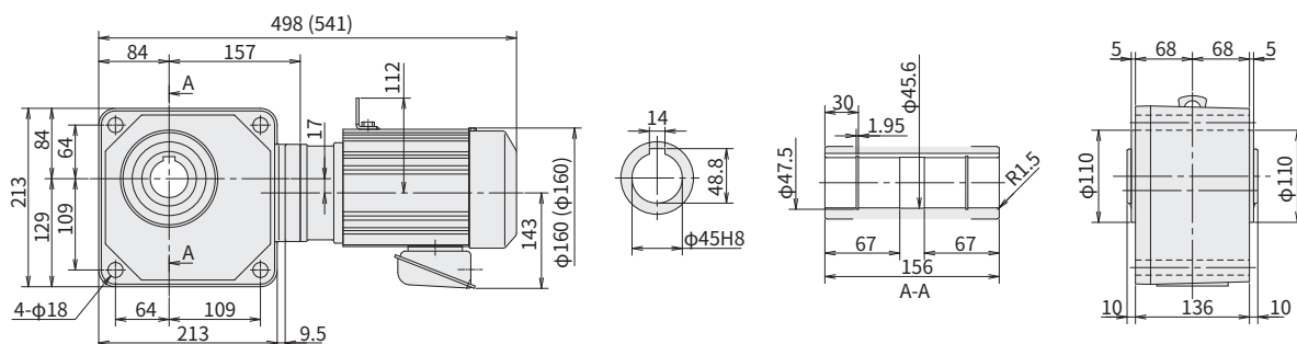
图 E52 RNYM1-1530-80~120 (RNYM1-1530-B-80~120) 重量 25kg (重量 28kg)
