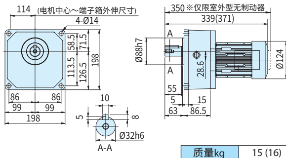
图C15 ZNFM05-1320-100~200 (ZNFM05-1320-B-100~200)
