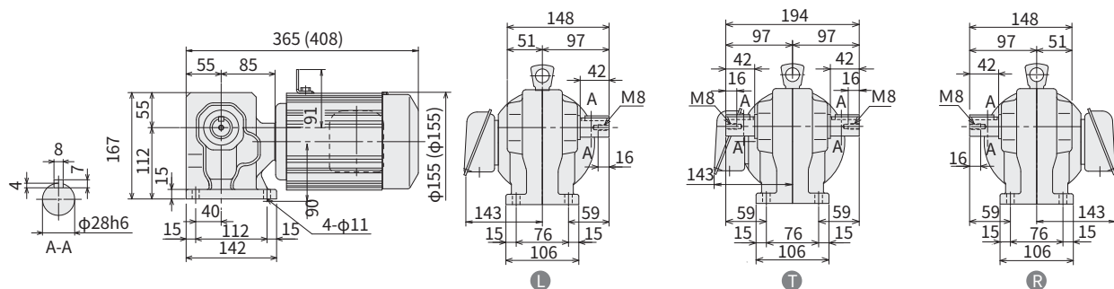
图 E369 RNHM1-370-B-5~30 重量 13.5kg (RNHM1-370-B-5~30) (重量 16.5kg)
