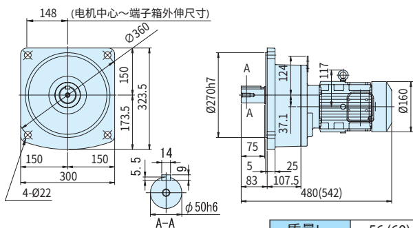
图C33 ZNFM2-1500-100~200 (ZNFM2-1500-B-100~200)
