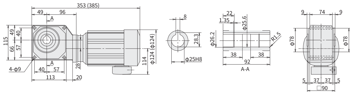
图 E109 RNYM02-1220-AV-20~60 (RNYM02-1220-AV-B-20~60) 重量 9.5kg (重量 11kg)
