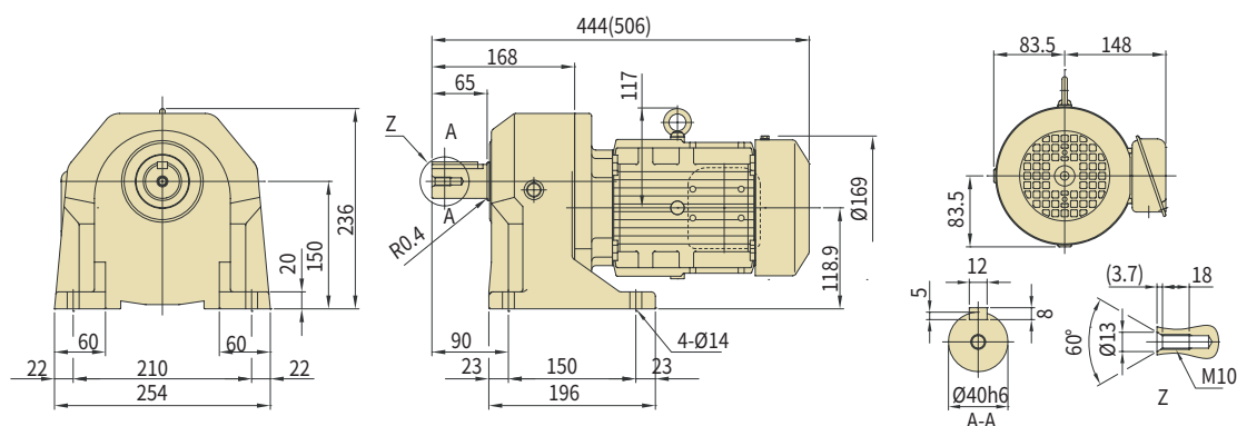
图 C91 ZNHM1-1400-AV-100~200 (ZNHM1-1400-AV-B-100~200)
