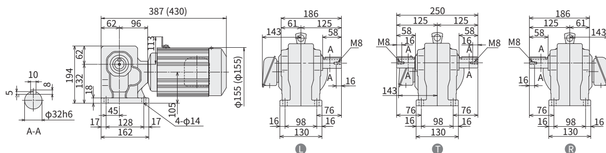
图 E401 RNHM05-43-AV-40~60 (RNHM05-43-AV-B-40~60) 重量 17kg (重量 20kg)
