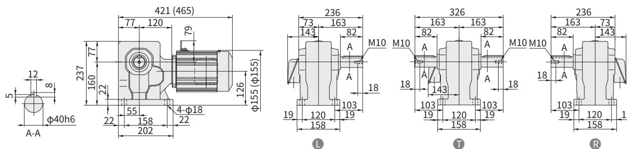
图 E402 RNHM05-50-AV-80~120 (RNHM05-50-AV-B-80~120) 重量 24kg (重量 27kg)
