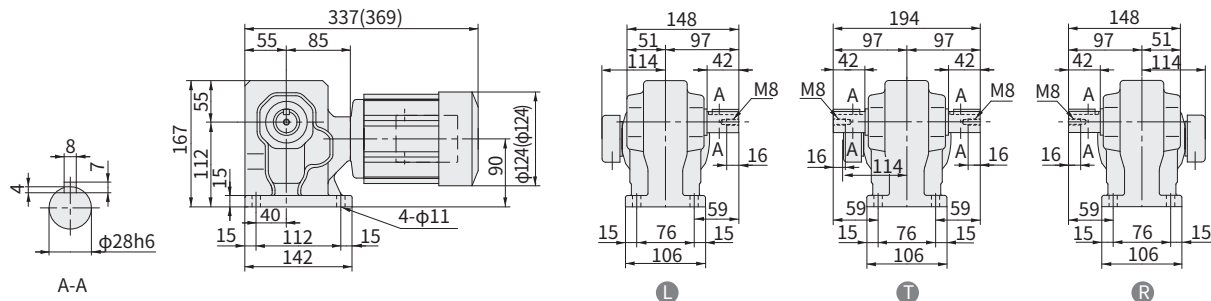
图 E411 RNHM02-33-EP-40~60 重量 11kg (RNHM02-33-EP-B-40~60) (重量 12kg)
