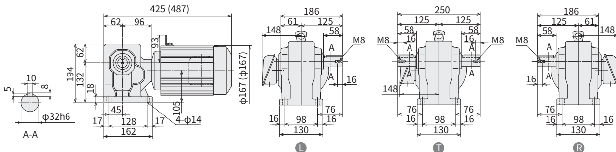
图 E376 RNHM2-470 1 -5~30 (RNHM2-470 1 -B-5~30) 重量 21.5kg (重量 26.5kg)
