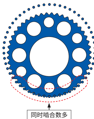
多齿差齿形
