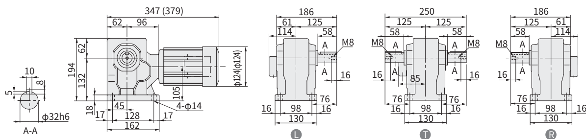
图 E357 RNHM03-40-J80~120 (RNHM03-40-J-B-80~120) 重量 14kg (重量 15kg)
