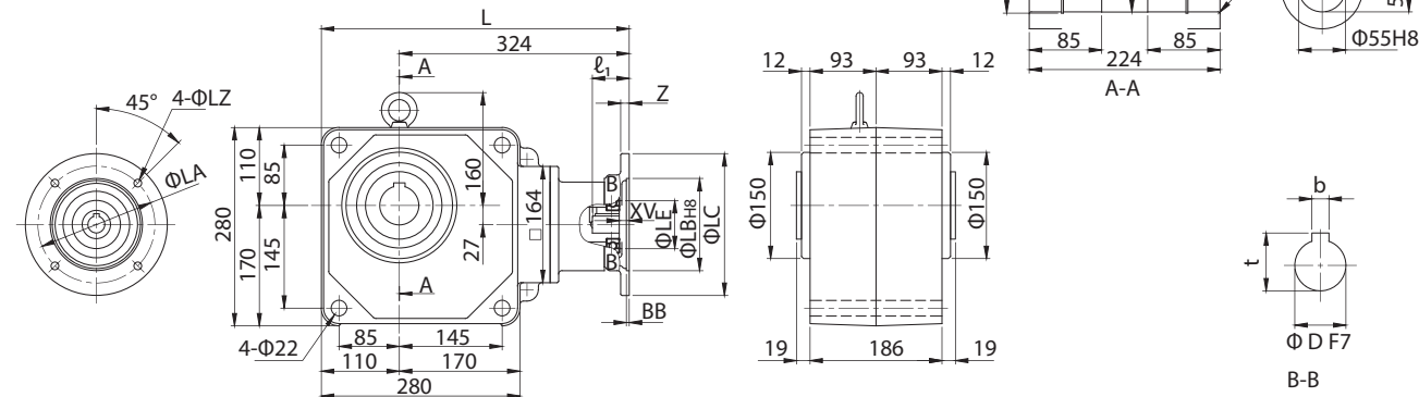
图 E416 RNYX - 1630 - [ 减速比 ]
