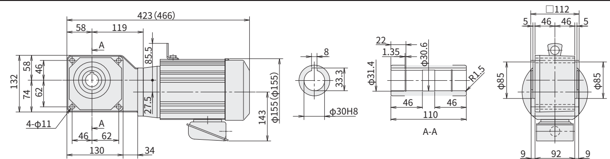
图 E118 RNYM05-1320-AV-5~30 (RNYM05-1320-AV-B-5~30) 重量 15kg (重量 17kg)
