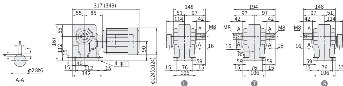
图 E350 RNHM02-35 h -150~240 (RNHM02-35 B -B-150~240) 重量 10kg (重量 11kg)
