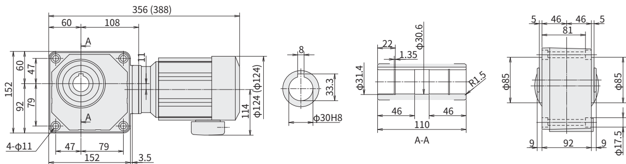
图 E22 RNYM02-1330-80~240 (RNYM02-1330-B-80~240)
