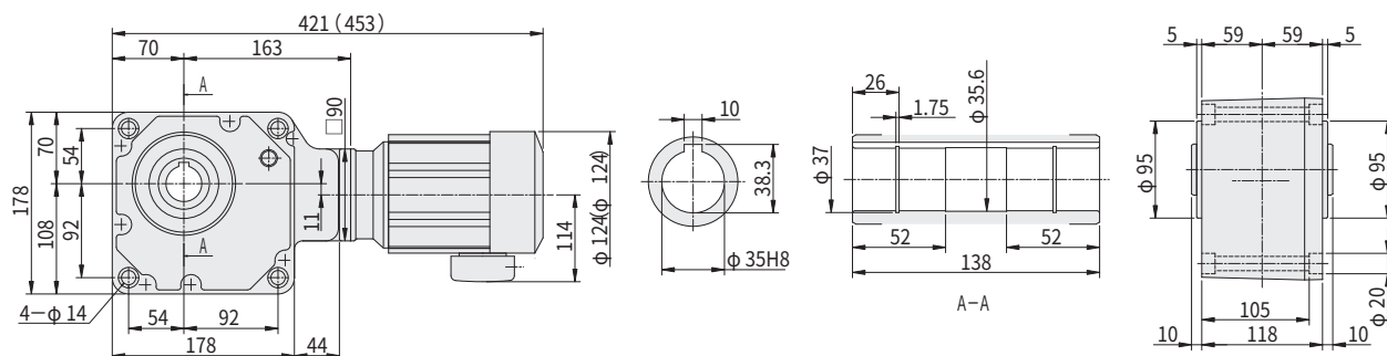
图 E104 RNYM01-1440-AV-720~1440 (RNYM01-1440-AV-B-720~1440) 重量 15.5kg (重量 17kg)
