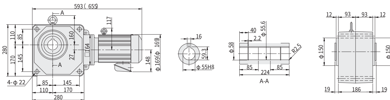
图 E126 RNYM1-1630-AV-100~120 重量 52kg (RNYM1-1630-AV-B-100~120) (重量 56kg)
