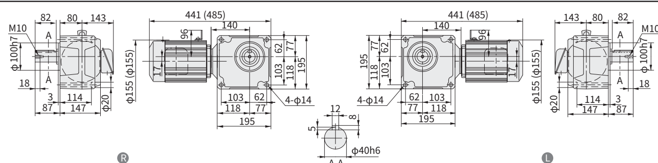
图 E259 RNFM1-50 R -80~120 重量 24kg (重量 27kg) • 安装本机器时请使用内六角螺钉 (M12)。
