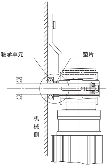
图 D4 用垫片固定 (从动轴无阶梯)
