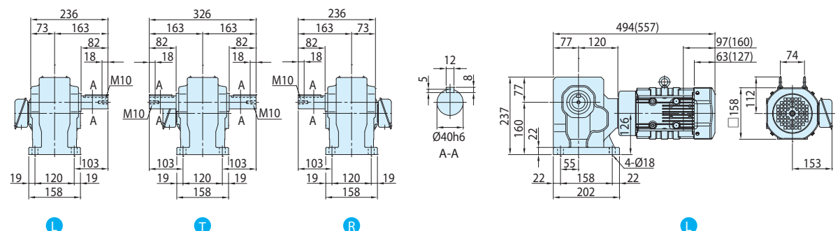
图E433 RNHM08-55 \frac{1}{2} -EP-150~240 (RNHM08-55 \frac{1}{2} -EP-B-150~240)
