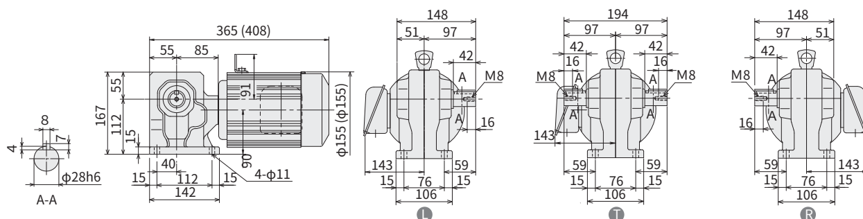
图 E365 RNHM08-370 h6 -5~30 (RNHM08-370 h6 -B-5~30) 重量 13.5kg (重量 16.5kg)
