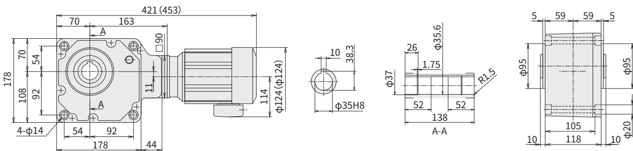
图 E24 RNYM02-1440-300~1440 (RNYM02-1440-B-300~1440)
