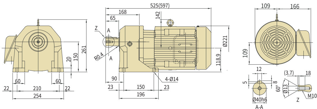
图 C102 ZNHM3-1501-AV-30~100 (ZNHM3-1501-AV-B-30~100)
