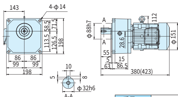
图C25 ZNFM1-1321-30~100 (ZNFM1-1321-B-30~100)
