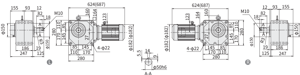
图 E300 RNFM2-1631 R -AVX1-150~240 重量 62kg • 安装本机器时请使用内六角螺钉 (M20)。 (RNFM2-1631 R -AVX1-B-150~240) (重量 68kg)
