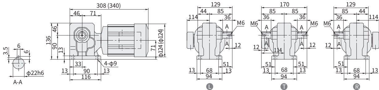
图 E410 RNHM02-270-EP-5~30 重量 8.5kg (RNHM02-270-EP-B-5~30) (重量 10kg)
