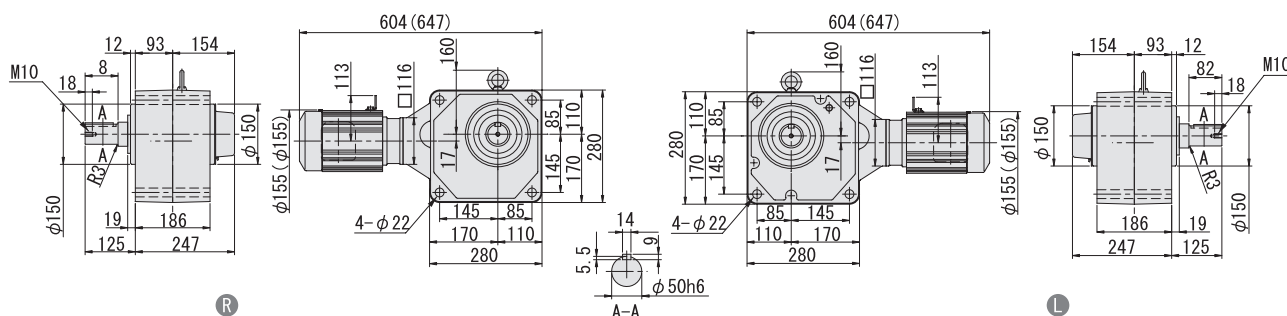
图 E256 RNFM08-1640 R -X1-300~1440 重量 72kg (重量 74kg) • 安装本机器时请使用内六角螺钉 (M20)。
