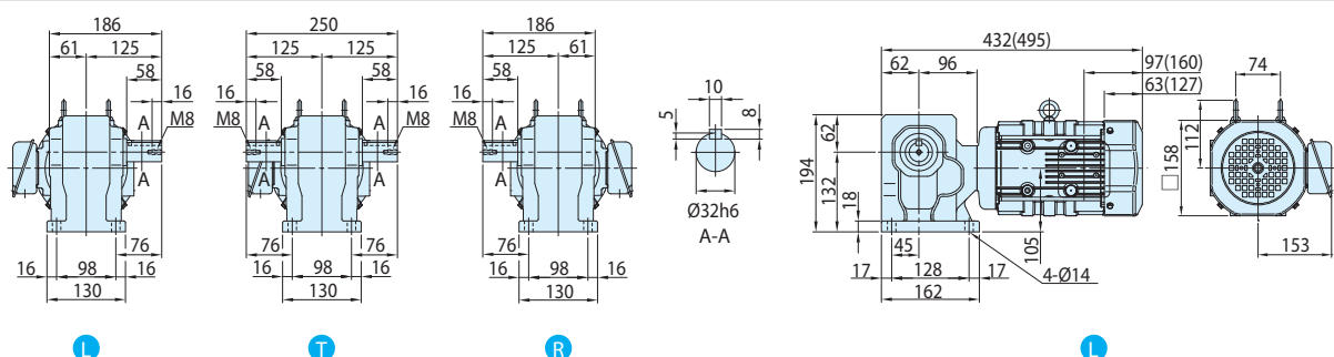
图E431 RNHM08-43 \frac{1}{2} -EP-40~60 (RNHM08-43 \frac{1}{2} -EP-B-40~60)
