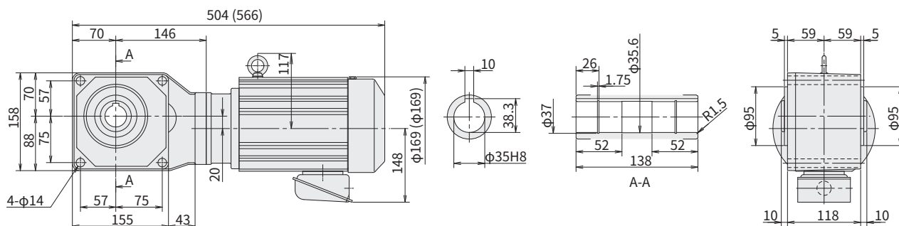
图 E123 RNYM1-1420-AV-5~30 重量 22kg (RNYM1-1420-AV-B-5~30) (重量 26kg)
