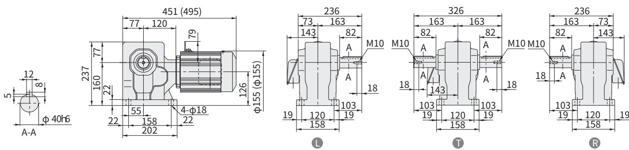
图 E368 RNHM08-55-B-150~240 重量 25kg (RNHM08-55-B-150~240) (重量 28kg)
