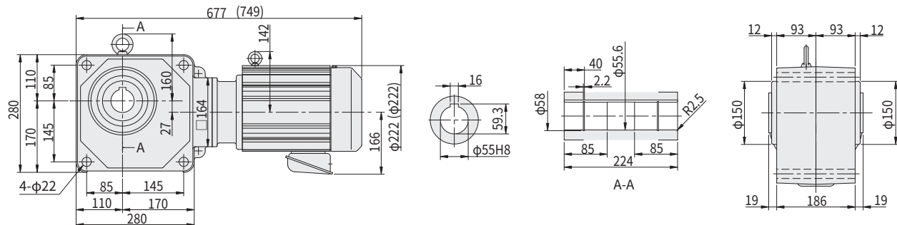
图 E134 RNYM3-1632-AV-30~60 (RNYM3-1632-AV-B-30~60)
