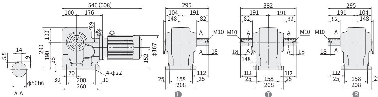
图 E375 RNHM1H-60 1 -100~120 (RNHM1H-60 1 -B-100~120) 重量 69kg (重量 73kg)
