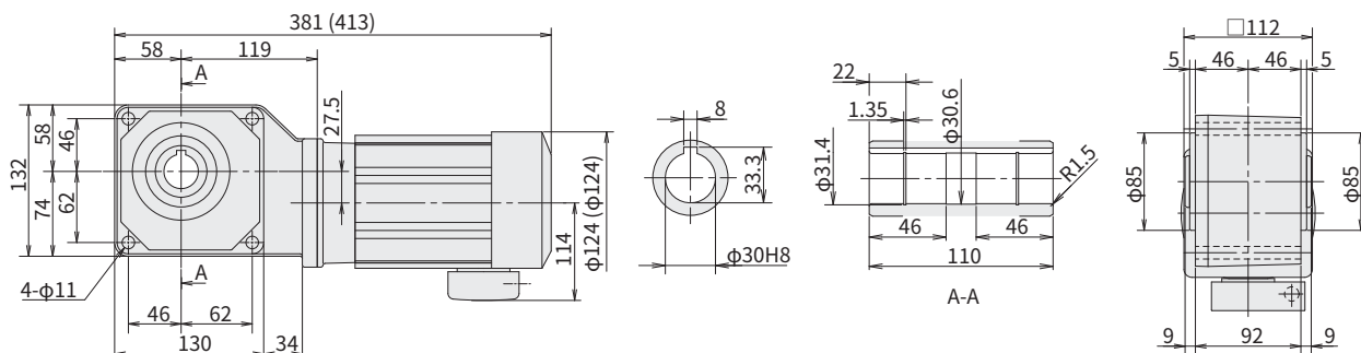
图 E33 RNYM05-1320-5~12 (RNYM05-1320-B-5~12)
