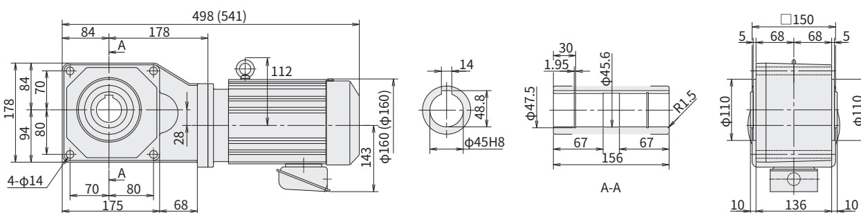
图 E51 RNYM1-1520-40~60 (RNYM1-1520-B-40~60) 重量 26kg (重量 28kg)
