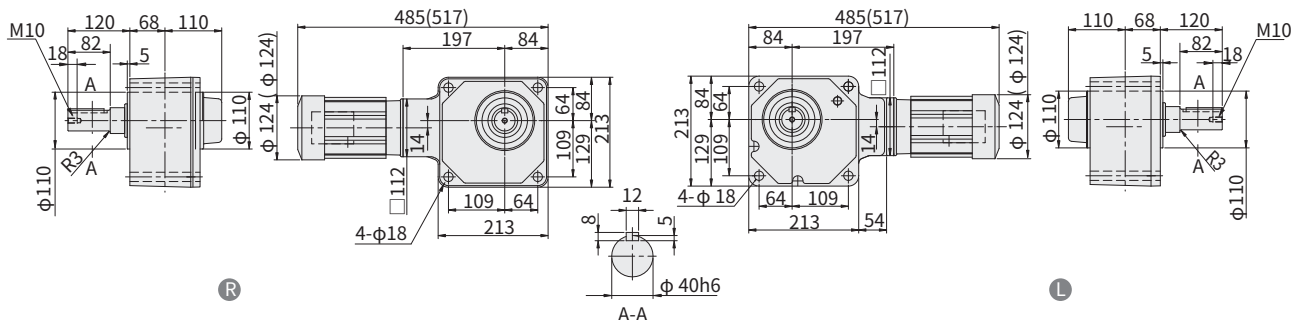
图 E250 RNFM05-1540 \frac{h}{B} -X1-600~1440 重量 29kg (重量 30kg) • 安装本机器时请使用内六角螺钉 (M16)。
