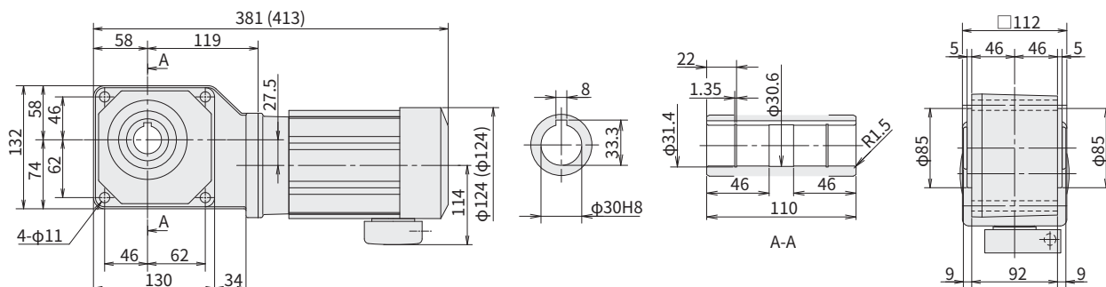
图 E35 RNYM05-1320-15~60 (RNYM05-1320-B-15~60)
