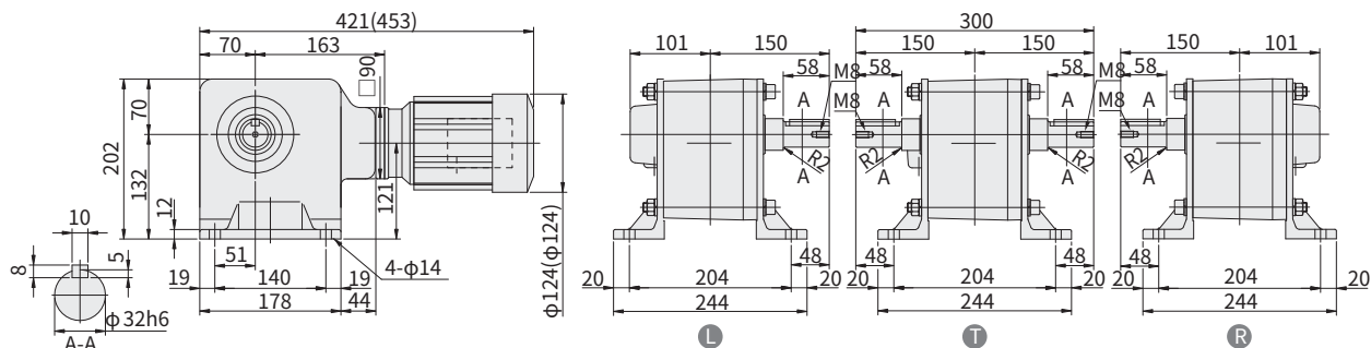
图 E351 RNHM02-1440-J1-300~480 (RNHM02-1440-J1-B-300~480) 重量 23kg (重量 24.5kg)
