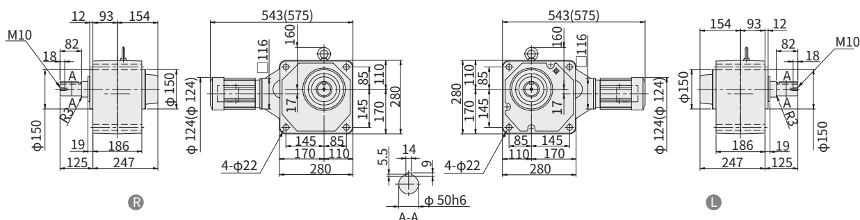
图 E249 RNFM05-1640 \frac{h}{B} -X1-300~480 重量 68kg (重量 69kg) • 安装本机器时请使用内六角螺钉 (M20)。
