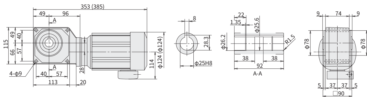
图 E141 RNYM02-1220-EP-5~15 (RNYM02-1220-EP-B-5~15)
