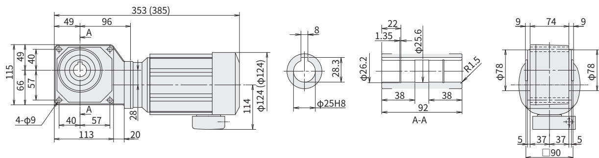
图 E143 RNYM02-1220-EP-20~60 重量 9.5kg (RNYM02-1220-EP-B-20~60) (重量 11kg)
