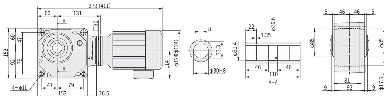
图 E103 RNYM01-1340-AV-720~1440 (RNYM01-1340-AV-B-720~1440) 重量 11kg (重量 12kg)
