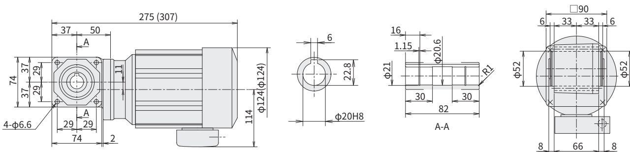
图 E16 RNYM02-1110-5~10 (RNYM02-1110-B-5~10) 重量 6.0kg (重量 7.5kg)
