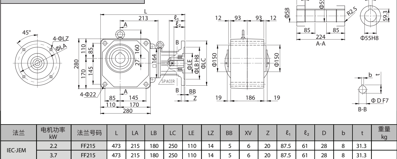
图 E420 RNYX - 1632 - [ 减速比 ]
