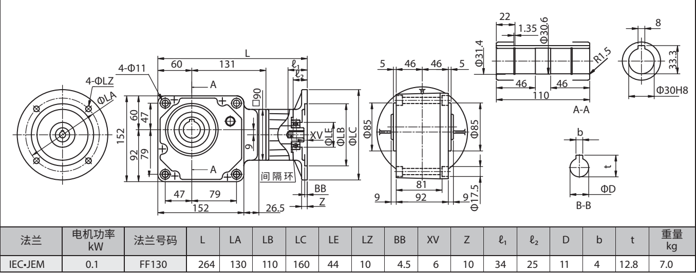
图 E409 RNYX - 1340 - [ 减速比 ]
