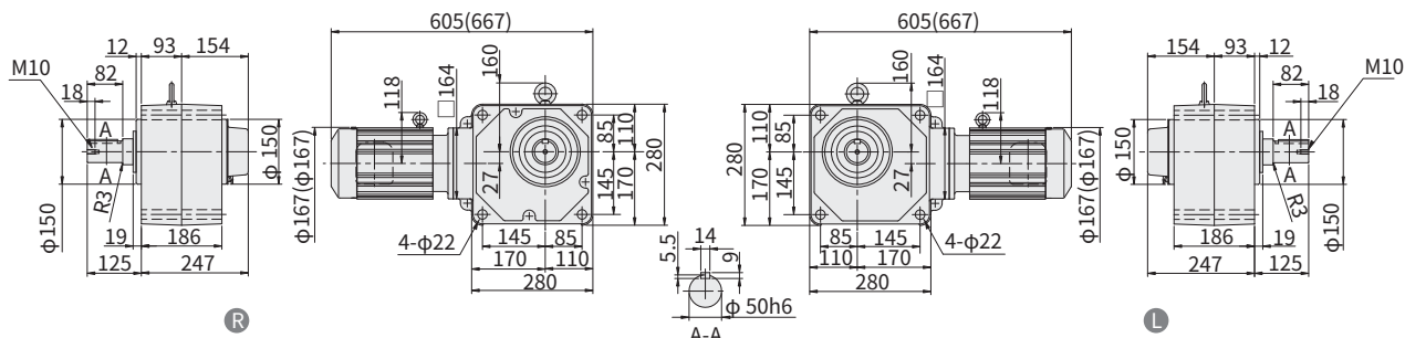
图 E297 RNFM1-1631 R -AVX1-150~240 重量 58kg • 安装本机器时请使用内六角螺钉 (M20)。 (RNFM1-1631 R -AVX1-B-150~240) (重量 62kg)
