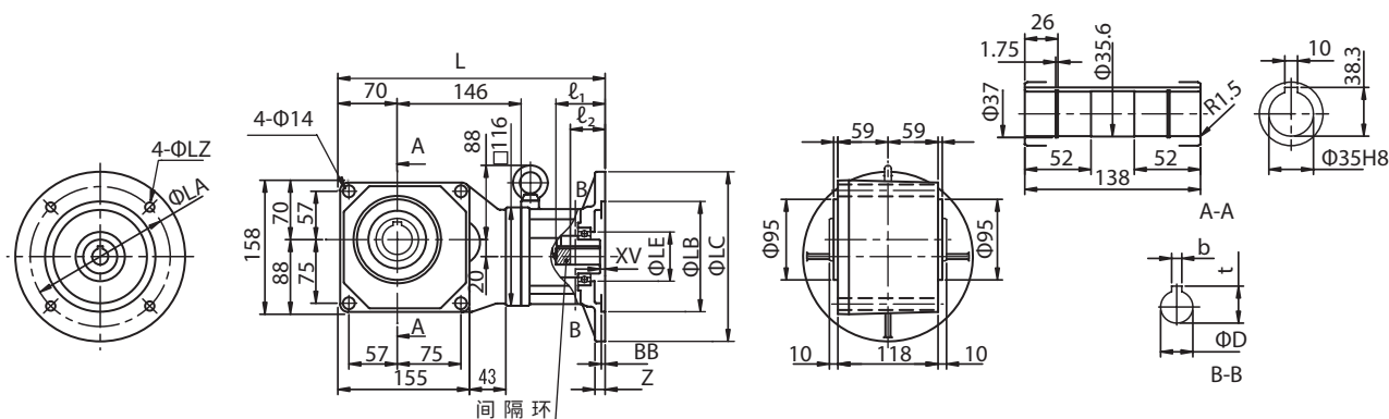
图 E410 RNYX - 1420 - [ 减速比 ]
