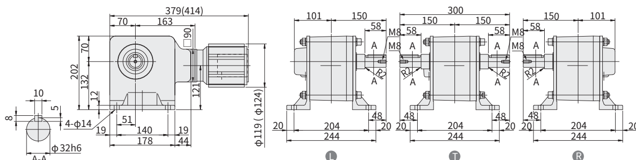
图 E346 RNHM01-1440-J1-300~1440 重量 22kg (RNHM01-1440-J1-B-300~1440) (重量 23.5kg)
