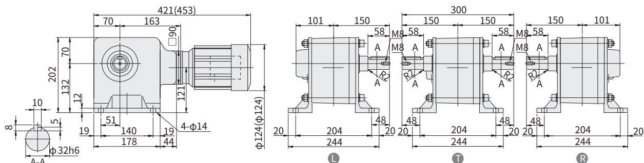
图 E353 RNHM02-1440-J1-600~1440 (RNHM02-1440-J1-B-600~1440) 重量 23kg (重量 24.5kg)
