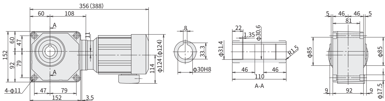
图 E100 RNYM01-1330-AV-80~240 (RNYM01-1330-AV-B-80~240) 重量 10kg (重量 11kg)
