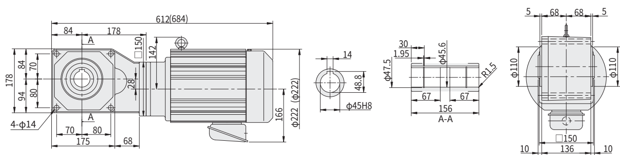
图 E88 RNYM5-1521-20~25 (RNYM5-1521-B-20~25) 重量 50kg (重量 61kg)
