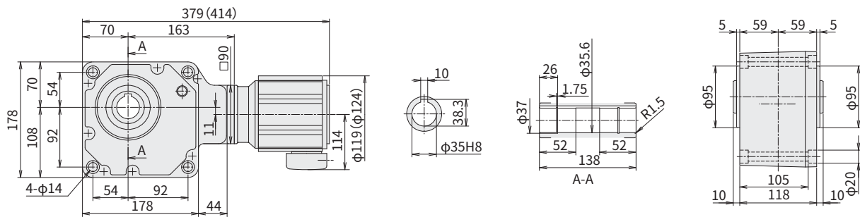
图 E15 RNYM01-1440-300~1440 (RNYM01-1440-B-300~1440) 重量 14.5kg (重量 16kg)
