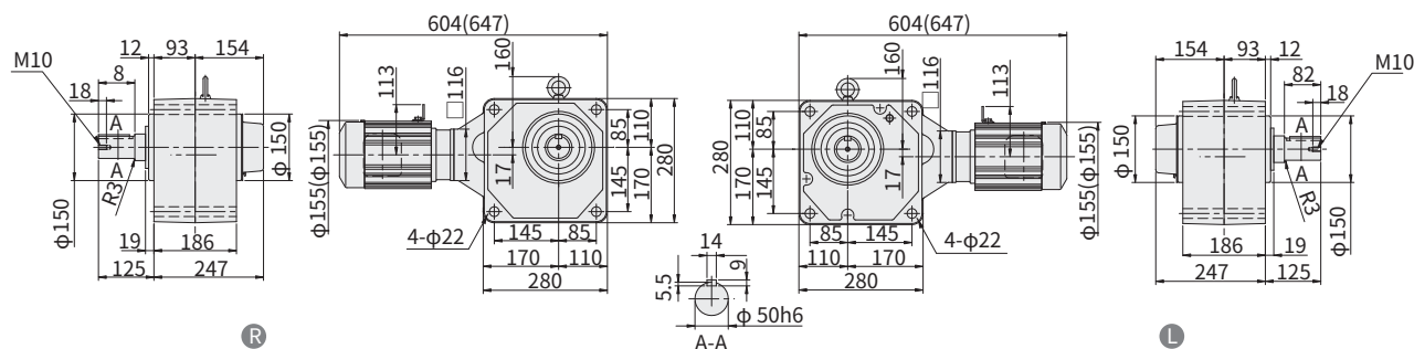
图 E321 RNF05-1640 II -EPX1-300~1440 重量 73kg (RNF05-1640 II -EPX1-B-300~1440) (重量 75kg)
