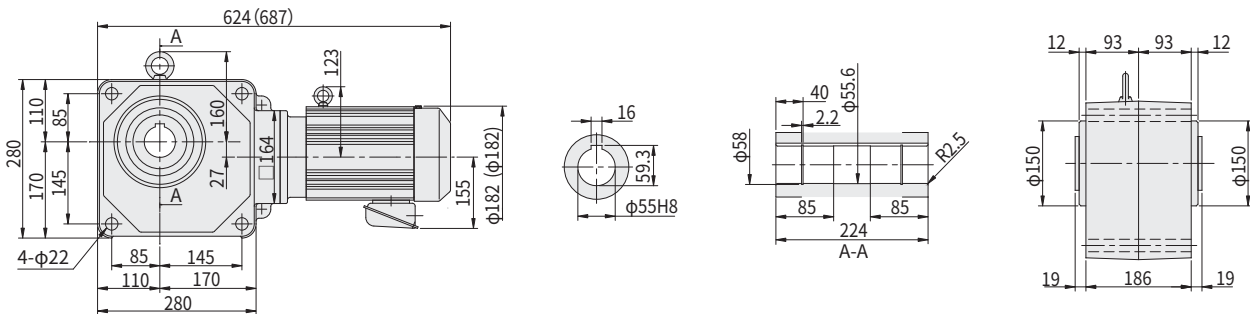
图 E79 RNYM3-1630-80~120 重量 57kg (RNYM3-1630-B-80~120) (重量 63kg)
