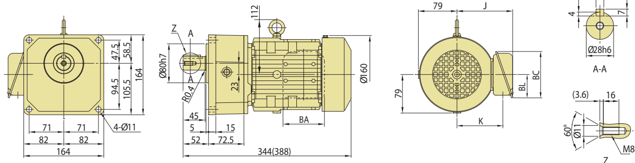
图 C21 ZNFM08-1321-30~100/ 规格代号 (ZNFM08-1321-B-30~100/ 规格代号)
