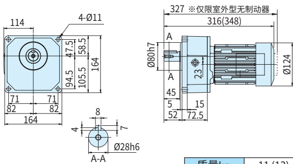
图C13 ZNFM05-1281-30~100 (ZNFM05-1281-B-30~100)
