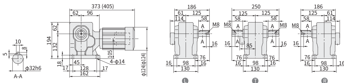
图 E363 RNHM05-45 h6 -150~240 (RNHM05-45 h6 -B-150~240) 重量 15kg (重量 16kg)
