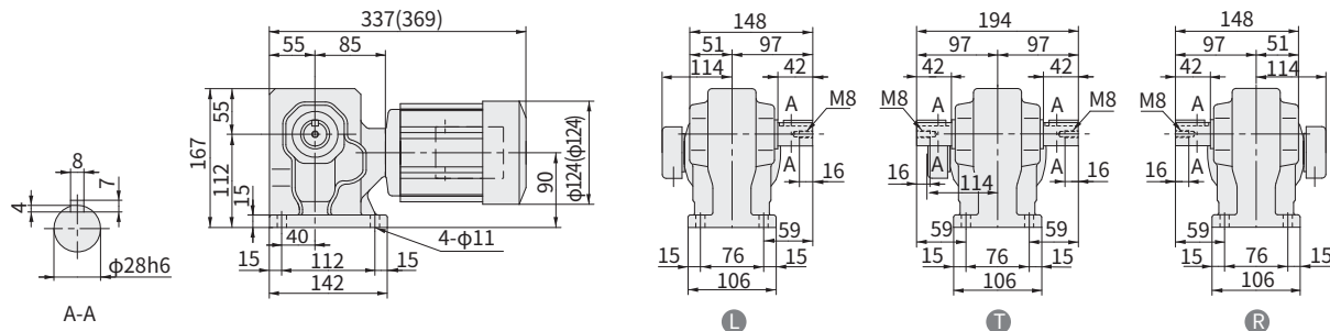
图 E419 RNHM03-33-EP-40~60 重量 11kg (RNHM03-33-EP-B-40~60) (重量 12kg)
