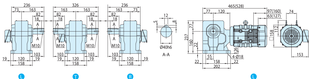
图E432 RNHM08-50 \frac{1}{2} -EP-80~120 (RNHM08-50 \frac{1}{2} -EP-B-80~120)
