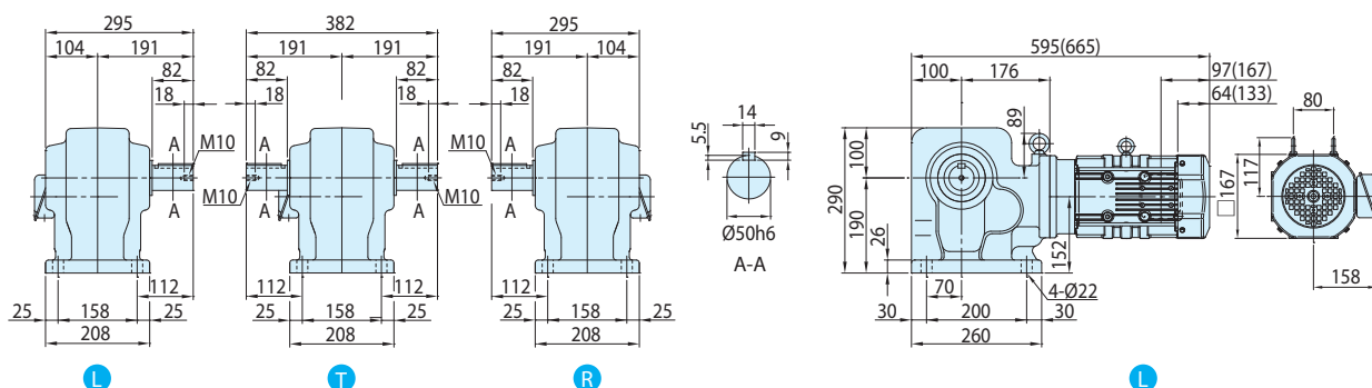
图E444 RNHM3-54 \frac{1}{2} -EP-10~60 (RNHM3-54 \frac{1}{2} -EP-B-10~60)
