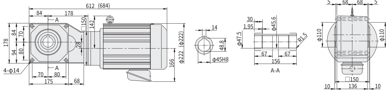
图 E133 RNYM3-1521-AV-5~25 (RNYM3-1521-AV-B-5~25)
