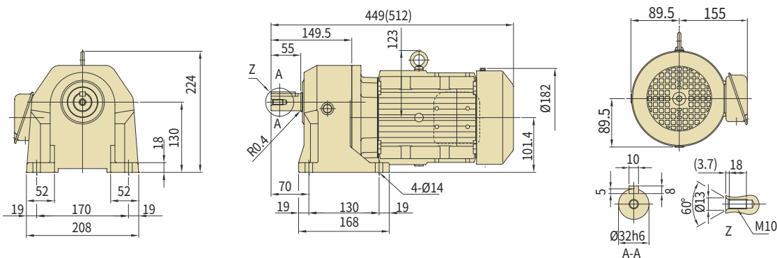
图 C95 ZNHM2-1320-AV-3~30 (ZNHM2-1320-AV-B-3~30)
