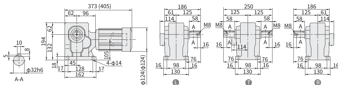
图 E395 RNHM02-45-AV-150~240 (RNHM02-45-AV-B-150~240) 重量 15kg (重量 16kg)
