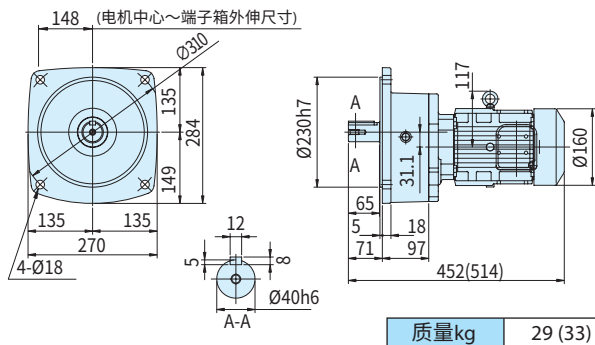
图C31 ZNFM2-1401-30~100 (ZNFM2-1401-B-30~100)
