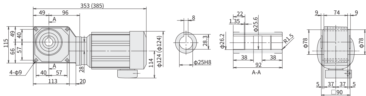
图 E107 RNYM02-1220-AV-5~15 (RNYM02-1220-AV-B-5~15) 重量 9.5kg (重量 11kg)
