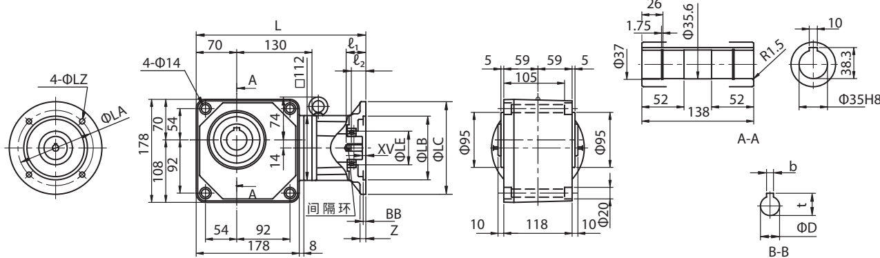
图 E411 RNYX - 1430 - [ 减速比 ]
