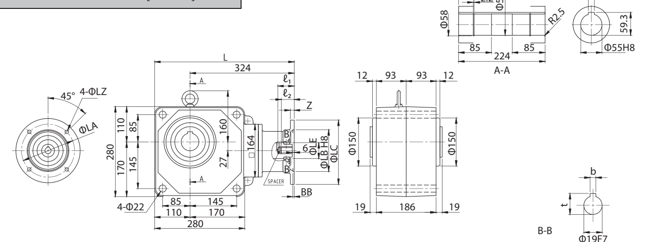
图 E418 RNYX - 1631 - [ 减速比 ]
