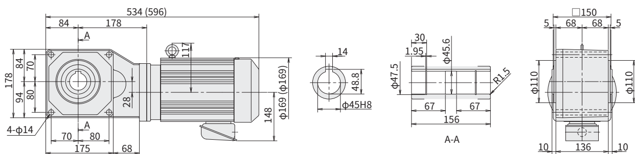
图 E124 RNYM1-1520-AV-40~60 (RNYM1-1520-AV-B-40~60) 重量 31kg (重量 35kg)
