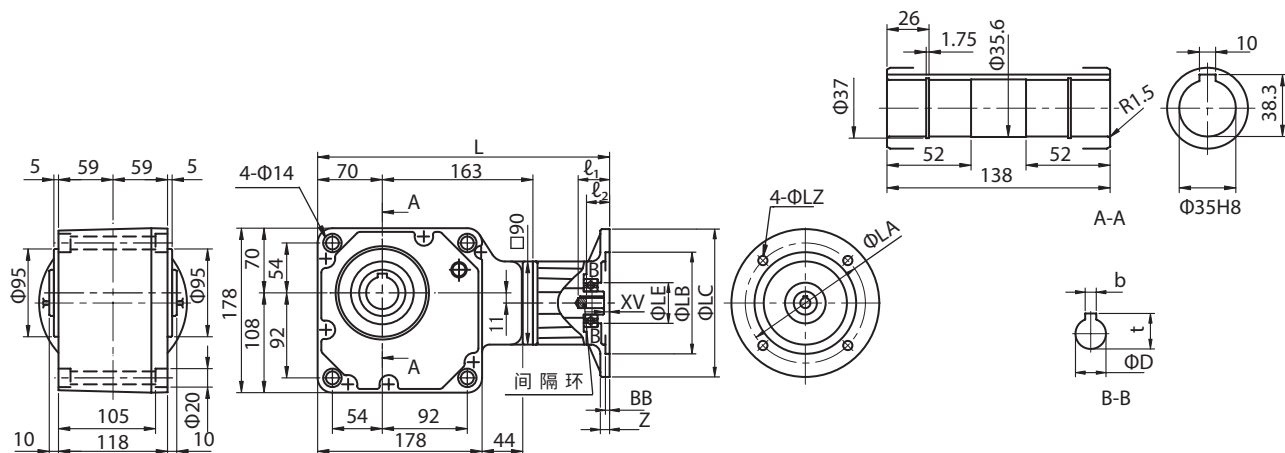
图 E412 RNYX - 1440 - [ 减速比 ]
