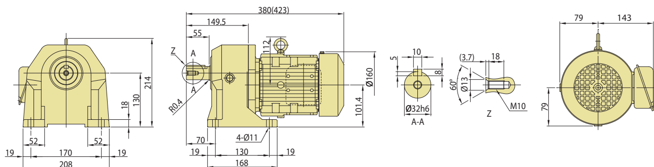
图 C47 ZNHM05-1320-EP-100~200 (ZNHM05-1320-EP-B-100~200)
