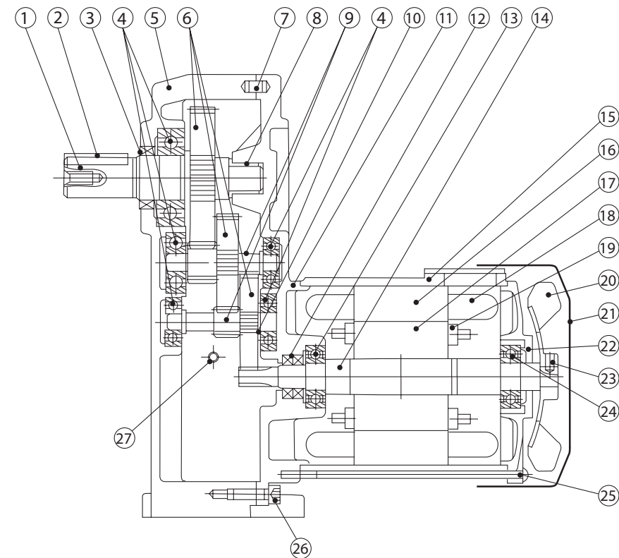
图DG2 地脚安装·齿轮电机结构图例
