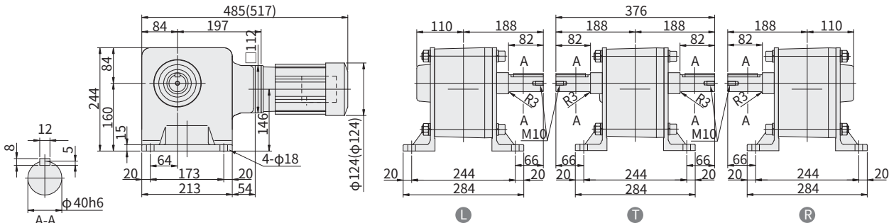
图 E359 RNHM03-1540 h -J1-300~1440 重量 41kg (RNHM03-1540 B -J1-B-300~1440) (重量 42kg)
