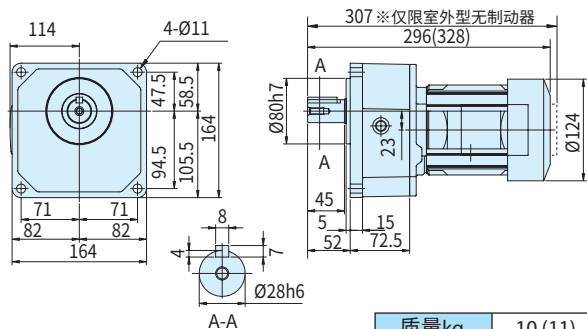
图C9 ZNFM02-1280-100~200 (ZNFM02-1280-B-100~200)
