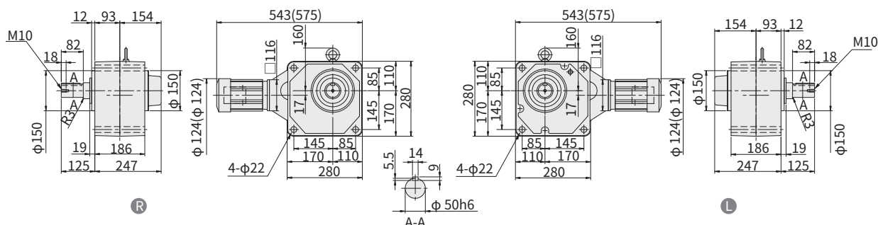
图 E251 RNFM05-1640 \frac{h}{B} -X1-600~1440 重量 68kg (重量 69kg) • 安装本机器时请使用内六角螺钉 (M20)。
