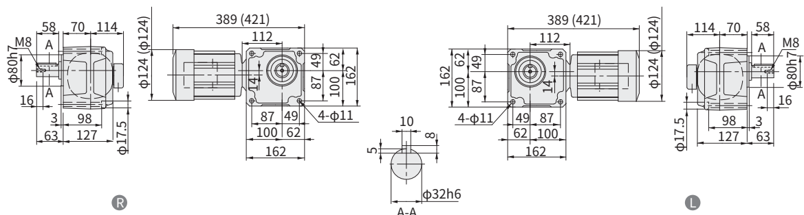
图 E247 RNF05-45 R -150~240 重量 15kg (RNF05-45 L -B-150~240) (重量 16kg)
