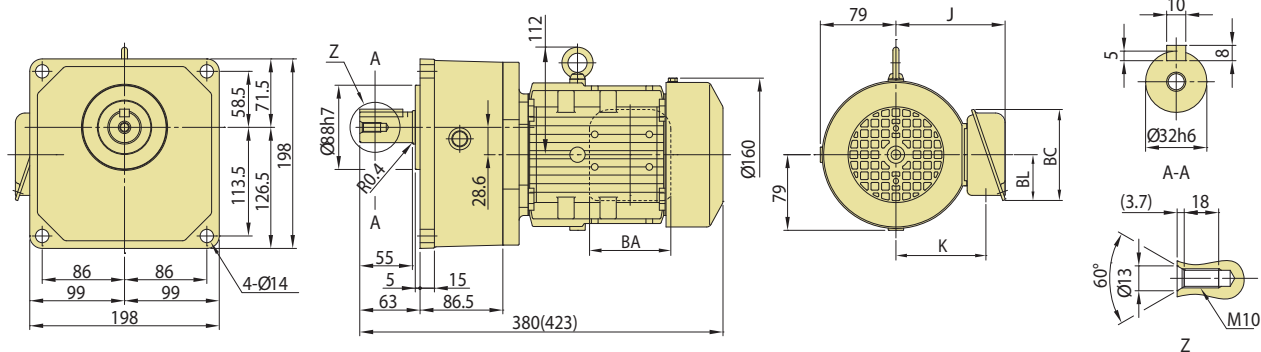
图 C22 ZNFM08-1400-100~200/ 规格代号 (ZNFM08-1400-B-100~200/ 规格代号)
