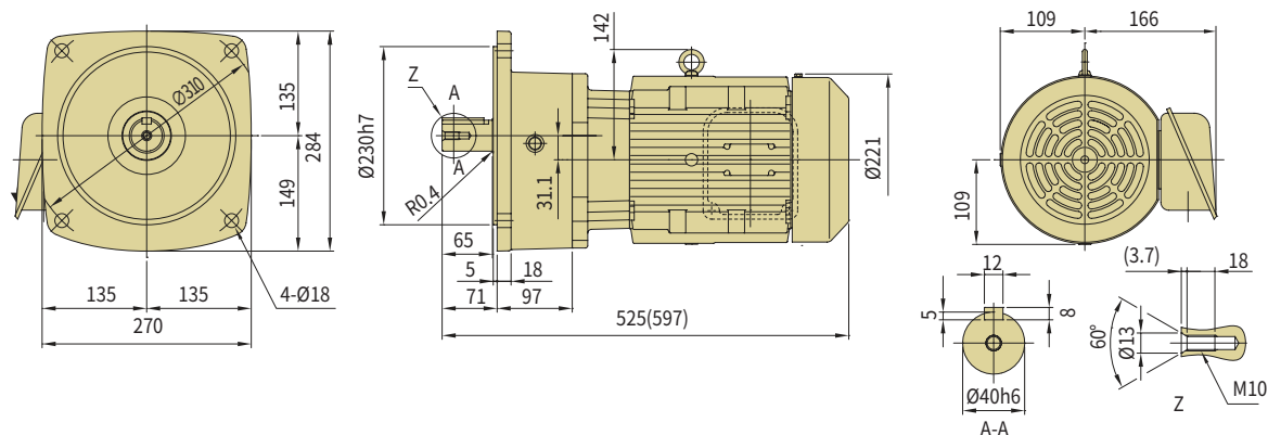
图 C104 ZNFM3-1501-AV-30~100 (ZNFM3-1501-AV-B-30~100)
