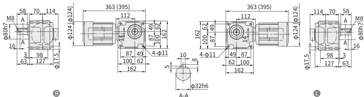
图 E311 RNFM03-40 L R -EP-80~120 重量 14kg (RNFM03-40 L R -EP-B-80~120) (重量 16kg) • 安装本机器时请使用内六角螺钉 (M10)。
