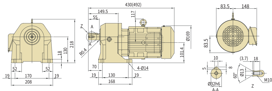
图 C90 ZNHM1-1321-AV-30~100 (ZNHM1-1321-AV-B-30~100)
