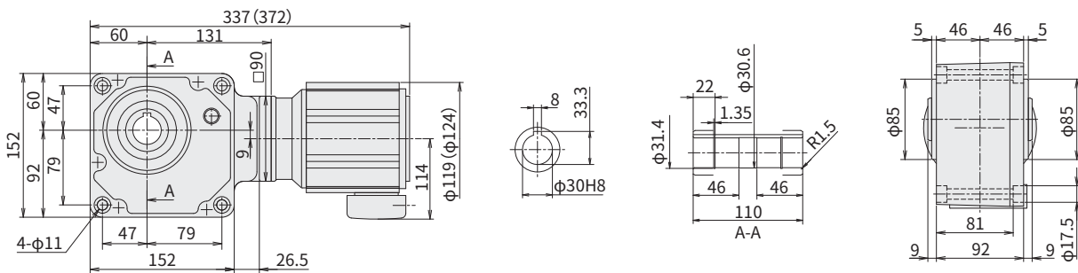
图 E14 RNYM01-1340-300~1440 (RNYM01-1340-B-300~1440) 重量 10kg (重量 11kg)
