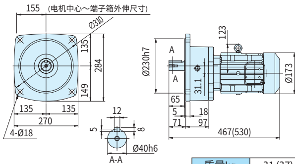
图C35 ZNFM3-1400-3~30 (ZNFM3-1400-B-3~30)
