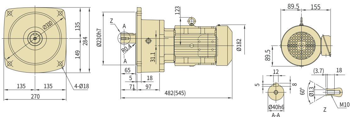
图 C99 ZNFM2-1401-AV-30~100 (ZNFM2-1401-AV-B-30~100)
