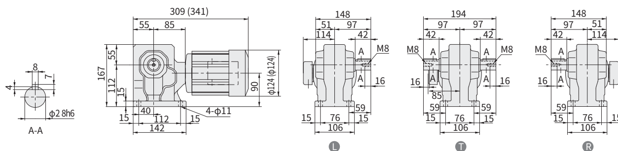
图 E349 RNHM02-30-B-80~120 重量 9.5kg (RNHM02-30-B-80~120) (重量 11kg)
