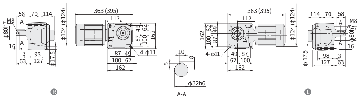
图 E246 RNF M05-40 R-80~120 重量 14kg (RNF M05-40 B-80~120) (重量 16kg) • 安装本机器时请使用内六角螺钉 (M10)。
