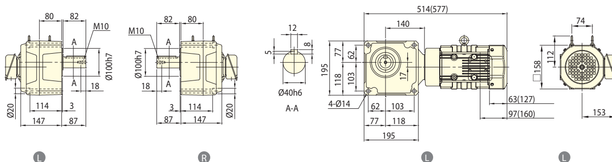
图 E325 RNFM08-55 k -EP-150~240 (RNFM08-55 k -EP-B-150~240)
