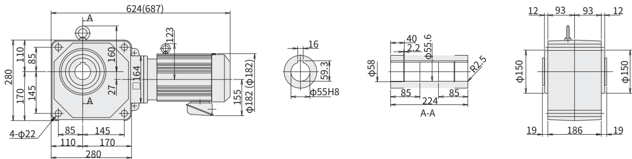
图 E77 RNYM3-1632-30~60 重量 55kg (RNYM3-1632-B-30~60) (重量 61kg)
