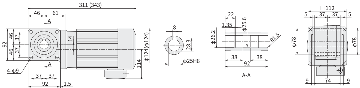
图 E31 RNYM05-1210-5~10 (RNYM05-1210-B-5~10) 重量 9kg (重量 10kg)
