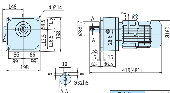
图C29 ZNFM2-1320-3~30 (ZNFM2-1320-B-3~30)
