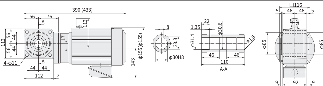
图 E117 RNYM05-1310-AV-5~10 (RNYM05-1310-AV-B-5~10) 重量 13kg (重量 16kg)
