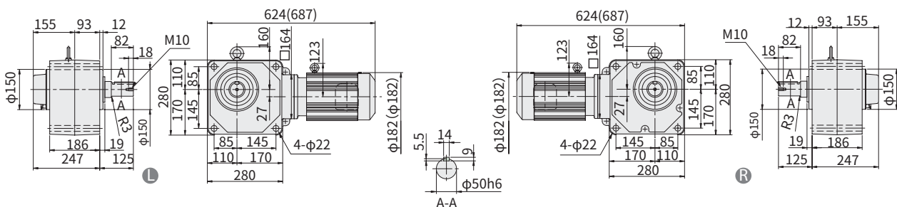
图 E299 RNFM2-1630 R -AVX1-80~120 重量 62kg • 安装本机器时请使用内六角螺钉 (M20)。 (RNFM2-1630 R -AVX1-B-80~120) (重量 68kg)
