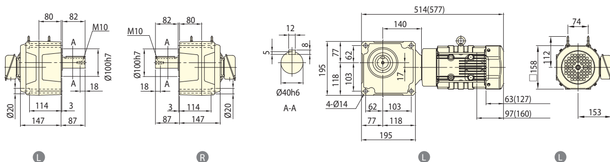
图 E329 RNFM1-55 L R -EP-150~240 (RNFM1-55 L R -EP-B-150~240)
