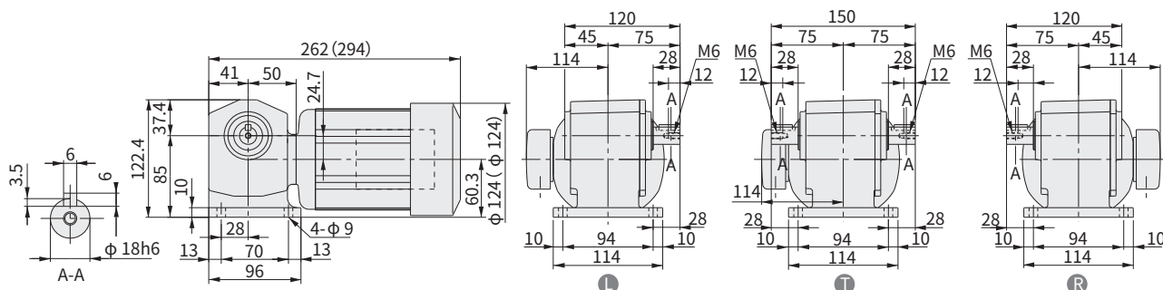
图 E384 RNHM01-190-AV-5~30 (RNHM01-190-AV-B-5~30) 重量 5.5kg (重量 7.0kg)
