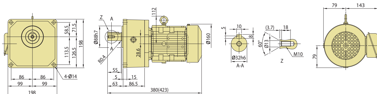
图 C50 ZNFM05-1320-EP-100~200 (ZNFM05-1320-EP-B-100~200)
