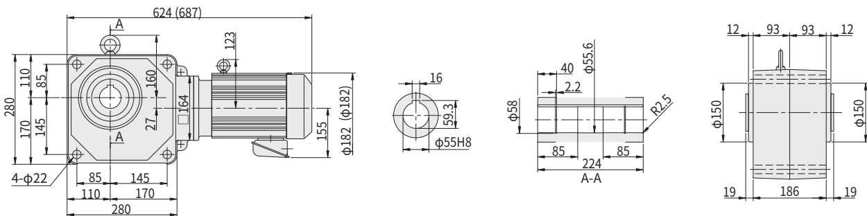
图 E80 RNYM3-1631-150~240 重量 57kg (RNYM3-1631-B-150~240) (重量 63kg)
