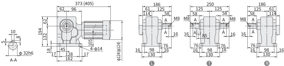
图 E358 RNHM03-45 h -150~240 重量 15kg (RNHM03-45 B -B-150~240) (重量 16kg)
