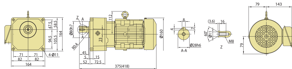
图 C49 ZNFM05-1281-EP-30~100 (ZNFM05-1281-EP-B-30~100)
