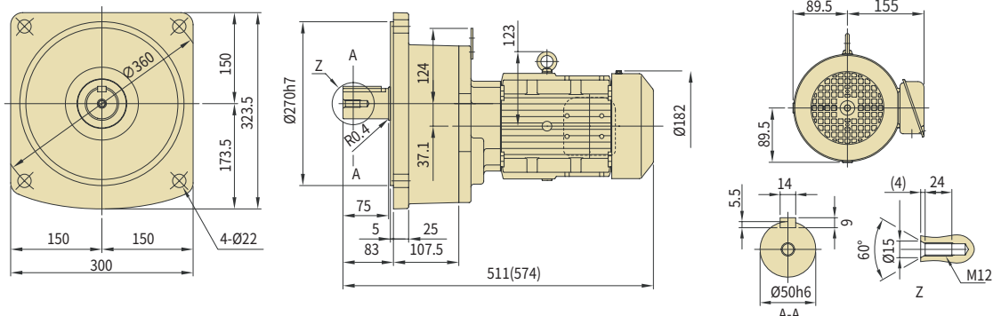
图 C101 ZNHM3-1400-AV-3~30 (ZNHM3-1400-AV-B-3~30)
