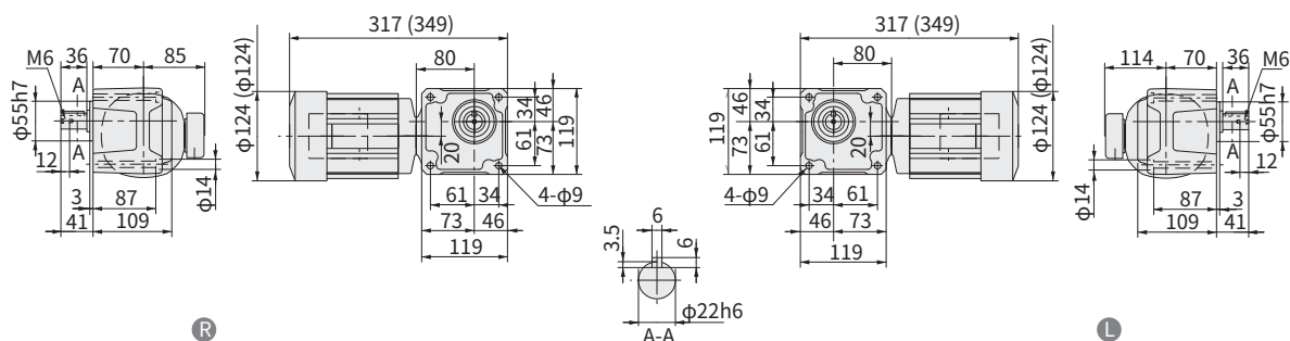
图 E244 RNF05-270 L R -5~30 重量 9.0kg • 安装本机器时请使用内六角螺钉 (M8)。 (RNF05-270 L R -B-5~30) (重量 10.5kg)
