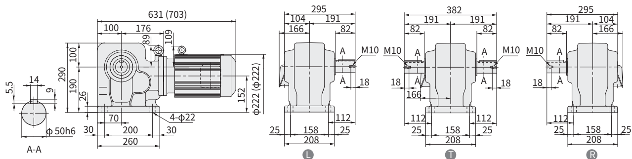
图 E382 RNHM5-63 L -10~50 重量 85kg (RNHM5-63 R -B-10~50) (重量 94kg)
