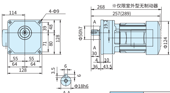
图C5 ZNFM02-1180-3~30 (ZNFM02-1180-B-3~30)
