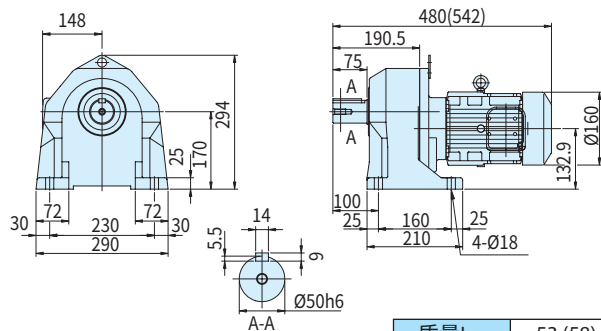
图C34 ZNHM2-1500-100~200 (ZNHM2-1500-B-100~200)
