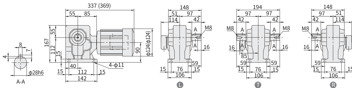
图 E356 RNHM03-33-J40~60 (RNHM03-33-J-B-40~60) 重量 11kg (重量 12kg)
