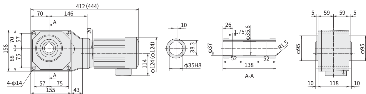
图 E36 RNYM05-1420-40~60 (RNYM05-1420-B-40~60)
