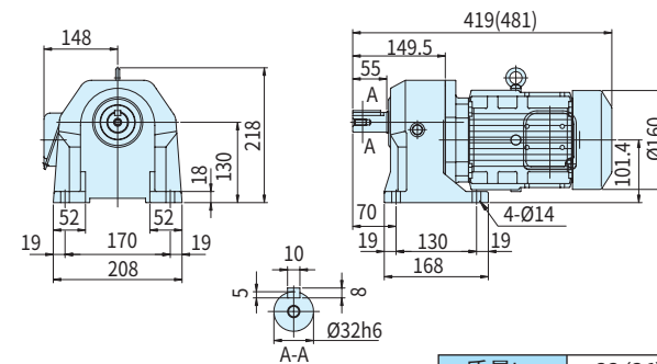
图C30 ZNFM2-1320-3~30 (ZNFM2-1320-B-3~30)
