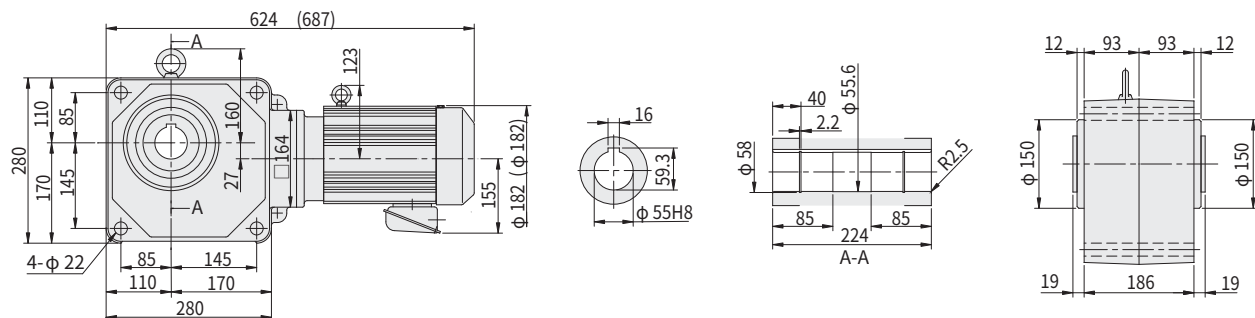
图 E131 RNYM2-1630-AV-80~120 (RNYM2-1630-AV-B-80~120)
