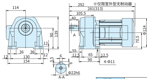
图C8 ZNHM02-1221-30~100 (ZNHM02-1221-B-30~100)
