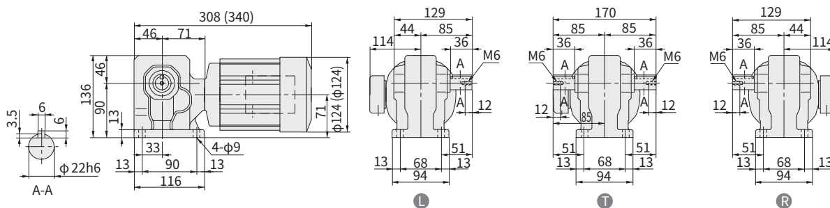
图 E355 RNHM03-270-J5~30 (RNHM03-270-J5-B~30) 重量 8.5kg (重量 10kg)
