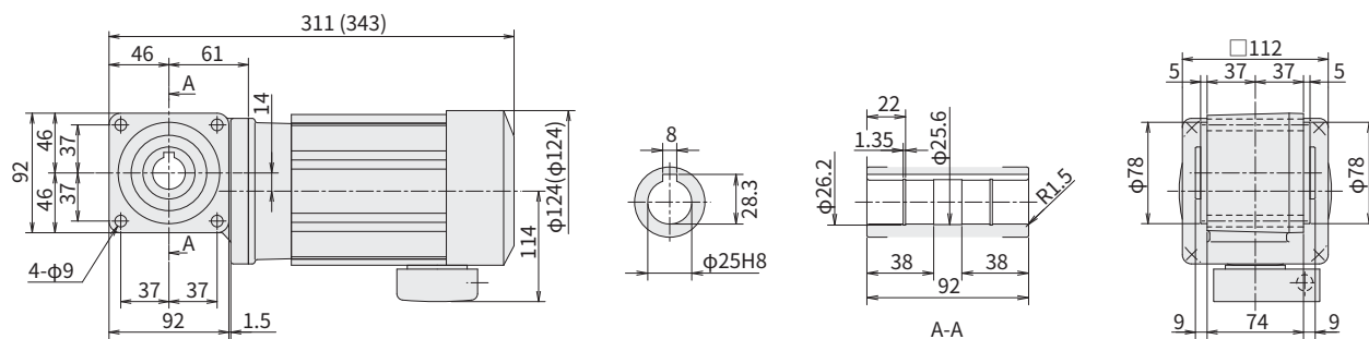
图 E139 RNYM02-1210-EP-5~10 (RNYM02-1210-EP-B-5~10)
