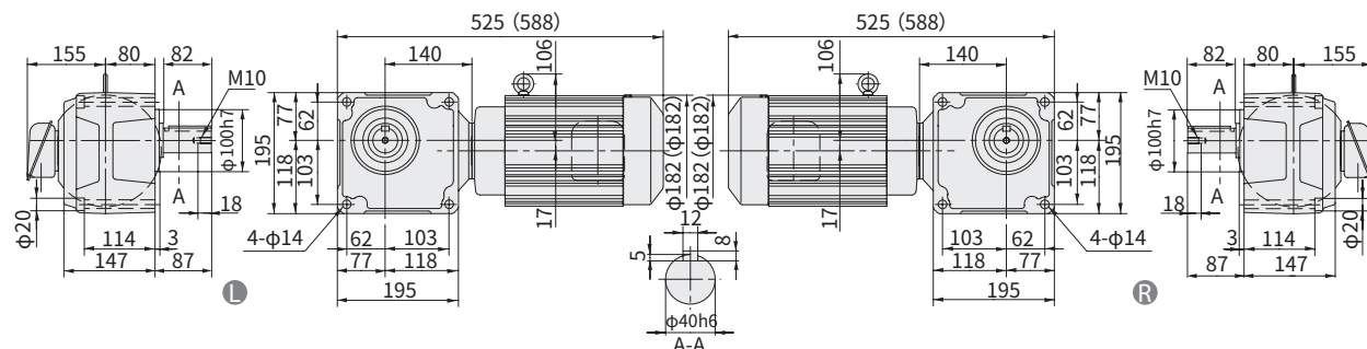
图 E298 RNFM2-54 R -AV-10~60 重量 34kg • 安装本机器时请使用内六角螺钉 (M12)。 (RNFM2-54 R -AV-B-10~60) (重量 40kg) • 请注意电机是否与安装面干涉。
