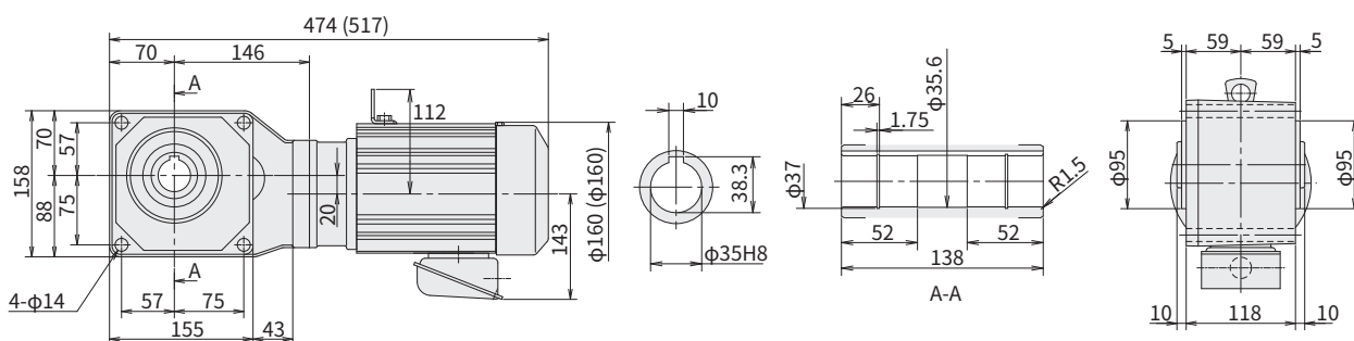
图 E50 RNYM1-1420-15~60 (RNYM1-1420-B-15~60) 重量 18kg (重量 20kg)
