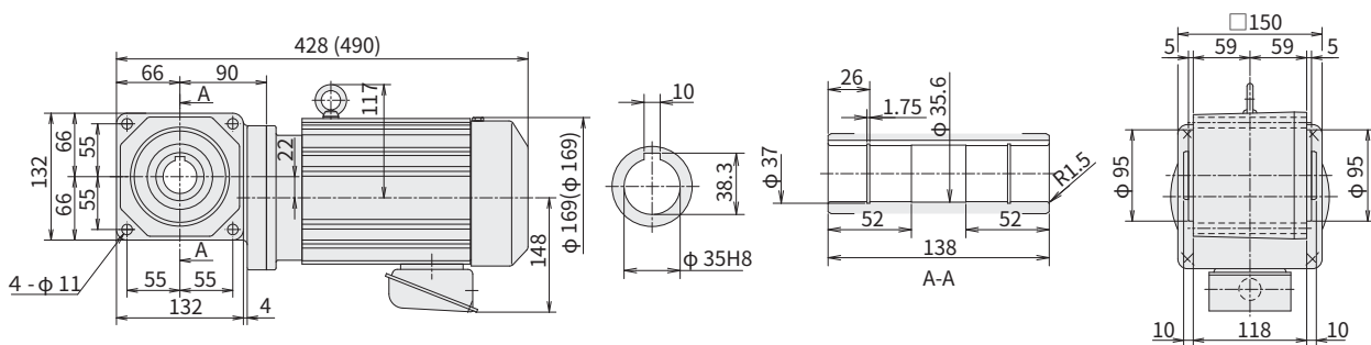
图 E64 RNYM2-1410-5~10 (RNYM2-1410-B-5~10) 重量 22kg (重量 26kg)
