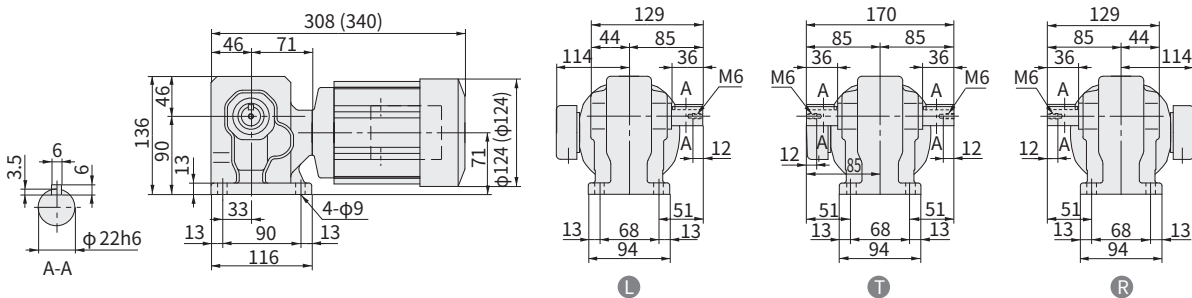
图 E360 RNHM05-270 h -5~30 重量 8.5kg (RNHM05-270 B -B-5~30) (重量 10kg)
