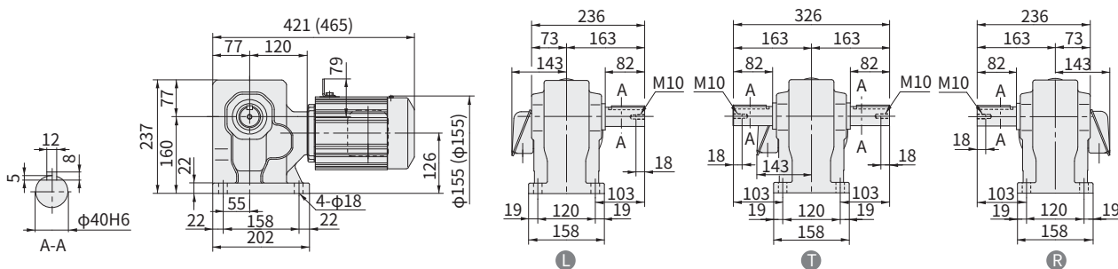
图 E367 RNHM08-50-B-80~120 重量 24kg (RNHM08-50-B-80~120) (重量 27kg)
