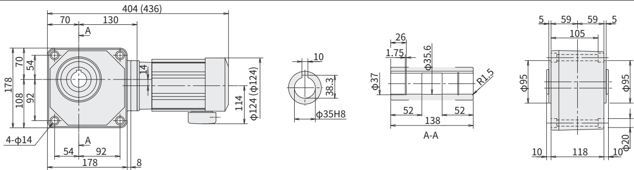
图 E29 RNYM03-1430-80~240 (RNYM03-1430-B-80~240) 重量 16kg (重量 17kg)
