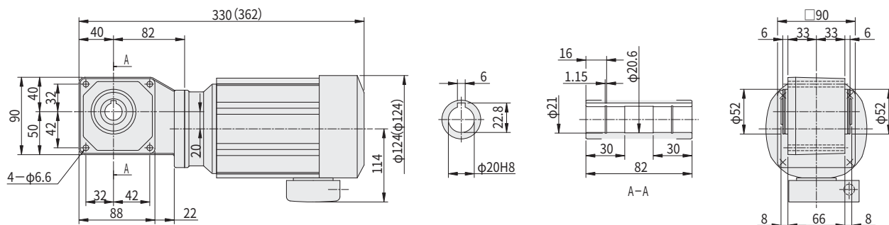
图 E106 RNYM02-1120-AV-5~15 (RNYM02-1120-AV-B-5~15) 重量 8.0kg (重量 9.0kg)
