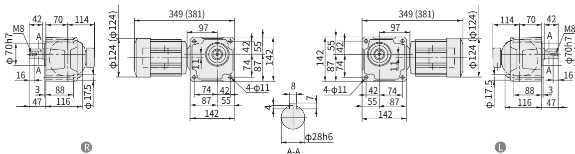
图 E310 RNFM03-33 L R -EP-40~60 重量 11kg (RNFM03-33 L R -EP-B-40~60) (重量 13kg) • 安装本机器时请使用内六角螺钉 (M10)。
