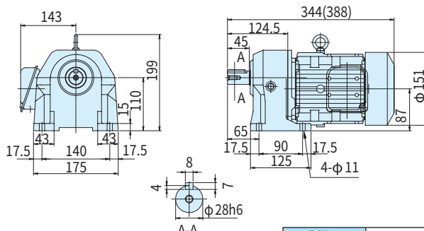
图C24 ZNFM1-1280-3~30 (ZNFM1-1280-B-3~30)
