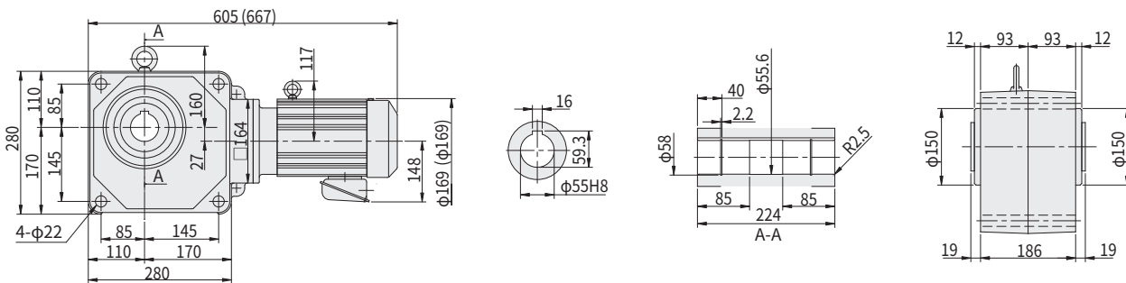
图 E63 RNYM1H-1631-150~240 (RNYM1H-1631-B-150~240) 重量 53kg (重量 57kg)
