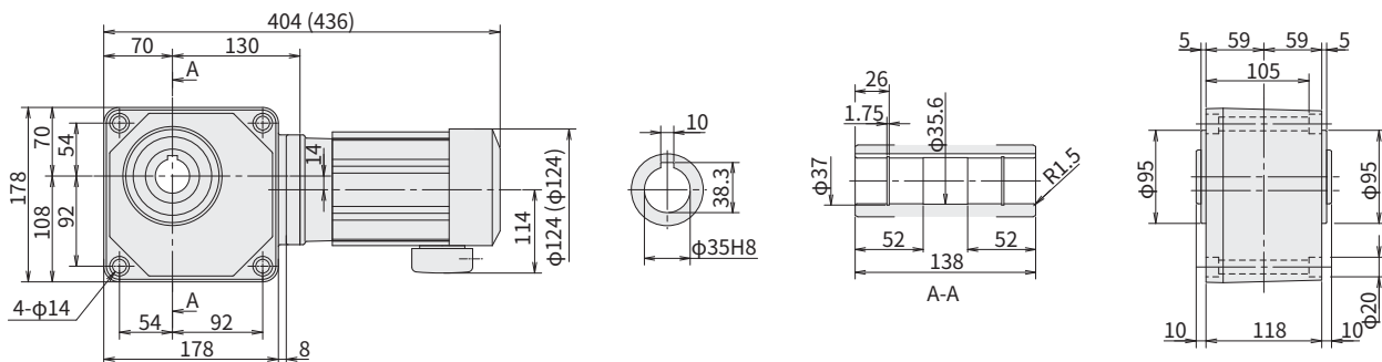
图 E37 RNYM05-1430-80~240 重量 16kg (RNYM05-1430-B-80~240) (重量 17kg)
