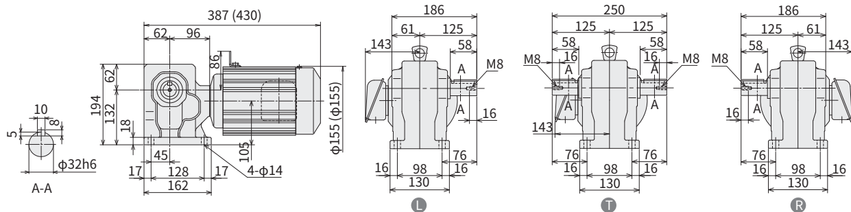
图 E366 RNHM08-43-B-40~60 重量 17kg (RNHM08-43-B-40~60) (重量 20kg)
