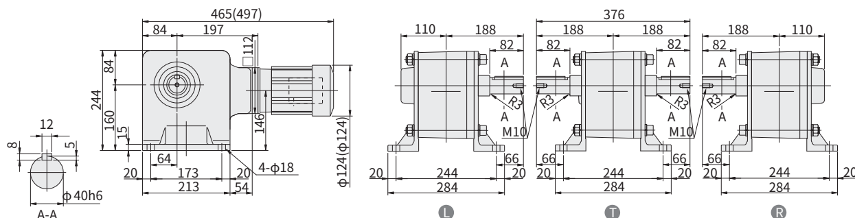
图 E354 RNHM02-1540-J1-600~1440 (RNHM02-1540-J1-B-600~1440) 重量 39kg (重量 40kg)
