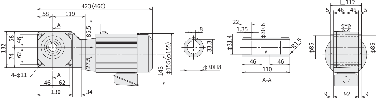
图 E160 RNYM05-1320-EP-5~30 (RNYM05-1320-EP-B-5~30) 重量 15kg (重量 17kg)
