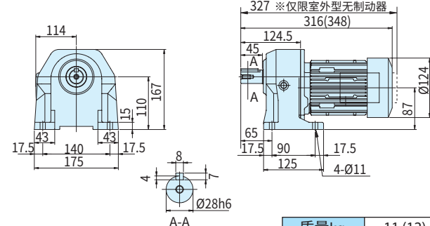
图C14 ZNHM05-1281-30~100 (ZNHM05-1281-B-30~100)
