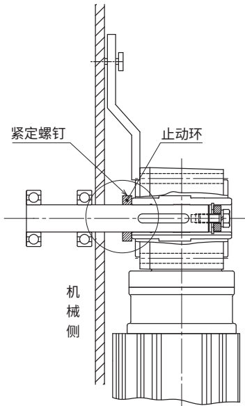
图 D5 用紧定螺钉和止动环固定 (从动轴无阶梯)
