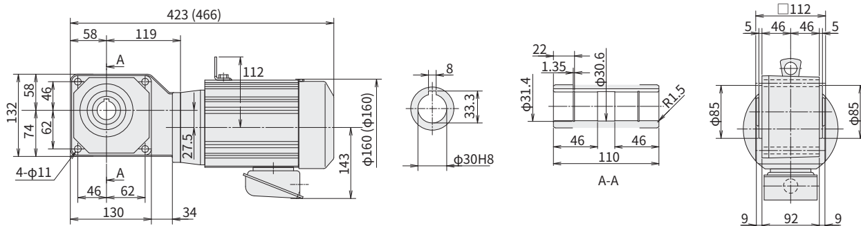
图 E49 RNYM1-1320-15~30 (RNYM1-1320-B-15~30) 重量 15kg (重量 17kg)
