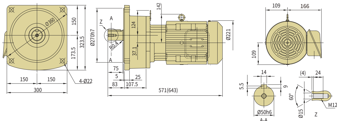
图 C104 ZNFM3-1501-AV-30~100 (ZNFM3-1501-AV-B-30~100)
