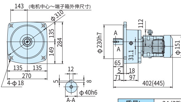
图C27 ZNFM1-1400-100~200 (ZNFM1-1400-B-100~200)
