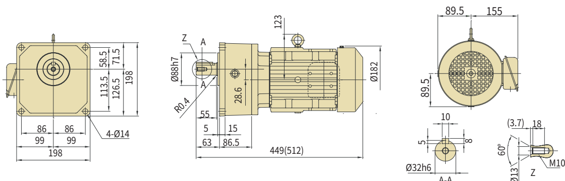
图 C99 ZNFM2-1401-AV-30~100 (ZNFM2-1401-AV-B-30~100)
