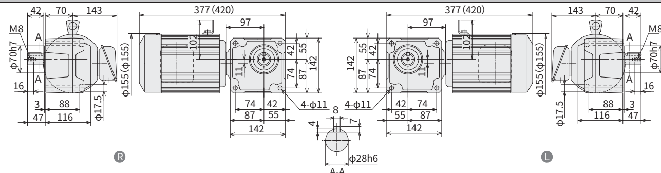
图 E257 RNFM1-370 R -5~30 重量 13kg (重量 16kg) • 安装本机器时请使用内六角螺钉 (M10)。 • 请注意电机是否与安装面干涉。
