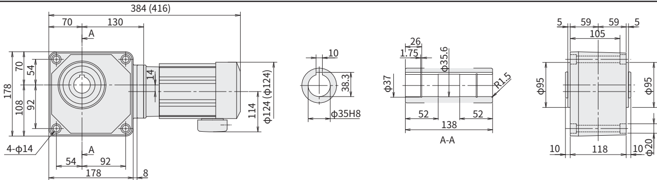
图 E23 RNYM02-1430-80~240 (RNYM02-1430-B-80~240)
