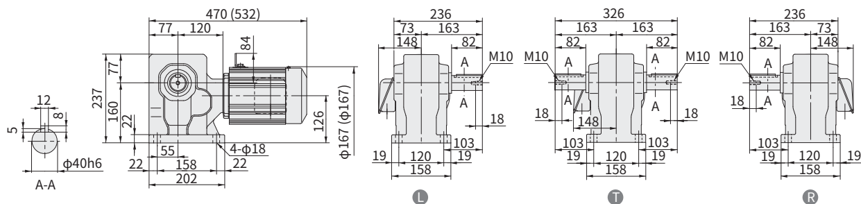
图 E377 RNHM2-53 1 -40~80 (RNHM2-53 1 -B-40~80) 重量 30kg (重量 34kg)
