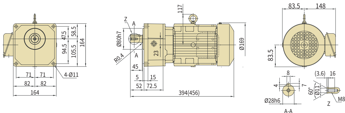
图 C93 ZNFM1-1321-AV-30~100 (ZNFM1-1321-AV-B-30~100)
