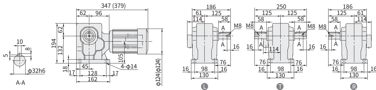
图 E420 RNHM03-40-EP-80~120 重量 14kg (RNHM03-40-EP-B-80~120) (重量 15kg)
