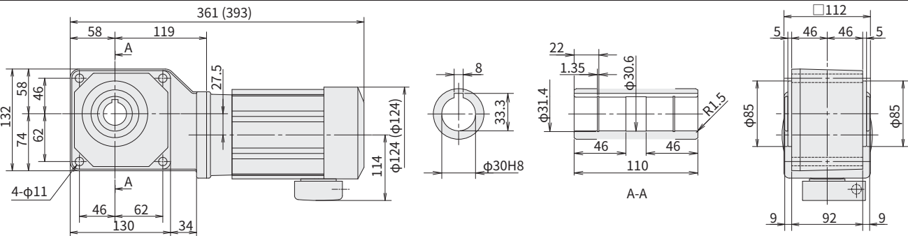
图 E21 RNYM02-1320-40~60 (RNYM02-1320-B-40~60)
