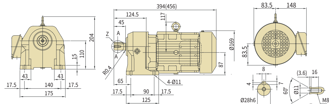
图 C89 ZNHM1-1280-AV-3~30 (ZNHM1-1280-AV-B-3~30)
