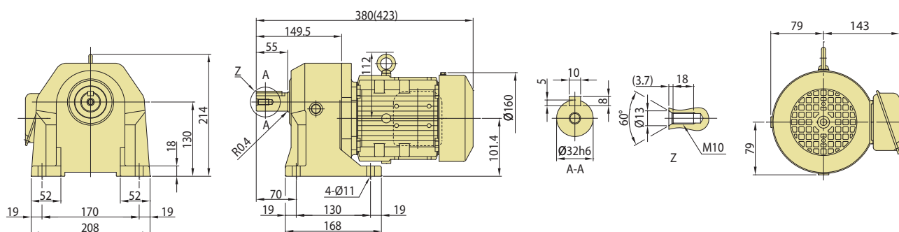
图 C85 ZNHM05-1320-AV-100~200 (ZNHM05-1320-AV-B-100~200)
