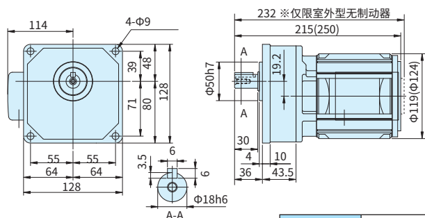
图C1 ZNFM01-1180-3~50 (ZNFM01-1180-B-3~50)
