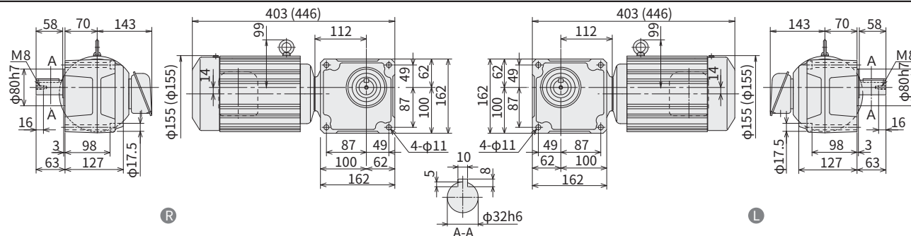
图 E258 RNFM1-43 R -40~60 重量 17kg (重量 20kg) • 安装本机器时请使用内六角螺钉 (M10)。 • 请注意电机是否与安装面干涉。
