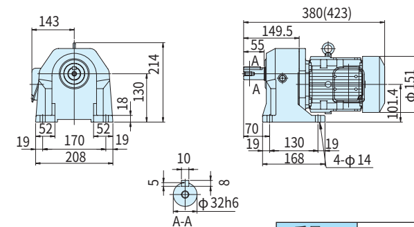
图C26 ZNFM1-1321-30~100 (ZNFM1-1321-B-30~100)
