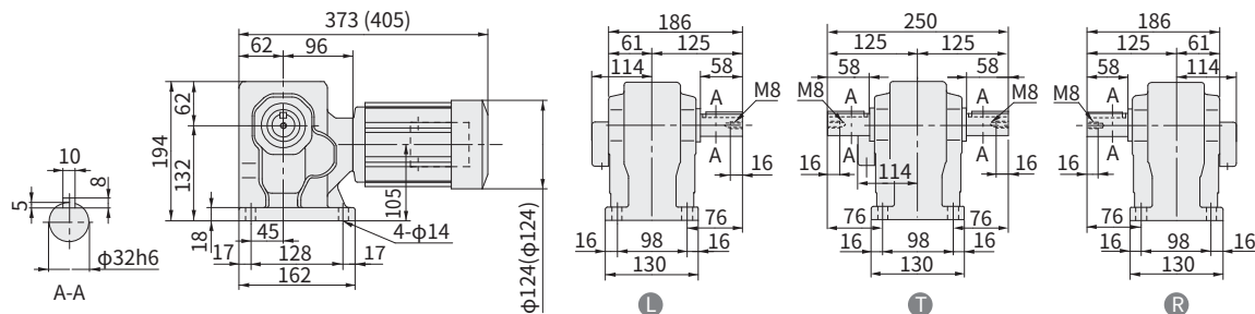
图 E421 RNHM03-45-EP-150~240 重量 15kg (RNHM03-45-EP-B-150~240) (重量 16kg)
