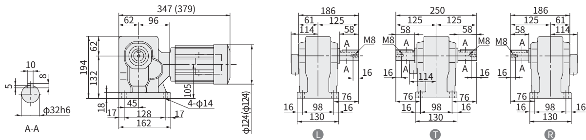
图 E412 RNHM02-40-EP-80~120 重量 14kg (RNHM02-40-EP-B-80~120) (重量 15kg)
