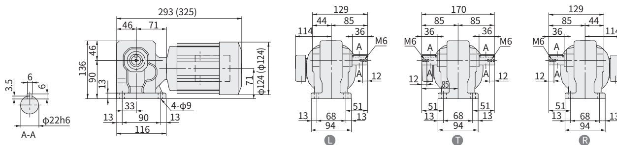
图 E348 RNHM02-23-B-40~60 重量 7.5kg (RNHM02-23-B-40~60) (重量 9.0kg)
