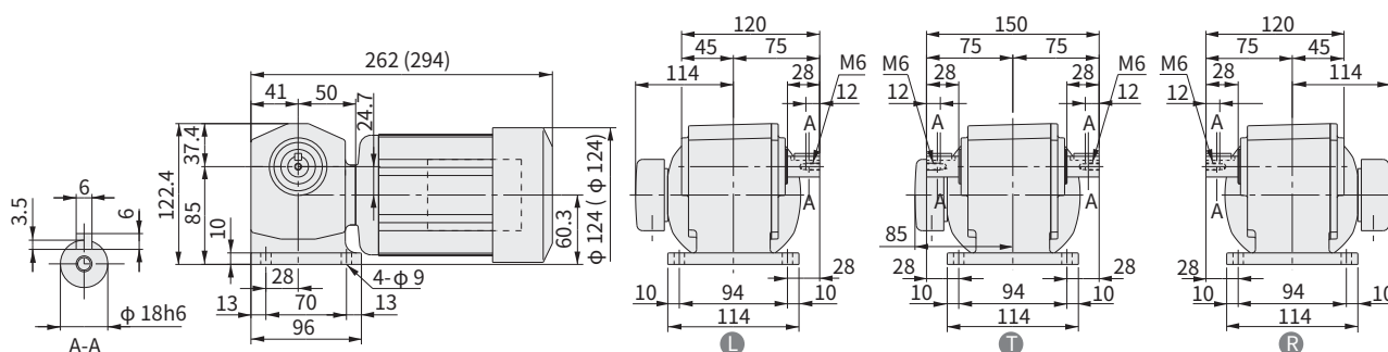
图 E347 RNHM02-190-B-5~30 重量 5.5kg (RNHM02-190-B-5~30) (重量 7.0kg)
