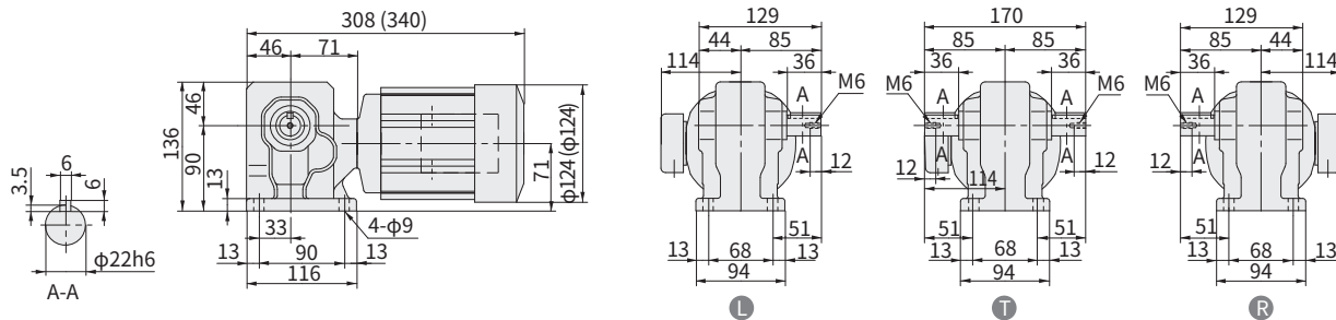
图 E418 RNHM03-270-EP-5~30 重量 8.5kg (RNHM03-270-EP-B-5~30) (重量 10kg)
