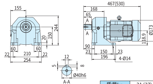
图C36 ZNHM3-1400-3~30 (ZNHM3-1400-B-3~30)
