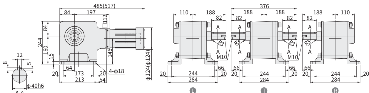
图 E364 RNHM05-1540 h6 -J1-300~1440 (RNHM05-1540 h6 -J1-B-300~1440) 重量 41kg (重量 42kg)
