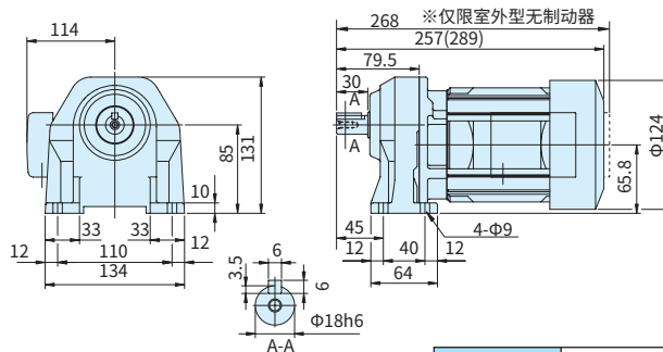
图C6 ZNHM02-1180-3~30 (ZNHM02-1180-B-3~30)
