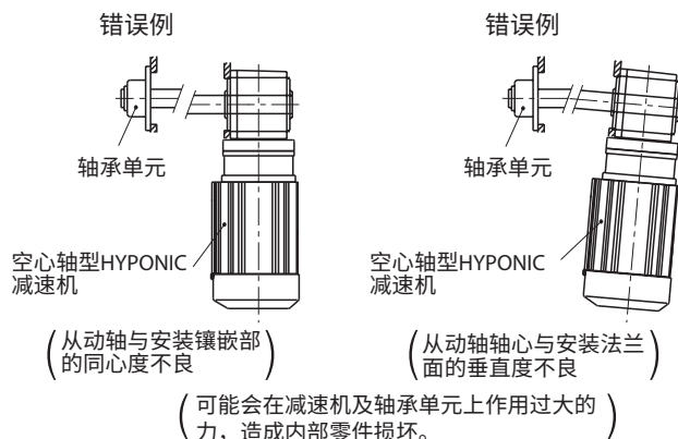
图 D11 法兰安装面
