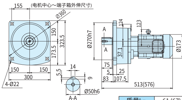
图C37 ZNFM3-1501-30~100 (ZNFM3-1501-B-30~100)
