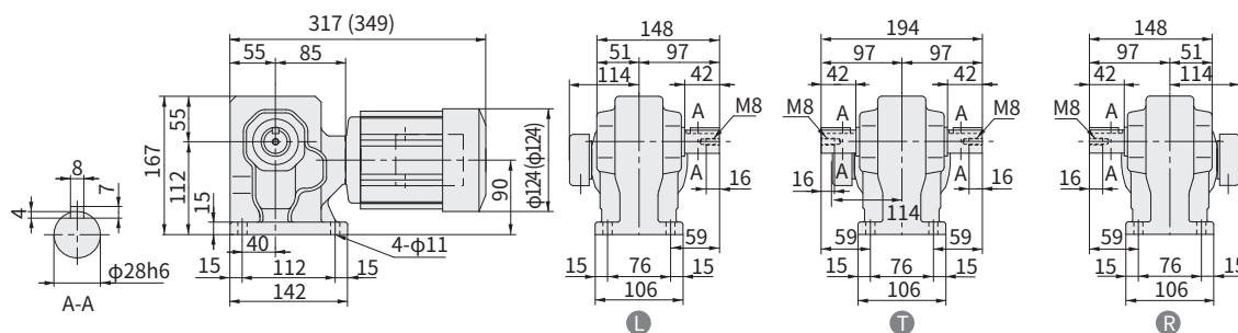
图 E387 RNHM01-35-AV-150~240 (RNHM01-35-AV-B-150~240) 重量 10kg (重量 11kg)
