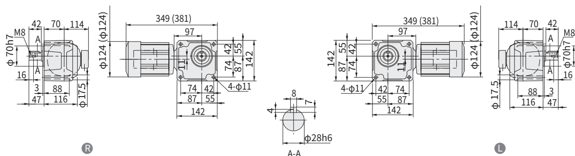
图 E245 RNF M05-33 R -40~60 重量 11kg (RNF M05-33 R -B-40~60) (重量 13kg) • 安装本机器时请使用内六角螺钉 (M10)。
