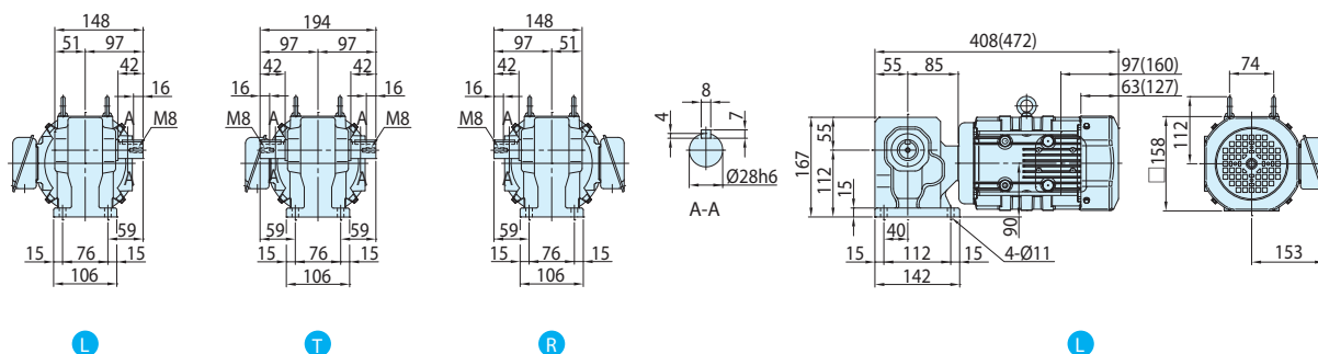
图E430 RNHM08-370 \frac{1}{2} -EP-5~30 (RNHM08-370 \frac{1}{2} -EP-B-5~30)
