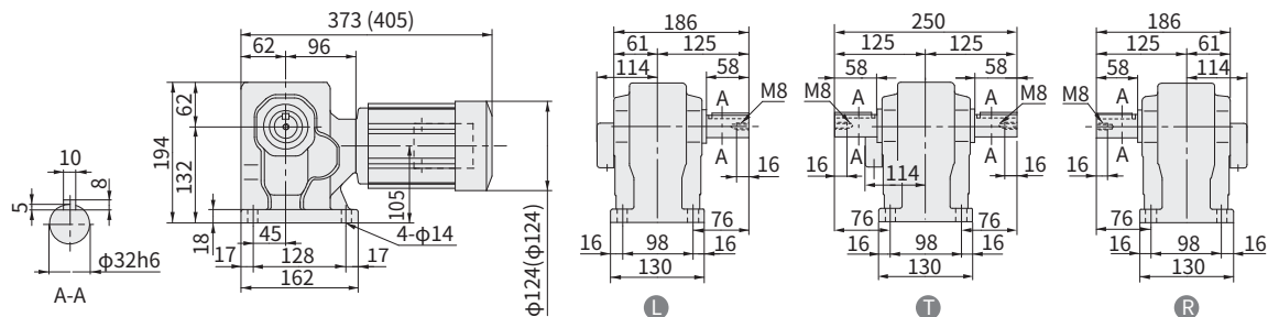
图 E413 RNHM02-45-EP-150~240 重量 15kg (RNHM02-45-EP-B-150~240) (重量 16kg)
