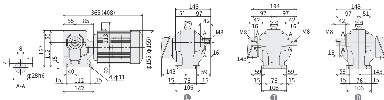
图 E400 RNHM05-370-AV-5~30 (RNHM05-370-AV-B-5~30) 重量 13.5kg (重量 16.5kg)
