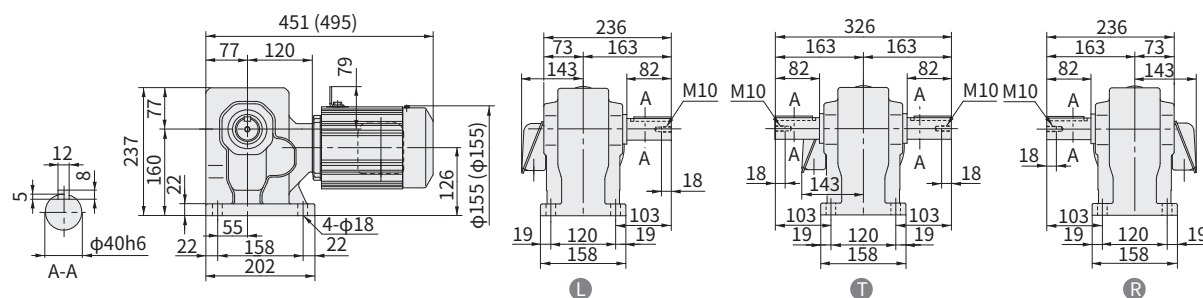
图 E403 RNHM05-55-AV-150~240 (RNHM05-55-AV-B-150~240) 重量 25kg (重量 28kg)
