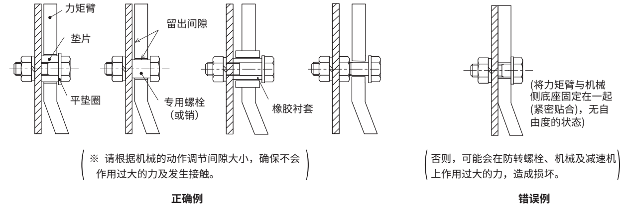
图 D9 防转螺栓部安装例 (A 部)
