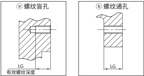
电机安装螺紋形状详情
