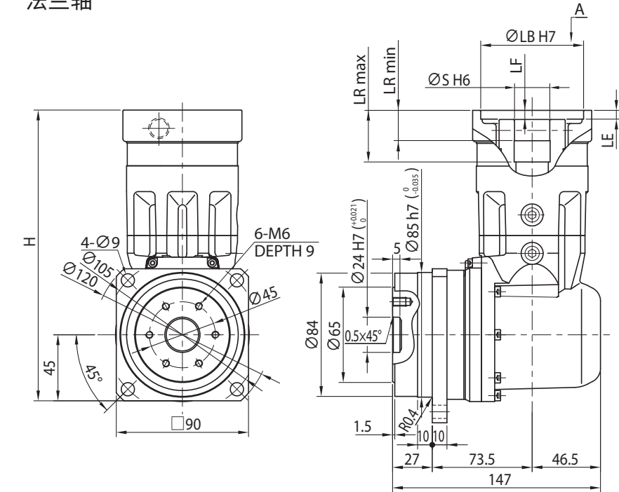
法兰轴
