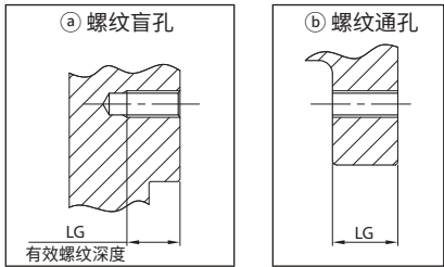
电机安装螺纹形状详情
