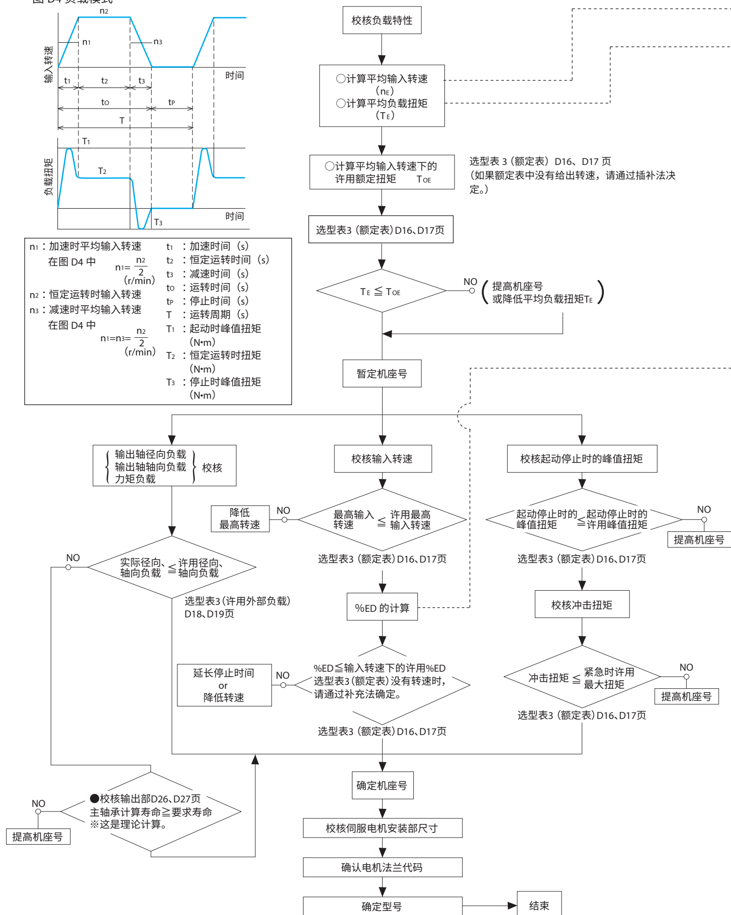
图 D4 负载模式
