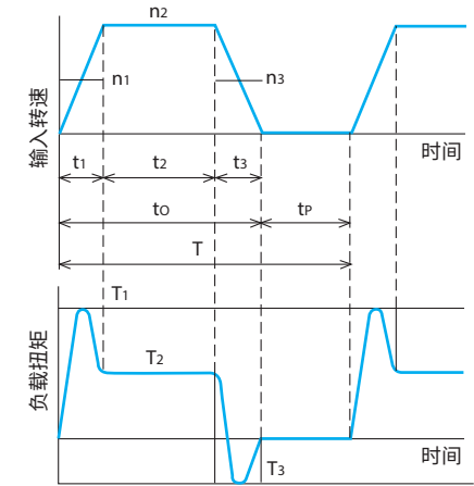
图 B4 负载模式
