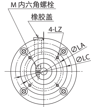
连接台形状: C
