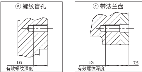
电机安装螺钉形状详情
