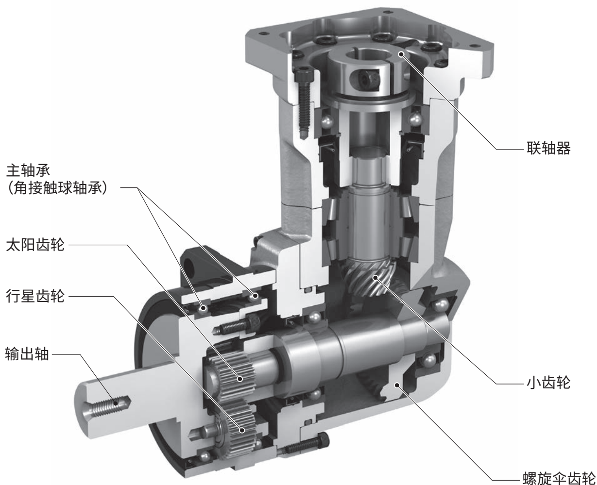
主要零件
