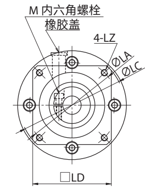
连接台形状: B
