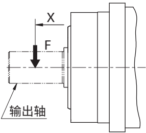
图 E3 径向负载位置
