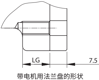
带电机用法兰盘的形状
