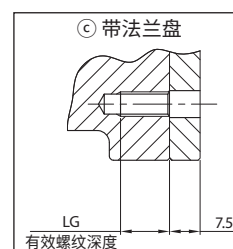
电机安装螺纹形状详情
