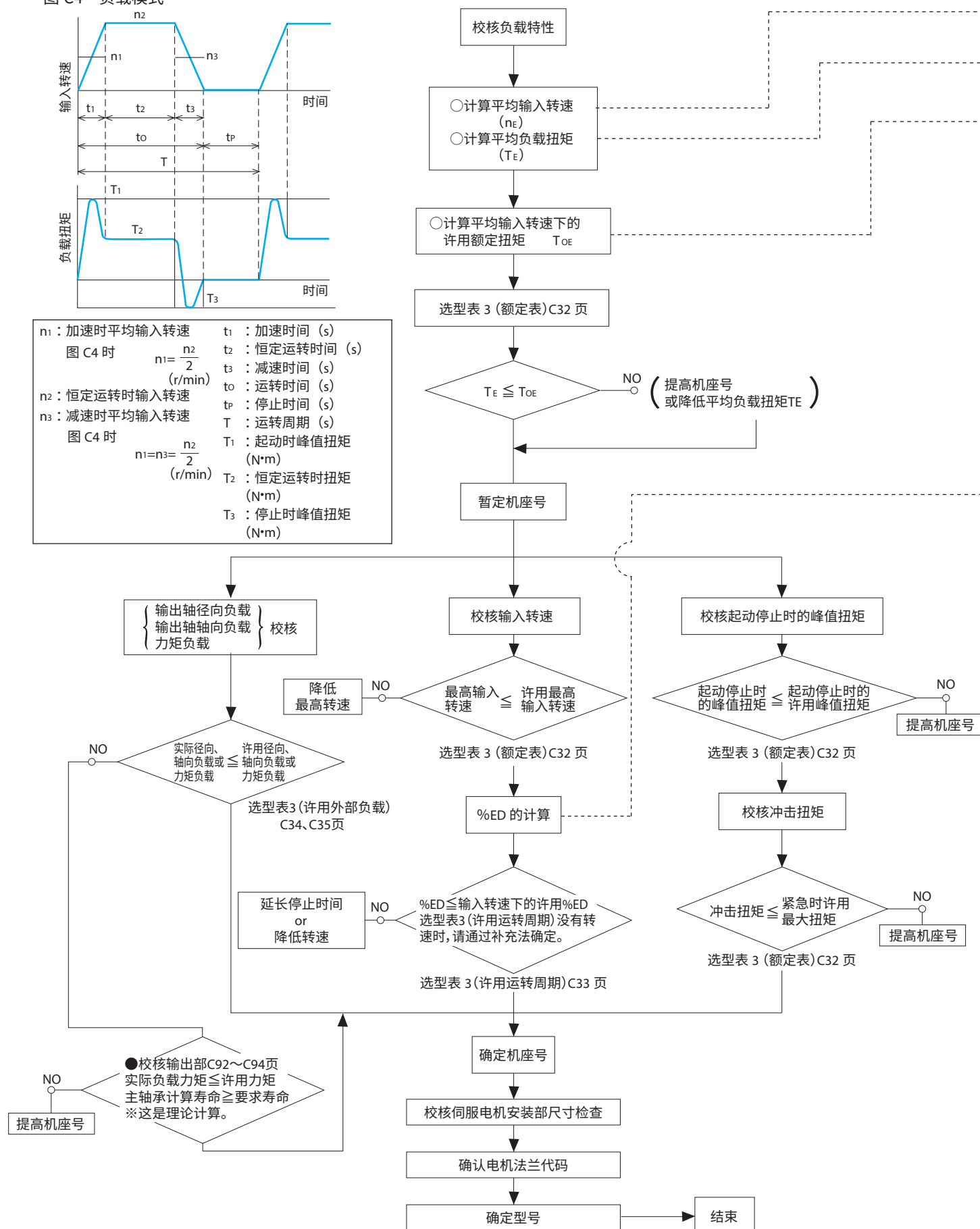
图 C4 负载模式
