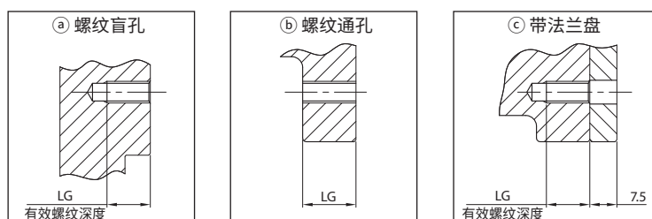
电机安装螺钉形状详情
