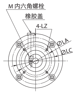
连接台形状: C ~A
