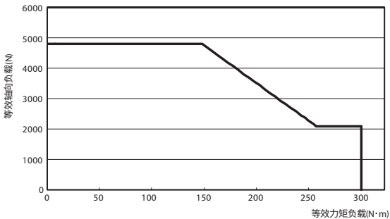
P120 许用力矩 - 轴向负载曲线图
