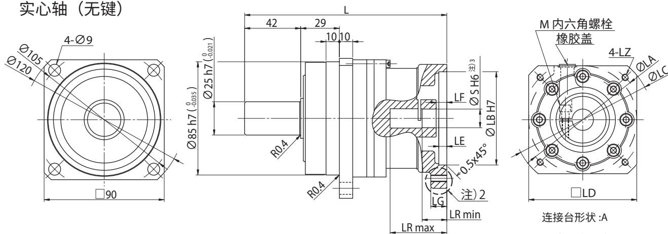
实心轴（有键）
