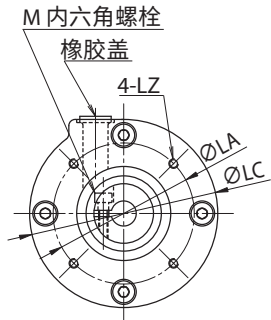
连接台形状: B ~A
