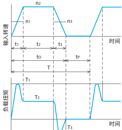
图 D4 负载模式
