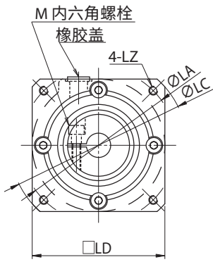
连接台形状：A
