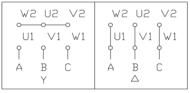
接 线 图
