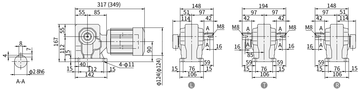
图 E350 RNHM02-35 h -150~240 重量 10kg (RNHM02-35 b -B-150~240) (重量 11kg)
