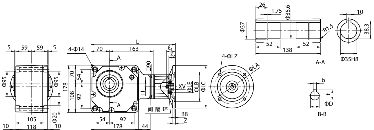
图 E412 RNYX - 1440 - [ 减速比 ]
