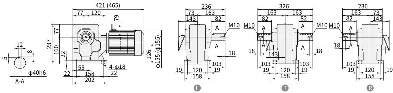
图 E402 RNHM05-50-AV-80~120 (RNHM05-50-AV-B-80~120)
