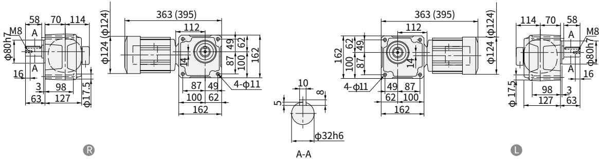
图 E246 RNFM05-40 L R -80~120 重量 14kg · 安装本机器时请使用内六角螺钉 (M10)。 (RNFM05-40 L R -B-80~120) (重量 16kg)
