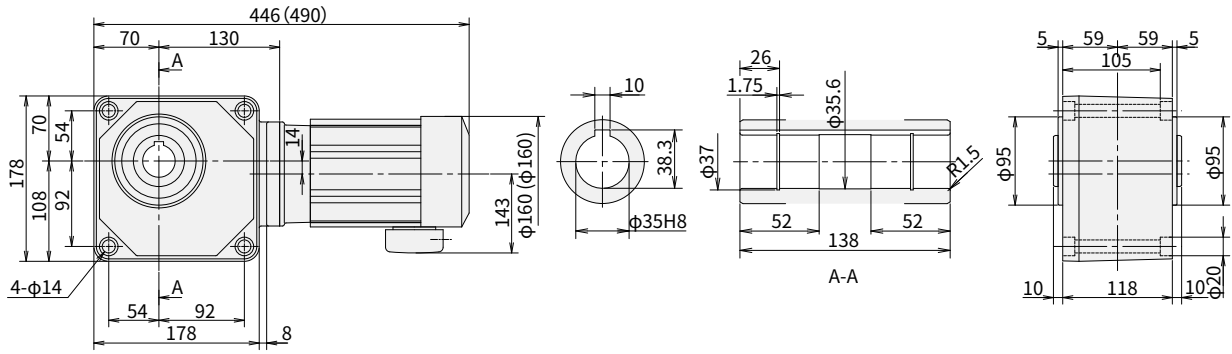
图 E163 RNYM05-1430-EP-80~120 (RNYM05-1430-EP-B-80~120) 重量 16kg (重量 17kg)
