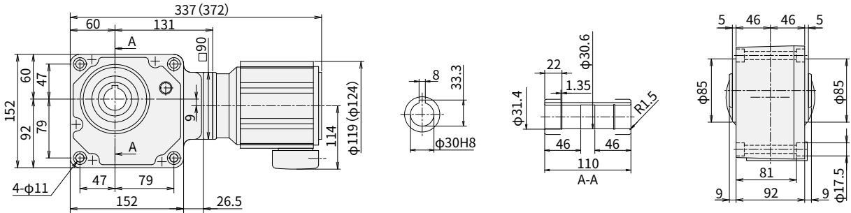
图 E14 RNYM01-1340-300~1440 (RNYM01-1340-B-300~1440) 重量 10kg (重量 11kg)
