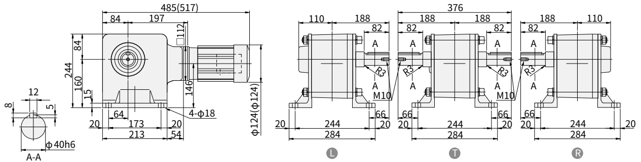
图 E397 RNHM02-1540-AVJ1-300~600 重量 41kg (RNHM02-1540-AVJ1-B-300~600) (重量 42kg)
