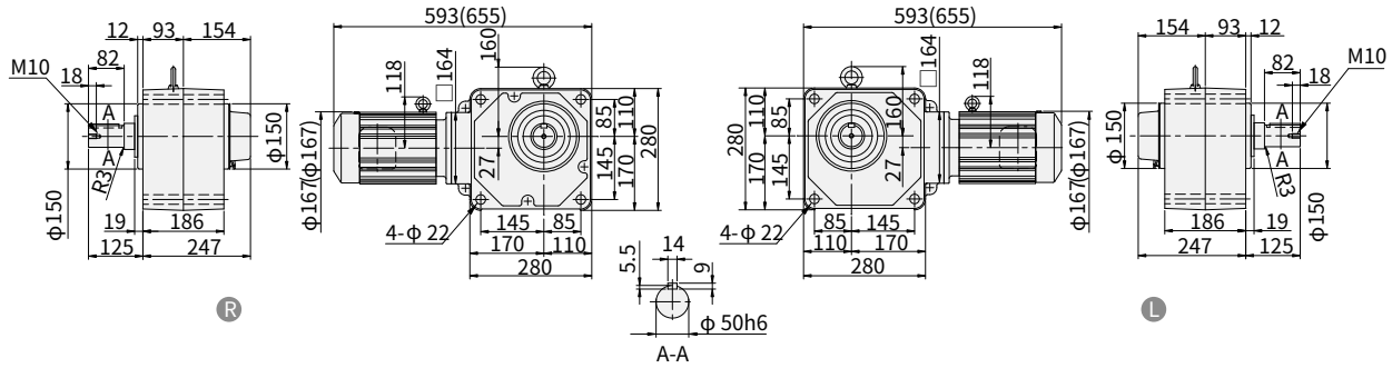
图 E268 RNFM2-1630 L R -X1-100,120 重量 57kg (RNFM2-1630 L R -X1-B-100,120) (重量 61kg) · 安装本机器时请使用内六角螺钉 (M20)。
