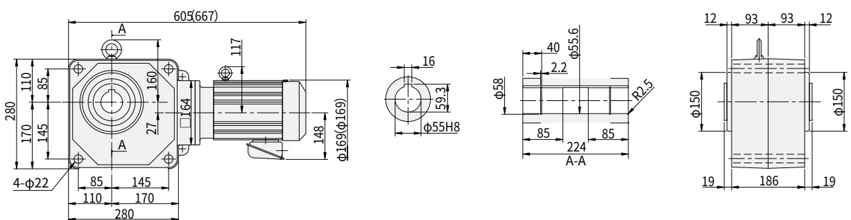
图 E72 RNYM2-1631-150~240 (RNYM2-1631-B-150~240) 重量 53kg (重量 57kg)
