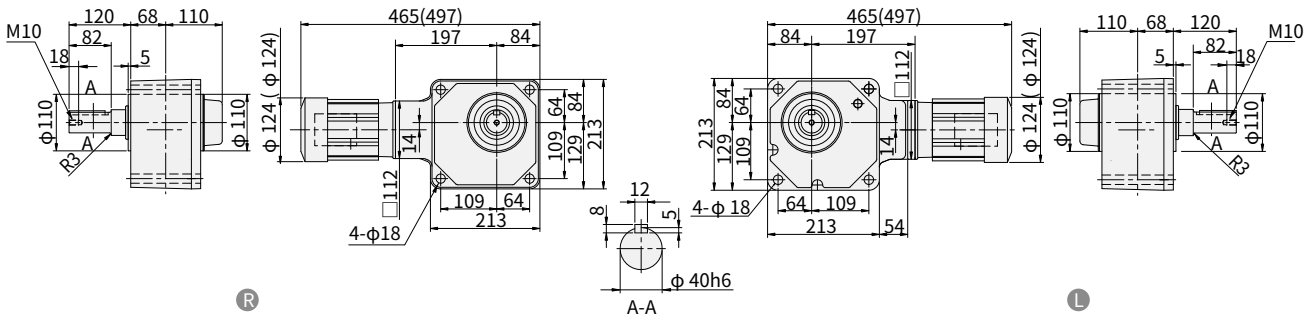
图 E236 RNFM02-1540 h -X1-300~480 重量 27.5kg · 安装本机器时请使用内六角螺钉 (M16)。 (RNFM02-1540 h -X1-B-300~480) (重量 28.5kg)
