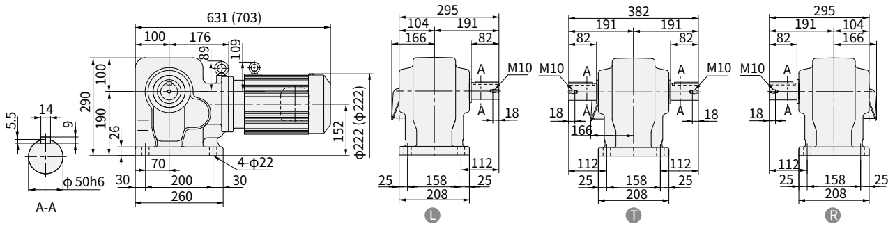
图 E382 RNHM5-63 \frac{1}{2} -10~50 (RNHM5-63 \frac{1}{2} -B-10~50) 重量 85kg (重量 94kg)
