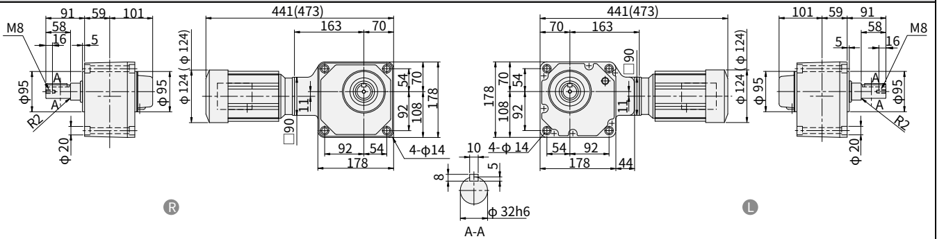
图 E313 RNFM03-1440 h -EPX1-300~600 重量 18.5kg · 安装本机器时请使用内六角螺钉 (M12)。 (RNFM03-1440 h -EPX1-B-300~600) (重量 19.5kg)
