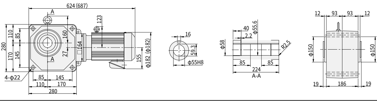
图 E79 RNYM3-1630-80~120 重量 57kg (RNYM3-1630-B-80~120) (重量 63kg)
