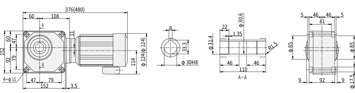
图 E145 RNYM02-1330-EP-80~240 重量 11kg (RNYM02-1330-EP-B-80~240) (重量 12kg)
