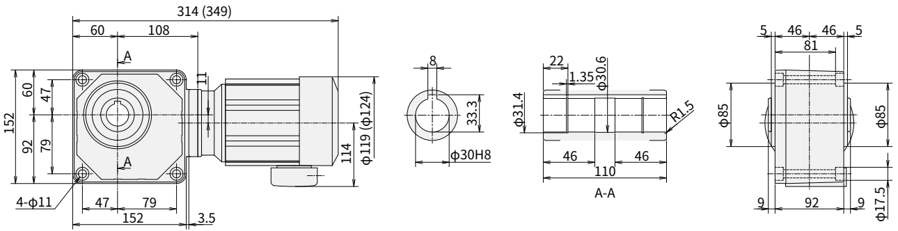
图 E13 RNYM01-1330-80~240 (RNYM01-1330-B-80~240) 重量 9.0kg (重量 10kg)
