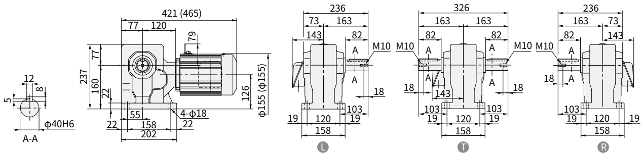
图 E367 RNHM08-50 h -80~120 重量 24kg (RNHM08-50 B -B-80~120) (重量 27kg)
