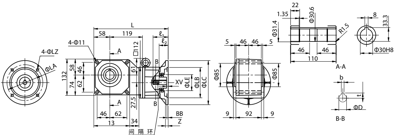
图 B407 RNYX - 1320 - [ 减速比 ]
