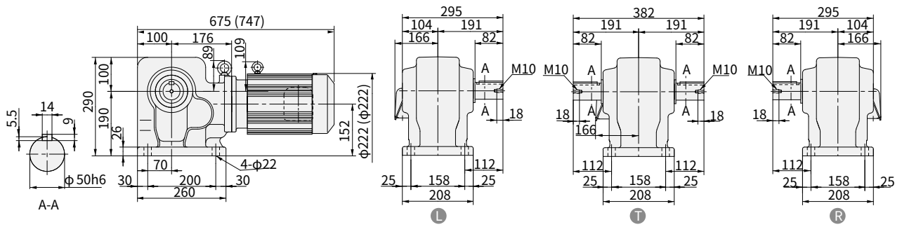
图 E383 RNHM8-64 \frac{1}{2} -10~40 (RNHM8-64 \frac{1}{2} -B-10~40) 重量 92kg (重量 101kg)
