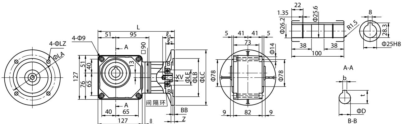
图 E406 RNYX - 1230 - [ 减速比 ]
