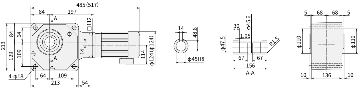
图 E39 RNYM05-1540-300~1440 (RNYM05-1540-B-300~1440) 重量 26kg (重量 27.5kg)
