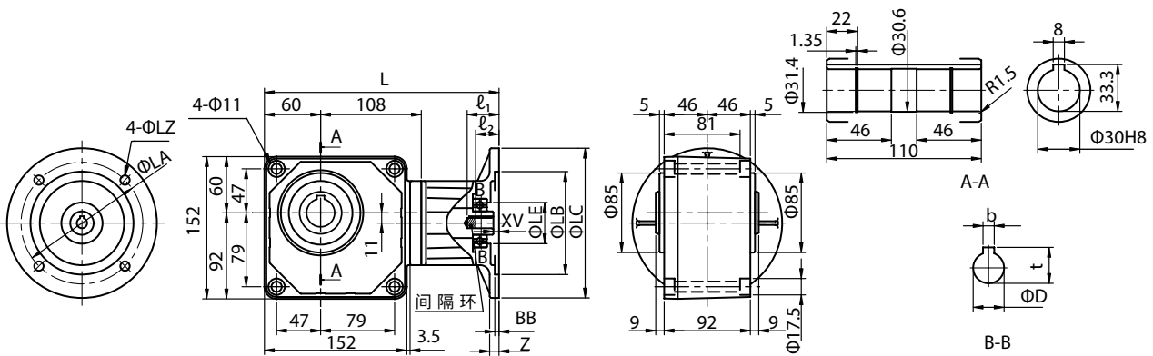
图 E408 RNYX - 1330 - [ 减速比 ]
