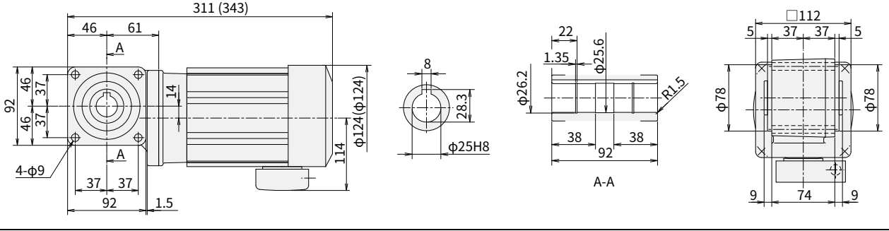
图 E31 RNYM05-1210-5~10 重量 9kg (RNYM05-1210-B-5~10) (重量 10kg)
