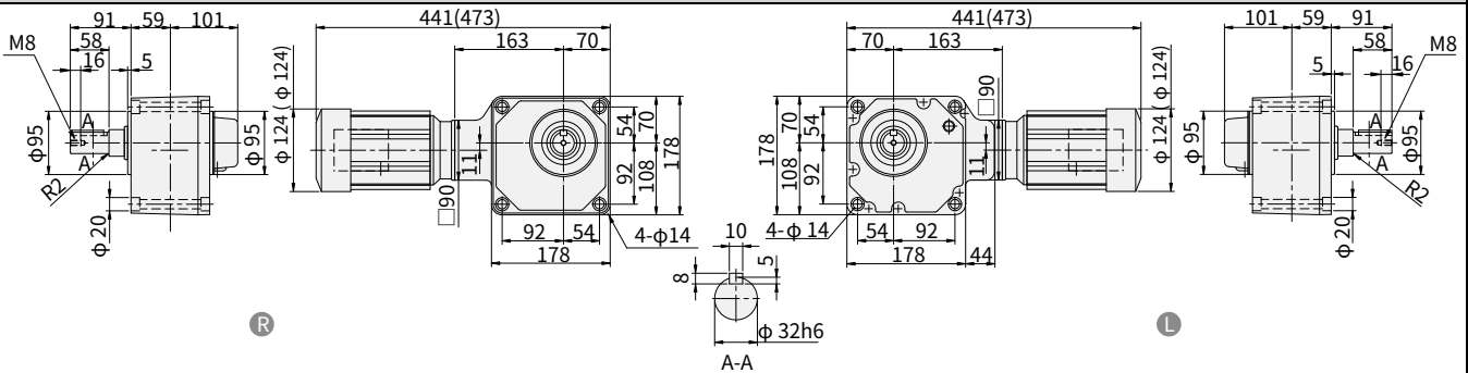
图 E315 RNFM03-1440 h -EPX1-720~1440 重量 18.5kg · 安装本机器时请使用内六角螺钉 (M12)。 (RNFM03-1440 h -EPX1-B-720~1440) (重量 19.5kg)
