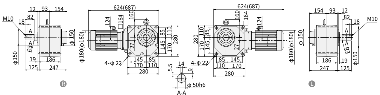
图 E271 RNFM3-1630 L R -X1-80~120 重量 62kg (RNFM3-1630 L R -X1-B-80~120) (重量 68kg) · 安装本机器时请使用内六角螺钉 (M20)。
