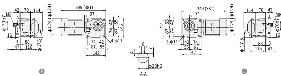
图 E245 RNFM05-33 L R -40~60 重量 11kg · 安装本机器时请使用内六角螺钉 (M10)。 (RNFM05-33 L R -B-40~60) (重量 13kg)
