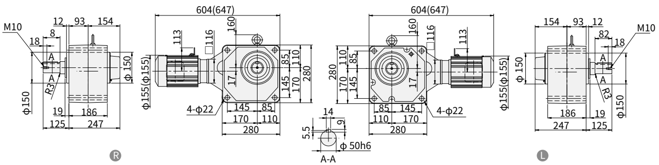
图 E293 RNFM05-1640 h -AVX1-300~1440 重量 73kg (RNFM05-1640 h -AVX1-B-300~1440) (重量 75kg) · 安装本机器时请使用内六角螺钉 (M20)。
