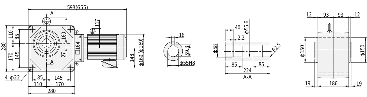
图 E62 RNYM1H-1630-100~120 (RNYM1H-1630-B-100~120) 重量 52kg (重量 56kg)
