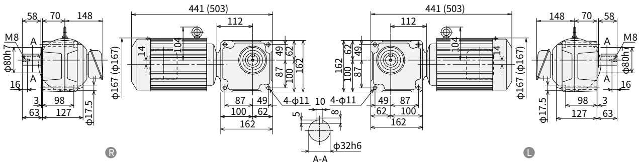
图 E294 RNFM1-470 h -AV-5~30 重量 21kg (RNFM1-470 h -AV-B-5~30) (重量 26kg) · 安装本机器时请使用内六角螺钉 (M10)。 · 请注意电机是否与安装面干涉。
