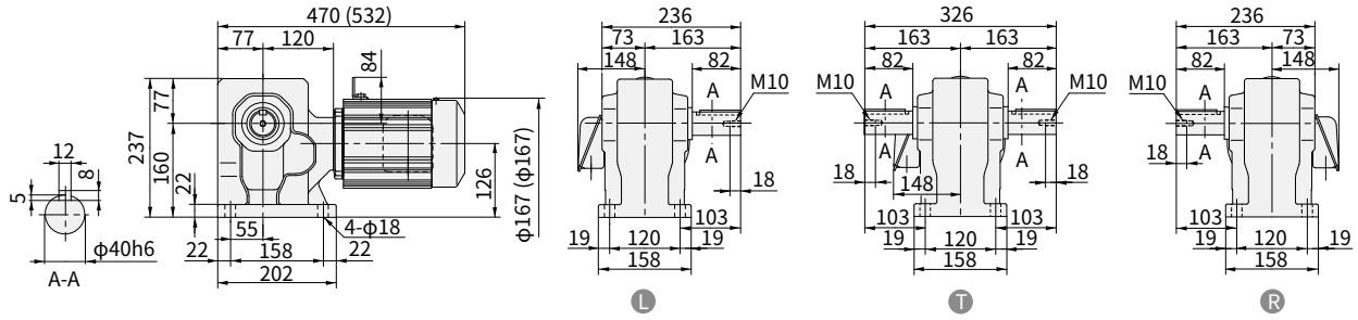
图 E374 RNHM1H-53 1/2 -40~80 (RNHM1H-53 1/2 -B-40~80) 重量 30kg (重量 34kg)
