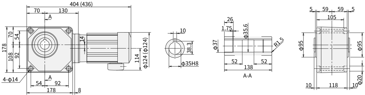
图 E37 RNYM05-1430-80~240 (RNYM05-1430-B-80~240) 重量 16kg (重量 17kg)
