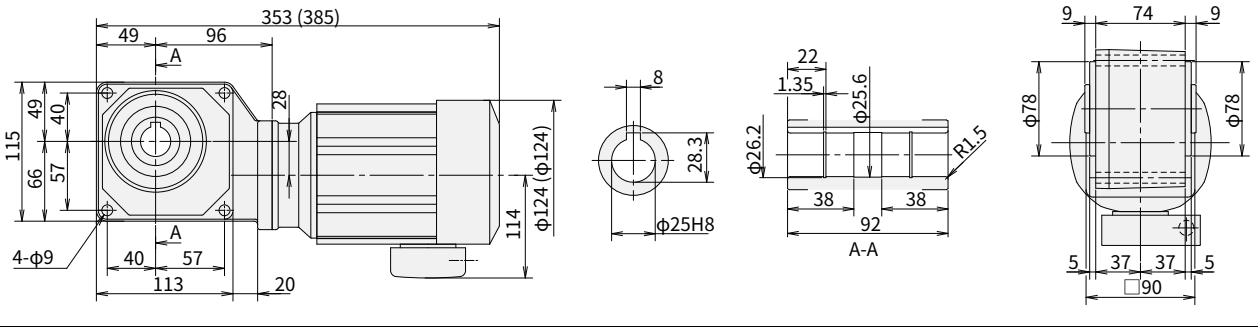
图 E32 RNYM05-1220-5~12 重量 9.5kg (RNYM05-1220-B-5~12) (重量 11kg)
