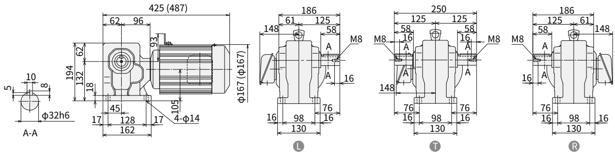
图 E376 RNHM2-470 1/2 -5~30 (RNHM2-470 1/2 -B-5~30) 重量 21.5kg (重量 26.5kg)
