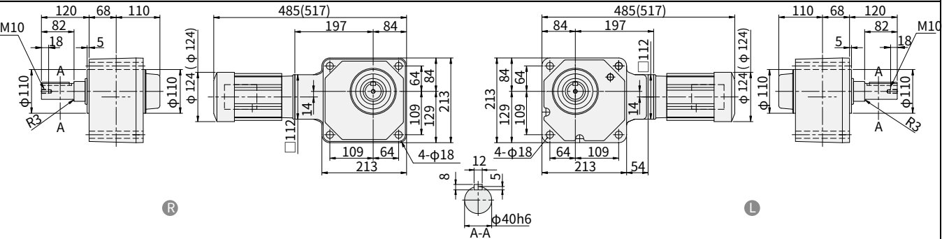
图 E314 RNFM03-1540 h -EPX1-300~600 重量 29kg · 安装本机器时请使用内六角螺钉 (M16)。 (RNFM03-1540 h -EPX1-B-300~600) (重量 30kg)
