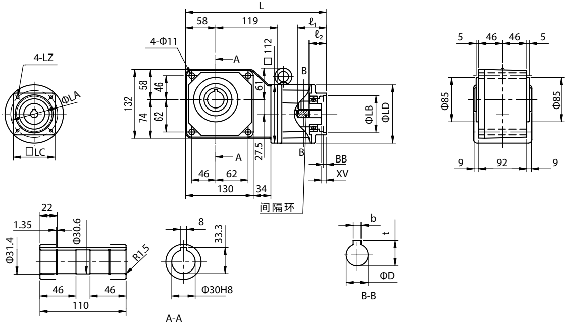
图 E424 RNYX - 1320 - [电机法兰代码] - [减速比]
