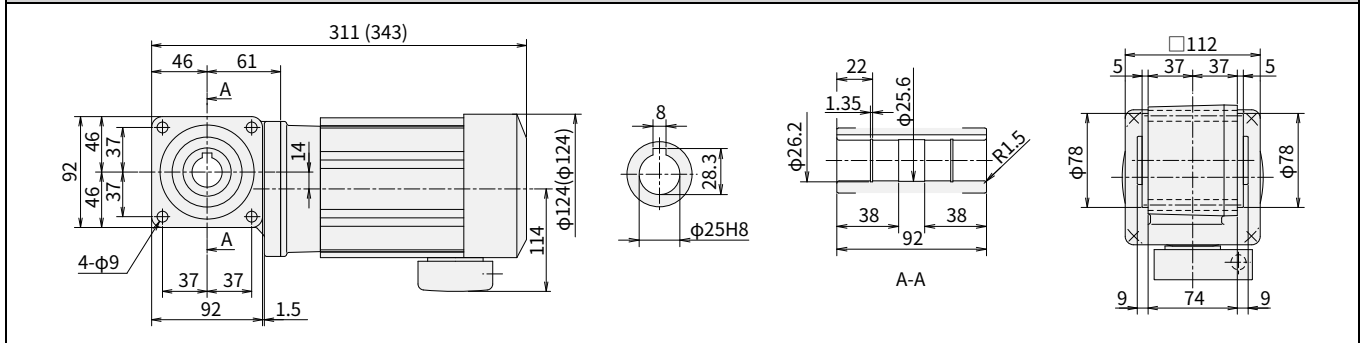
图 E26 RNYM03-1210-5~10 (RNYM03-1210-B-5~10) 重量 9.0kg (重量 10kg)
