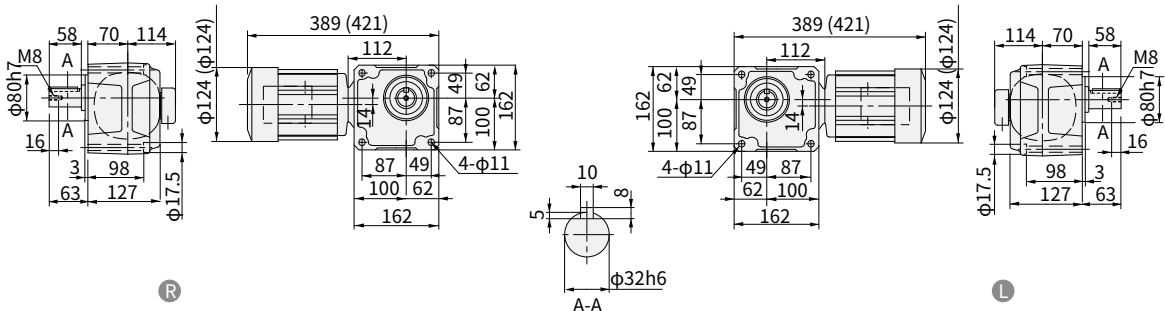
图 E247 RNFM05-45 L R -150~240 重量 15kg · 安装本机器时请使用内六角螺钉 (M10)。 (RNFM05-45 L R -B-150~240) (重量 16kg)
