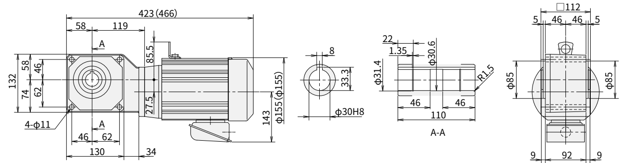
图 E118 RNYM05-1320-AV-5~30 重量 15kg (RNYM05-1320-AV-B-5~30) (重量 17kg)
