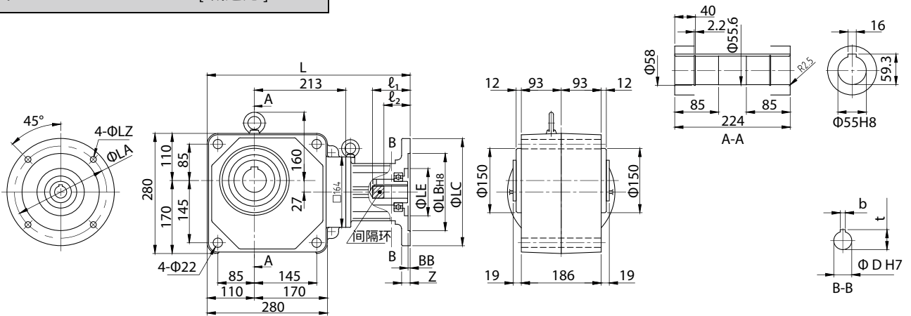
图 E417 RNYX - 1630 - [ 减速比 ]
