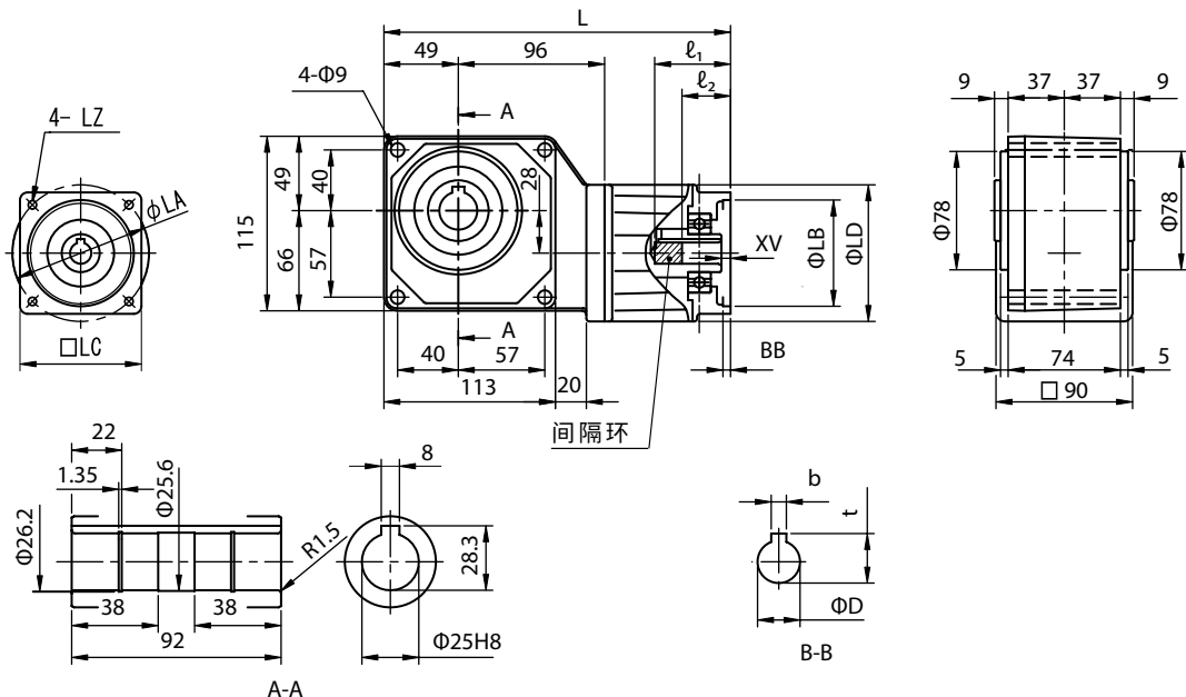
图 E423 RNYX - 1220 - [电机法兰代码] - [减速比]
