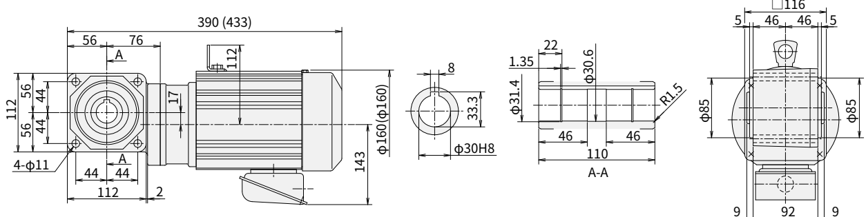
图 E46 RNYM1-1310-5~10 (RNYM1-1310-B-5~10) 重量 13kg (重量 16kg)
