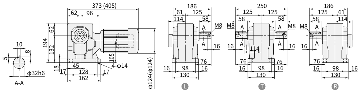
图 E421 RNHM03-45-EP-150~240 (RNHM03-45-EP-B-150~240) 重量 15kg (重量 16kg)
