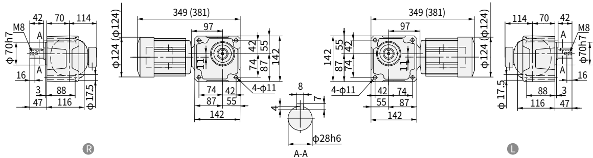
图 E282 RNFM02-33 L R -AV-40~60 重量 11kg · 安装本机器时请使用内六角螺钉 (M10)。 (RNFM02-33 L R -AV-B-40~60) (重量 13kg)
