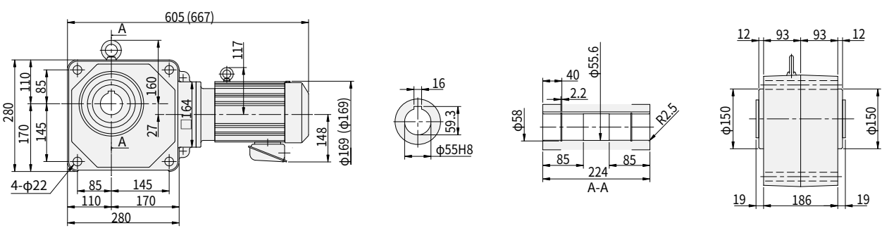
图 E63 RNYM1H-1631-150~240 (RNYM1H-1631-B-150~240) 重量 53kg (重量 57kg)
