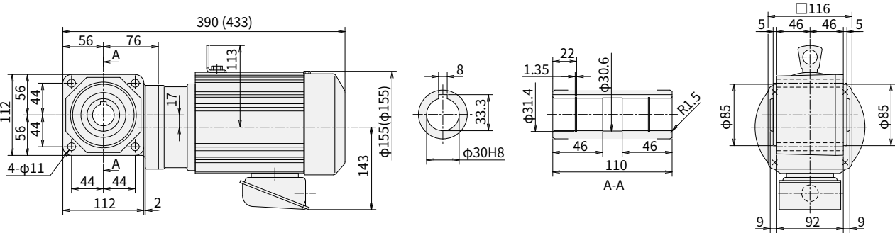
图 E117 RNYM05-1310-AV-5~10 重量 13kg (RNYM05-1310-AV-B-5~10) (重量 16kg)
