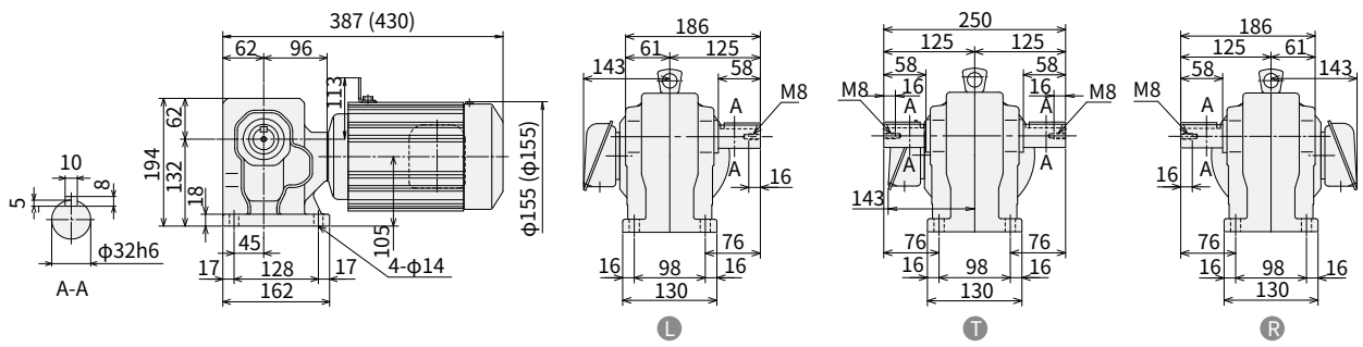
图 E401 RNHM05-43-AV-40~60 (RNHM05-43-AV-B-40~60)
