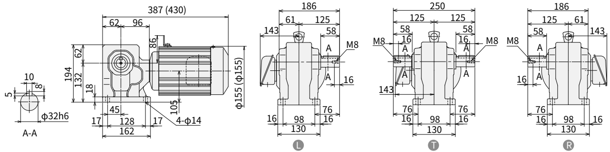
图 E366 RNHM08-43 h -40~60 重量 17kg (RNHM08-43 B -B-40~60) (重量 20kg)
