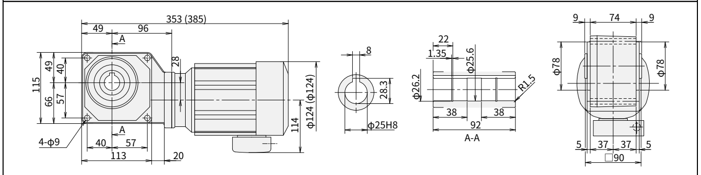
图 E27 RNYM03-1220-5~30 (RNYM03-1220-B-5~30) 重量 9.5kg (重量 11kg)
