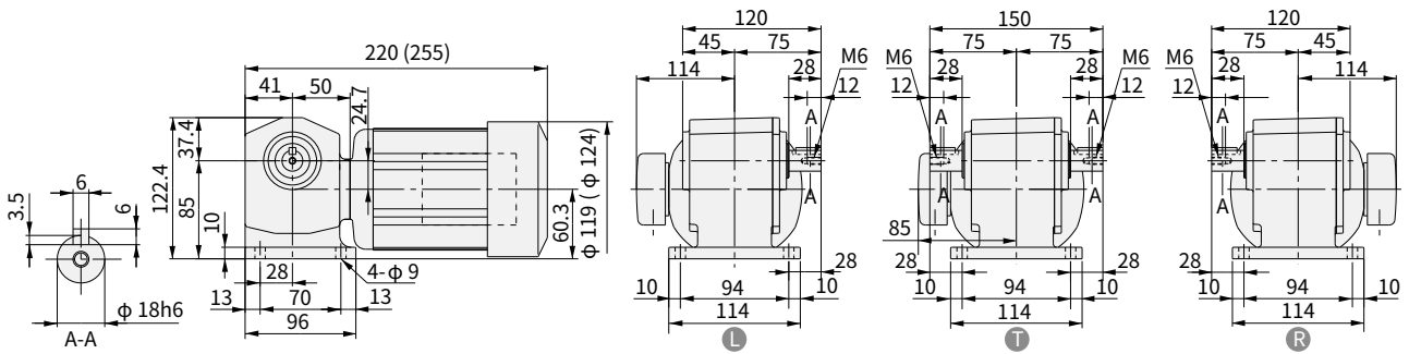
图 E342 RNHM01-190 5 -5~60 (RNHM01-190 B -5~60) 重量 4.5kg (重量 6.0kg)
