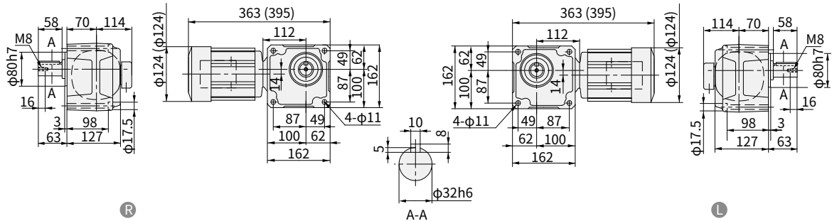
图 E283 RNFM02-40 L R -AV-80~120 重量 14kg · 安装本机器时请使用内六角螺钉 (M10)。 (RNFM02-40 L R -AV-B-80~120) (重量 16kg)
