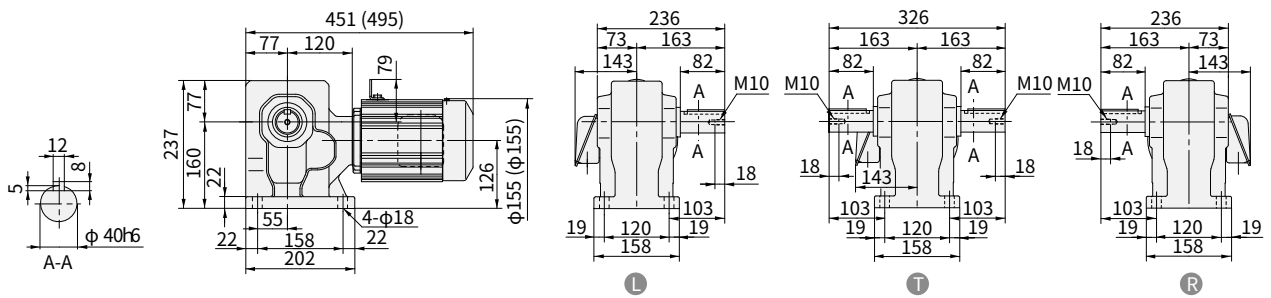
图 E368 RNHM08-55 h -150~240 重量 25kg (RNHM08-55 B -B-150~240) (重量 28kg)
