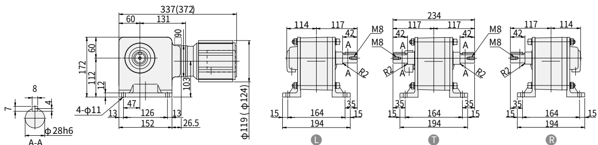
图 E345 RNHM01-1340 J1 -300~1440 (RNHM01-1340 J1-B -300~1440) 重量 15kg (重量 16kg)
