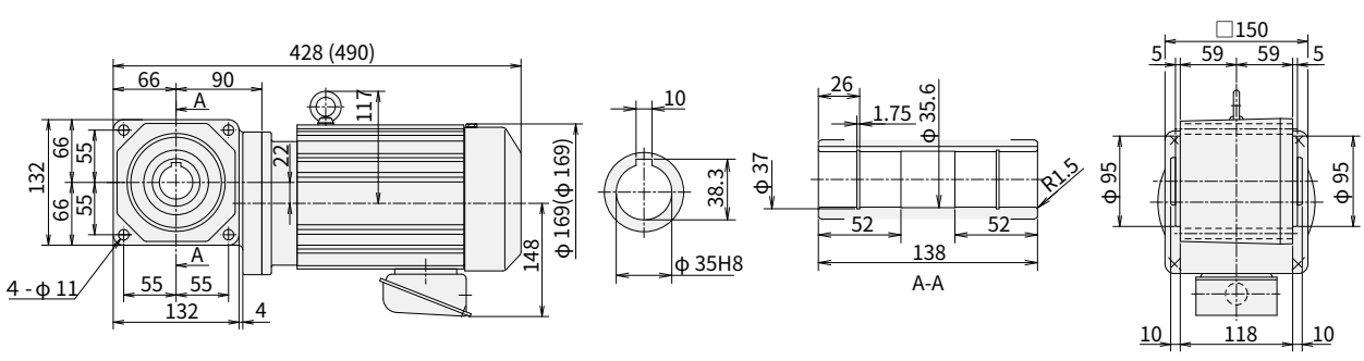
图 E64 RNYM2-1410-5~10 (RNYM2-1410-B-5~10) 重量 22kg (重量 26kg)
