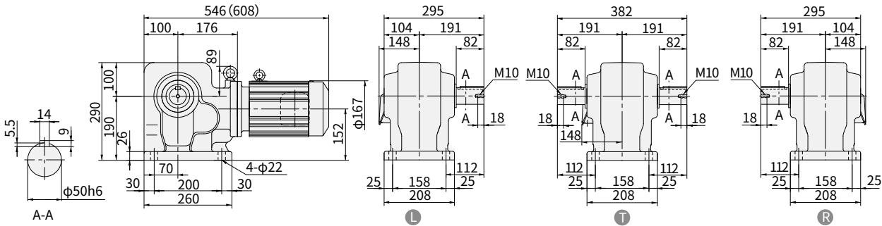
图 E375 RNHM1H-60 1/2 -100~120 (RNHM1H-60 1/2 -B-100~120) 重量 69kg (重量 73kg)
