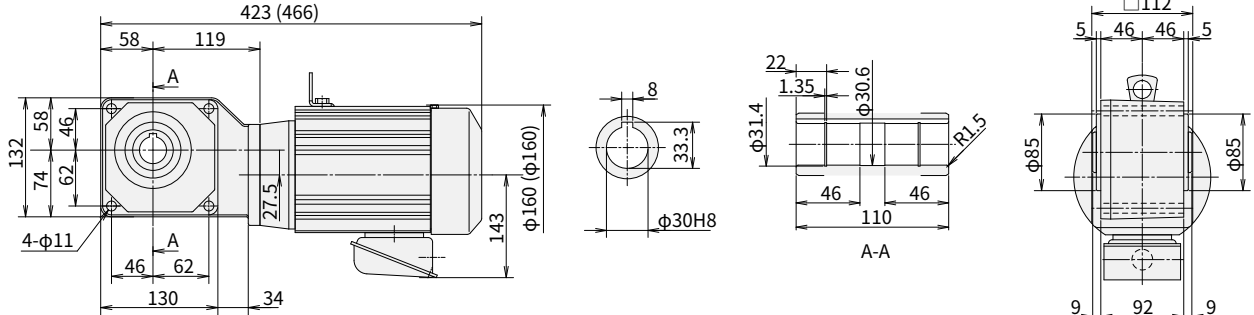
图 E47 RNYM1-1320-5~12 (RNYM1-1320-B-5~12) 重量 15kg (重量 17kg)
