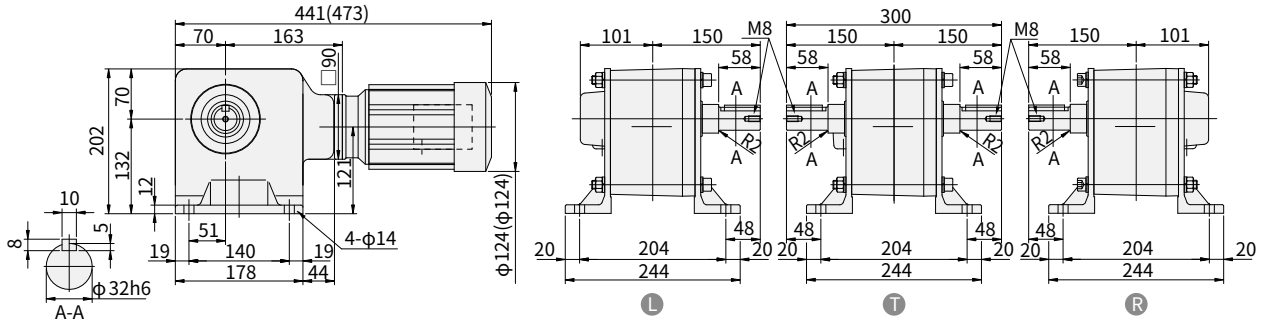
图 E396 RNHM02-1440-AVJ1-300~600 重量 24.5kg (RNHM02-1440-AVJ1-B-300~600) (重量 25.5kg)
