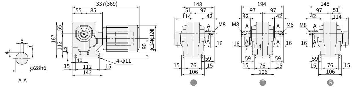
图 E411 RNHM02-33-EP-40~60 (RNHM02-33-EP-B-40~60) 重量 11kg (重量 12kg)
