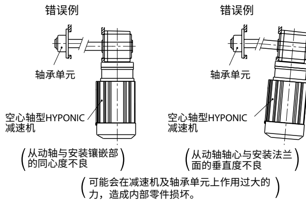
图 D11 法兰安装面
