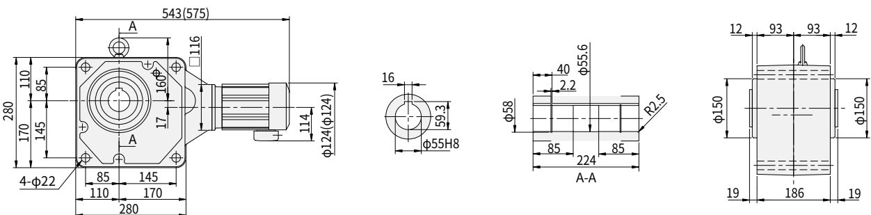
图 E40 RNYM05-1640-300~1440 (RNYM05-1640-B-300~1440) 重量 63kg (重量 64kg)
