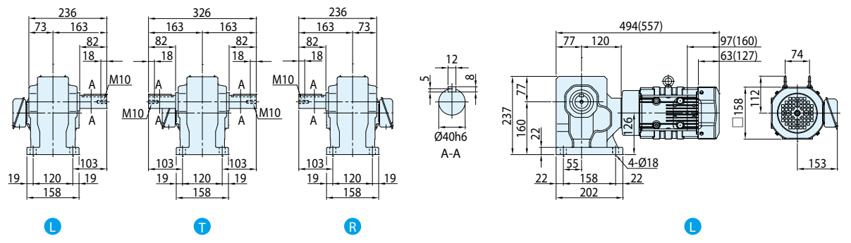
图E433 RNHM08-55 \frac{1}{2} -EP-150~240 (RNHM08-55 \frac{1}{2} -EP-B-150~240)
