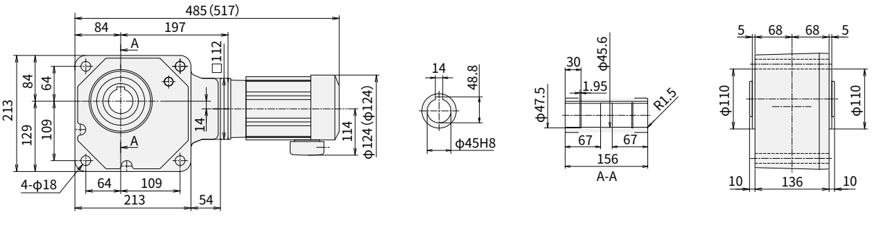
图 E30 RNYM03-1540-300~1440 重量 26kg (RNYM03-1540-B-300~1440) (重量 27.5kg)
