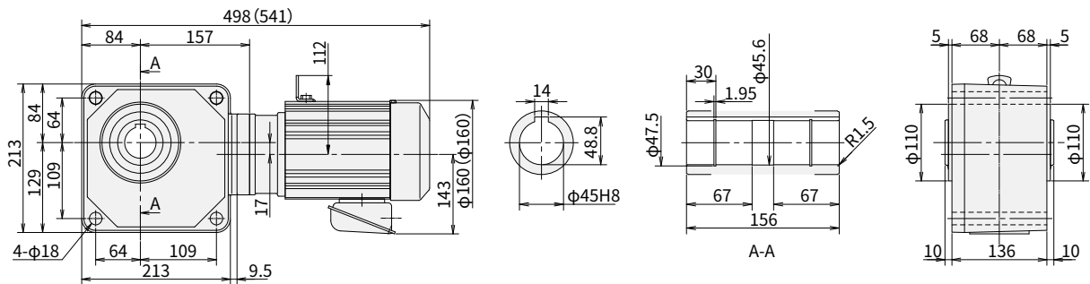
图 E164 RNYM05-1530-EP-80~240 (RNYM05-1530-EP-B-80~240) 重量 25kg (重量 28kg)
