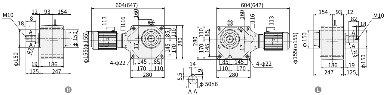
图 E321 RNFM05-1640 R -EPX1-300~1440 重量 73kg · 安装本机时请使用内六角螺钉 (M20)。 (RNFM05-1640 R -EPX1-B-300~1440) (重量 75kg)
