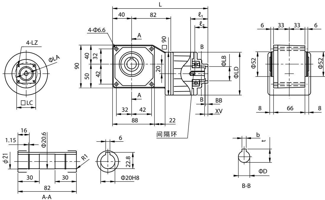
图 E422 RNYX - 1120 - [电机法兰代码] - [减速比]
