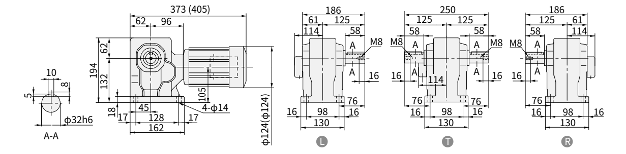
图 E413 RNHM02-45-EP-150~240 (RNHM02-45-EP-B-150~240) 重量 15kg (重量 16kg)
