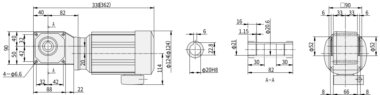
图 E142 RNYM02-1120-EP-20~30 (RNYM02-1120-EP-B-20~30)
