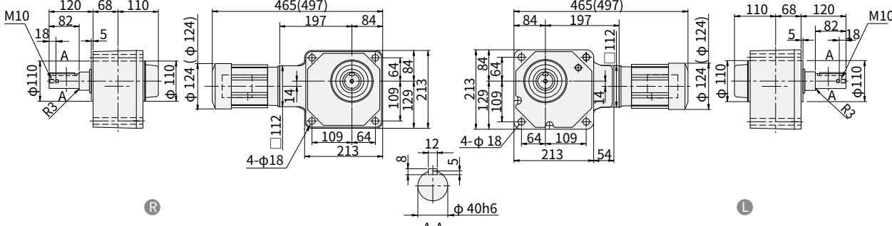
图 E238 RNFM02-1540 h -X1-600~1440 重量 27.5kg · 安装本机器时请使用内六角螺钉 (M16)。 (RNFM02-1540 h -X1-B-600~1440) (重量 28.5kg)
