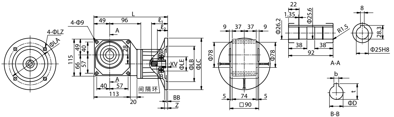
图 B405 RNYX - 1220 - [ 减速比 ]
