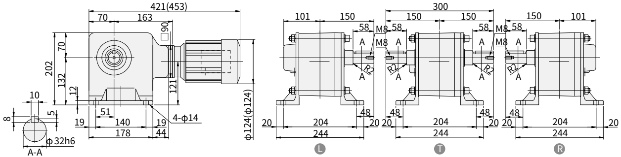
图 E351 RNHM02-1440 h -J1-300~480 重量 23kg (RNHM02-1440 b -J1-B-300~480) (重量 24.5kg)
