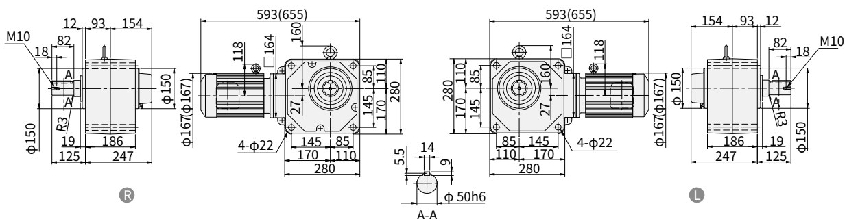
图 E296 RNFM1-1630 h -AVX1-100,120 重量 57kg (RNFM1-1630 h -AVX1-B-100,120) (重量 61kg) · 安装本机器时请使用内六角螺钉 (M20)。
