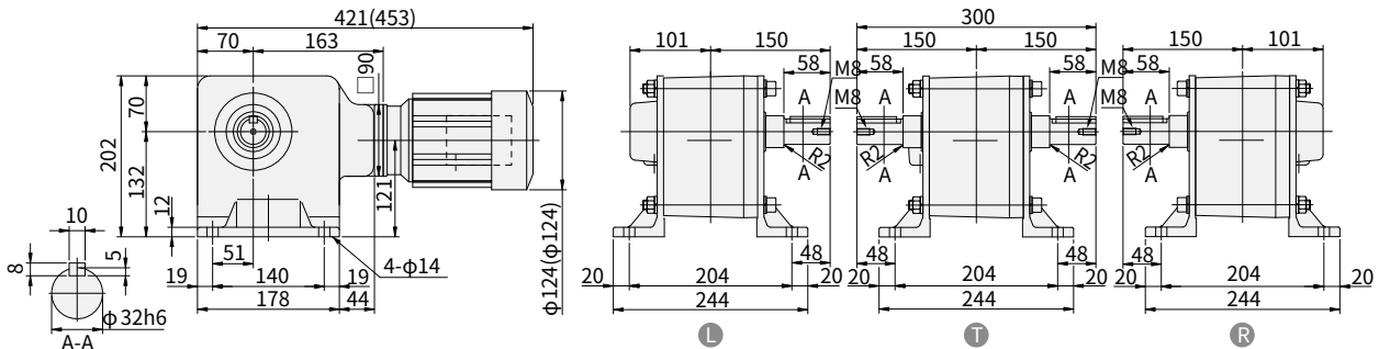
图 E353 RNHM02-1440 h -J1-600~1440 重量 23kg (RNHM02-1440 b -J1-B-600~1440) (重量 24.5kg)
