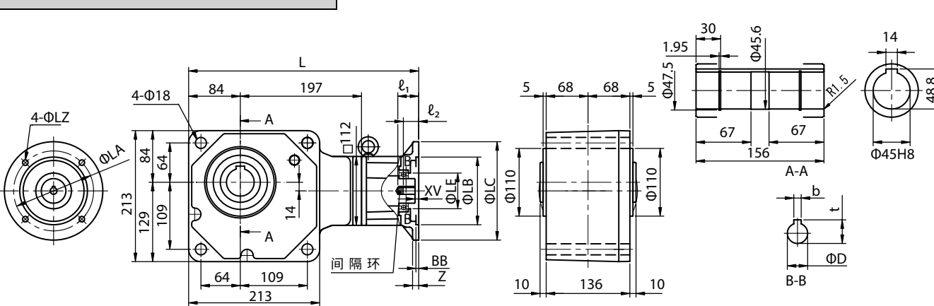
图 E415 RNYX - 1540 - [ 减速比 ]
