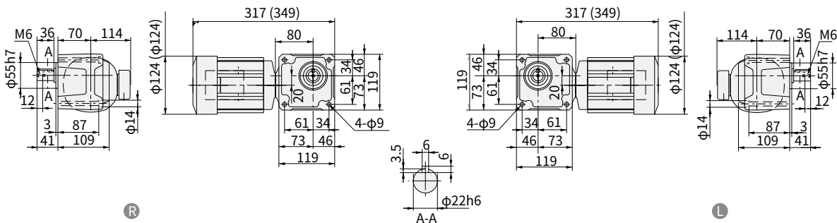
图 E239 RNFM03-270 h -5~30 重量 9.0kg · 安装本机器时请使用内六角螺钉 (M8)。 (RNFM03-270 h -B-5~30) (重量 10.5kg)
