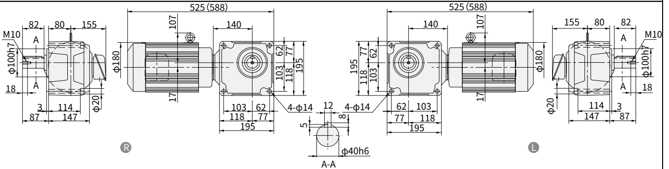
图 E270 RNFM3-54 h R -10~60 重量 34kg (RNFM3-54 h R -B-10~60) (重量 40kg) · 安装本机器时请使用内六角螺钉 (M12)。 · 请注意电机是否与安装面干涉。
