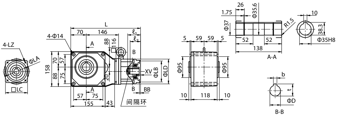
图 E425 RNYX - 1420 - [电机法兰代码] - [减速比]
