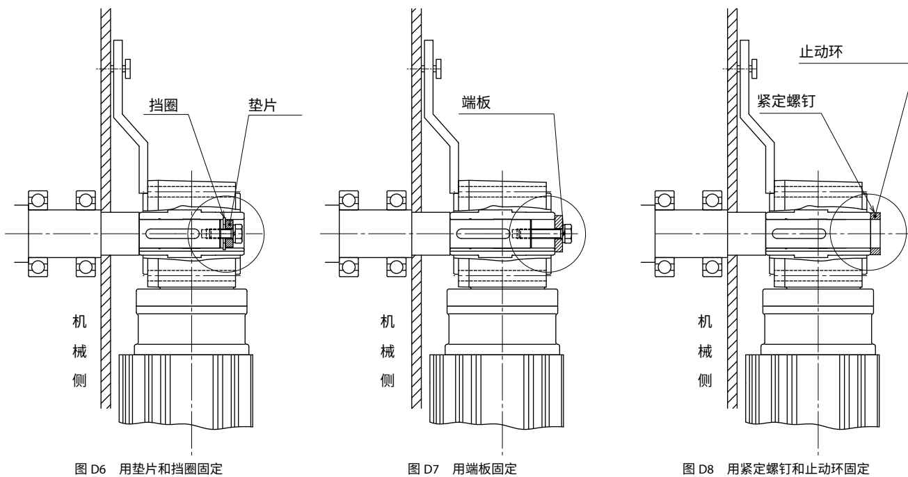
图 D6 用垫片和挡圈固定
