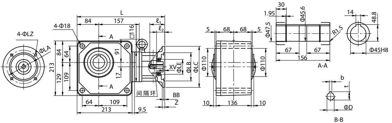
图 E413 RNYX - 1530 - [ 减速比 ]
