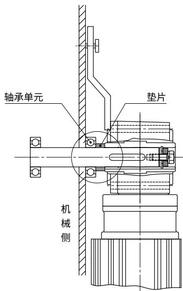
图 D4 用垫片固定 (从动轴无阶梯)
