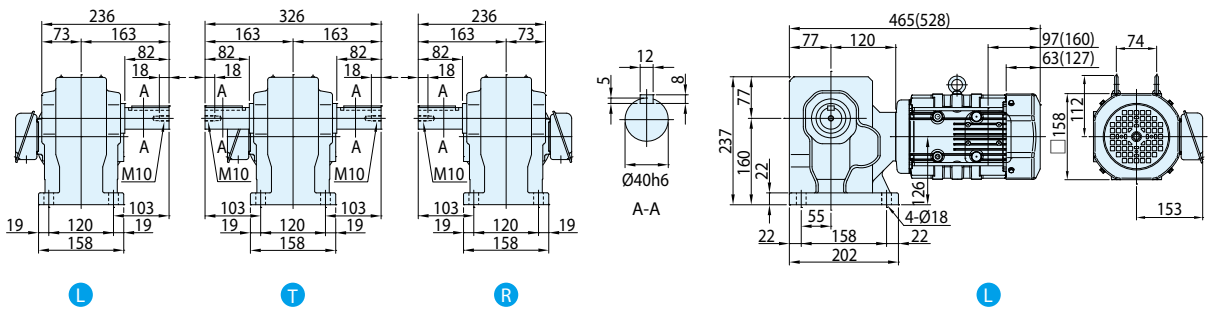
图E432 RNHM08-50 \frac{1}{2} -EP-80~120 (RNHM08-50 \frac{1}{2} -EP-B-80~120)
