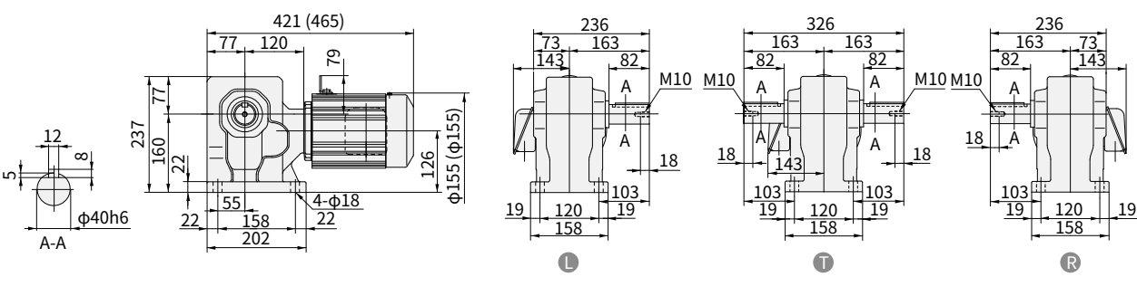
图 E428 RNHM05-50-EP-80~120 重量 24kg (RNHM05-50-EP-B-80~120) (重量 27kg)
