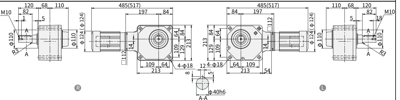
图 E308 RNFM02-1540 R -EPX1-720~1440 重量 29kg · 安装本机器时请使用内六角螺钉 (M16)。 (RNFM02-1540 L -EPX1-B-720~1440) (重量 30kg)
