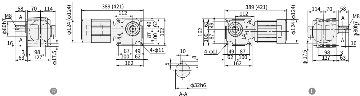
图 E284 RNFM02-45 L R -AV-150~240 重量 15kg · 安装本机器时请使用内六角螺钉 (M10)。 (RNFM02-45 L R -AV-B-150~240) (重量 16kg)
