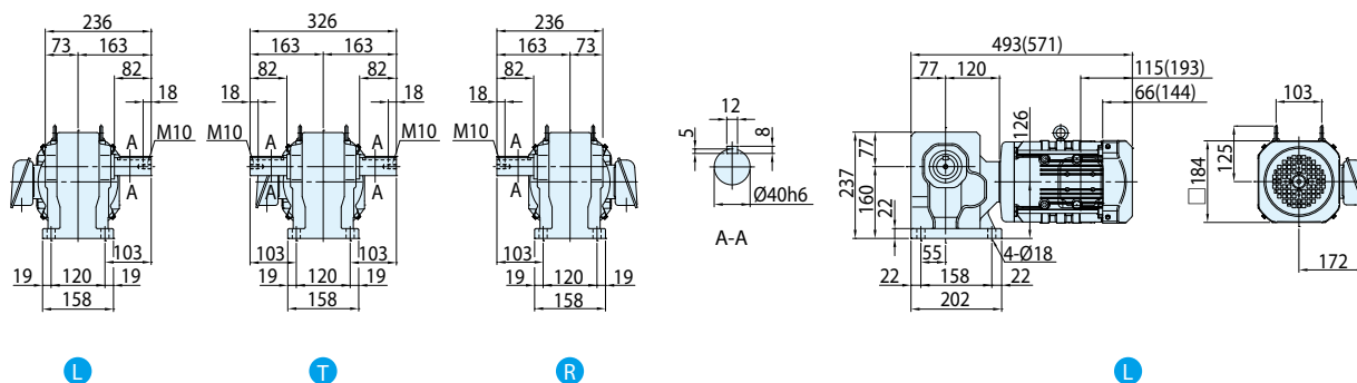
图E445 RNHM3-60 \frac{1}{2} -EP-80~120 (RNHM3-60 \frac{1}{2} -EP-B-80~120)
