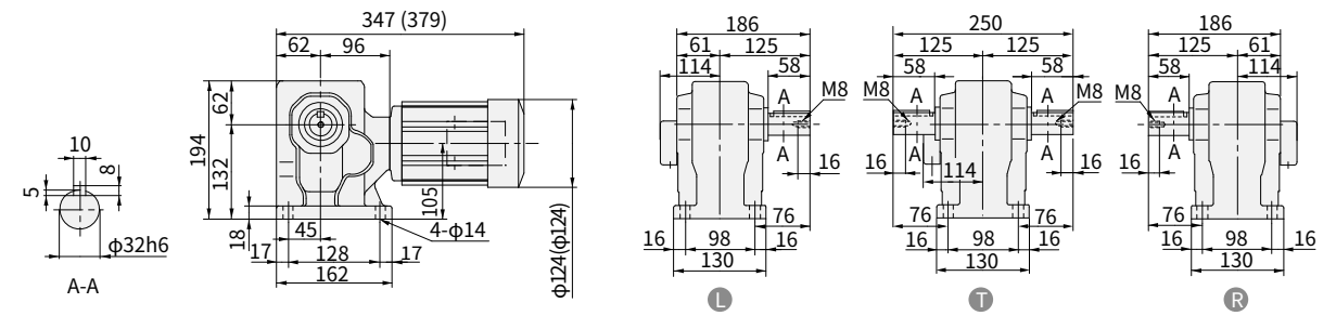
图 E412 RNHM02-40-EP-80~120 (RNHM02-40-EP-B-80~120) 重量 14kg (重量 15kg)
