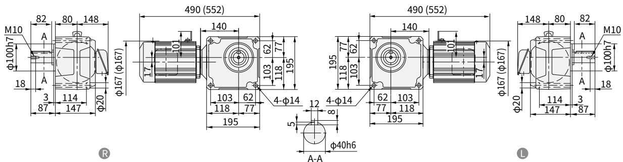
图 E295 RNFM1-53 h -AV-40~80 重量 30kg (RNFM1-53 h -AV-B-40~80) (重量 35kg) · 安装本机器时请使用内六角螺钉 (M12)。 · 请注意电机是否与安装面干涉。
