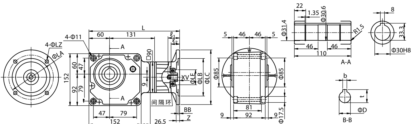
图 E409 RNYX - 1340 - [ 减速比 ]
