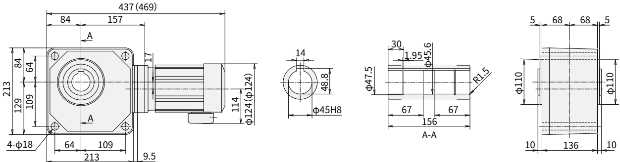
图 E38 RNYM05-1530-80~240 (RNYM05-1530-B-80~240) 重量 23kg (重量 24kg)
