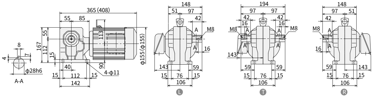
图 E400 RNHM05-370-AV-5~30 (RNHM05-370-AV-B-5~30)
