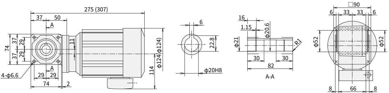
图 E16 RNYM02-1110-5~10 (RNYM02-1110-B-5~10) 重量 6.0kg (重量 7.5kg)
