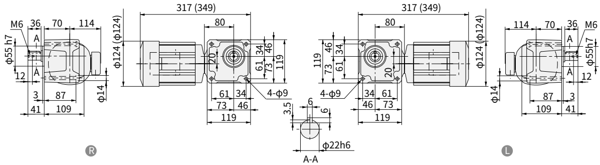
图 E281 RNFM02-270 L R -AV-5~30 重量 9.0kg · 安装本机器时请使用内六角螺钉 (M8)。 (RNFM02-270 L R -AV-B-5~30) (重量 10.5kg)
