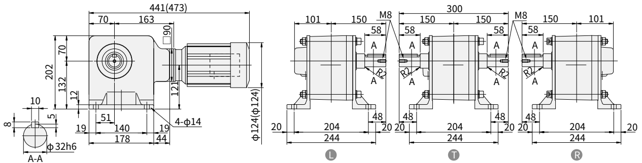
图 E398 RNHM02-1440-AVJ1-720~1440 重量 24.5kg (RNHM02-1440-AVJ1-B-720~1440) (重量 25.5kg)
