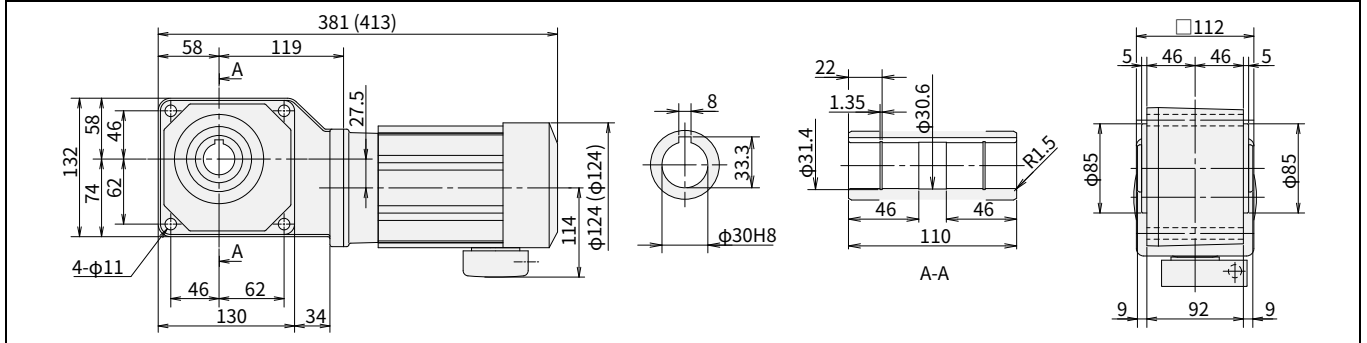
图 E28 RNYM03-1320-40~60 (RNYM03-1320-B-40~60) 重量 11kg (重量 13kg)
