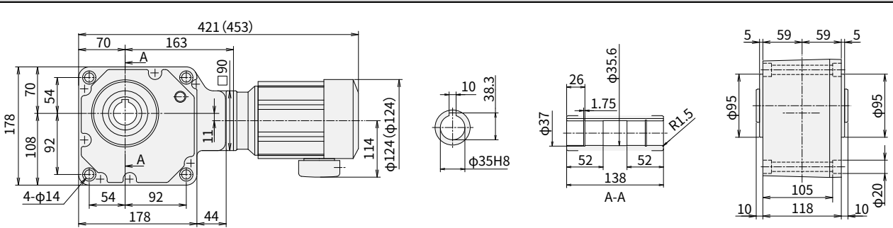
图 E24 RNYM02-1440-300~1440 (RNYM02-1440-B-300~1440)
