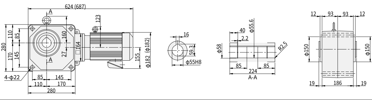
图 E80 RNYM3-1631-150~240 重量 57kg (RNYM3-1631-B-150~240) (重量 63kg)
