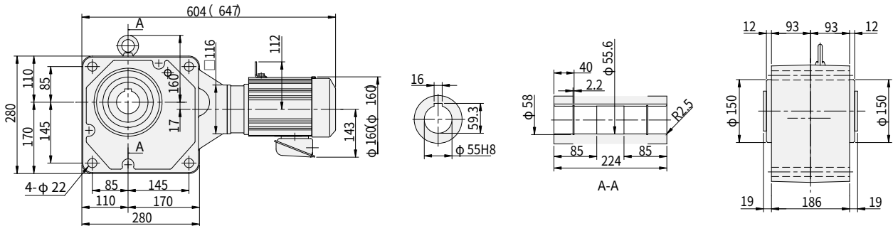
图 E165 RNYM05-1640-EP-300~1440 (RNYM05-1640-EP-B-300~1440) 重量 68kg (重量 70kg)
