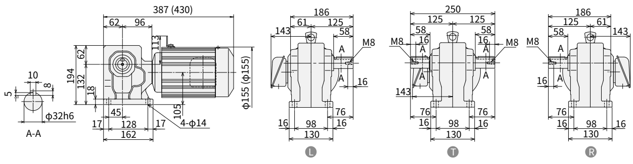
图 E427 RNHM05-43-EP-40~60 重量 17kg (RNHM05-43-EP-B-40~60) (重量 20kg)
