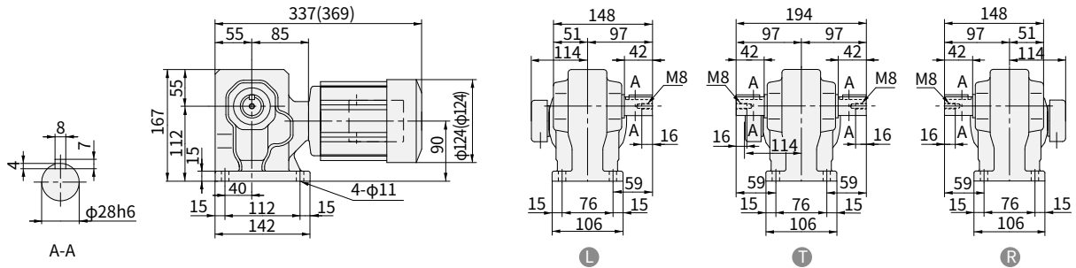
图 E419 RNHM03-33-EP-40~60 (RNHM03-33-EP-B-40~60) 重量 11kg (重量 12kg)
