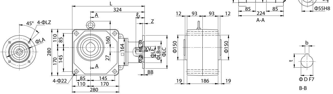
图 E416 RNYX - 1630 - [ 减速比 ]
