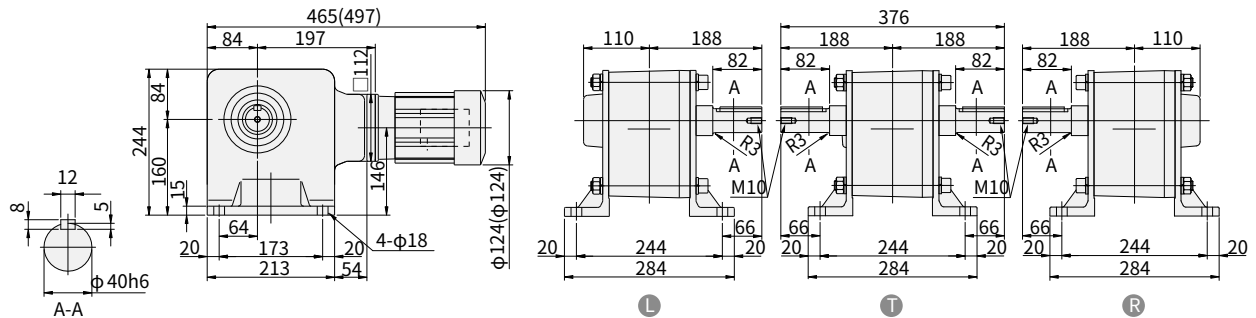
图 E352 RNHM02-1540 h -J1-300~480 重量 39kg (RNHM02-1540 b -J1-B-300~480) (重量 40kg)
