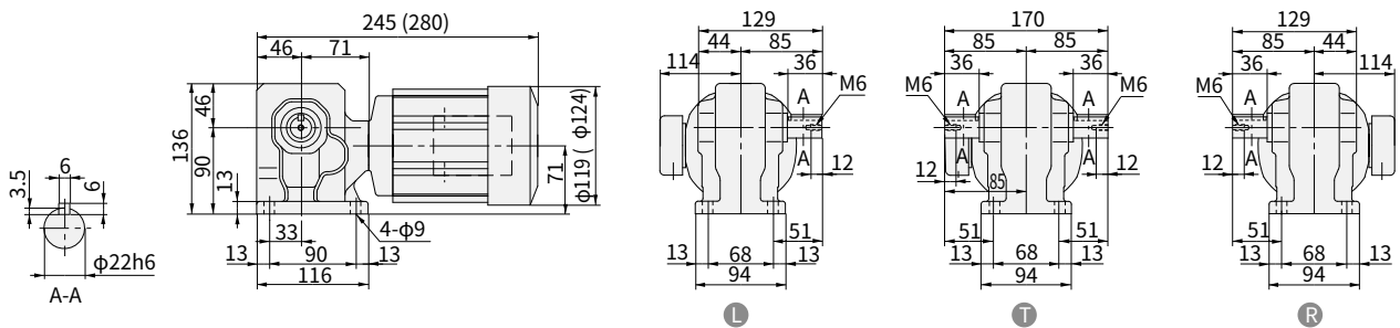
图 E343 RNHM01-20 8 -80~120 (RNHM01-20 B -80~120) 重量 6.5kg (重量 8.0kg)
