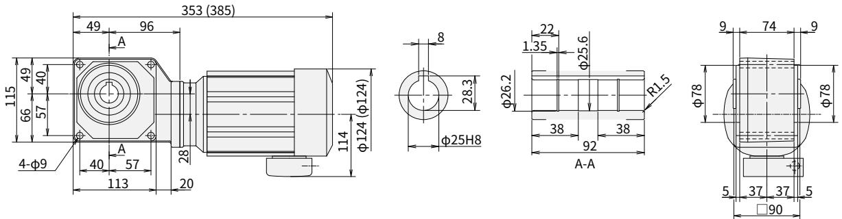
图 E141 RNYM02-1220-EP-5~15 (RNYM02-1220-EP-B-5~15)
