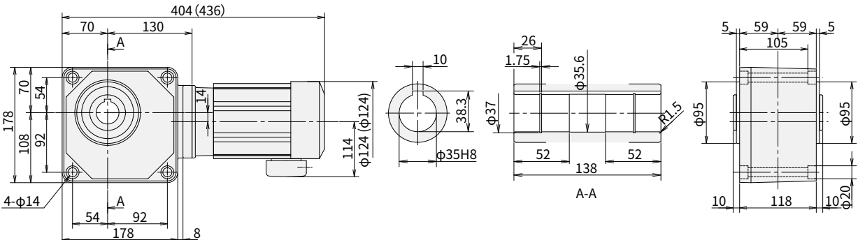
图 E146 RNYM02-1430-EP-80~240 重量 16kg (RNYM02-1430-EP-B-80~240) (重量 17kg)
