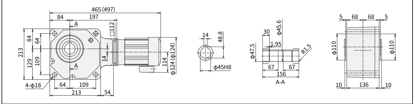
图 E25 RNYM02-1540-300~1440 (RNYM02-1540-B-300~1440) 重量 24.5kg (重量 25.5kg)
