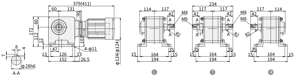
图 E390 RNHM01-1340- AVJ1-720~1440 (RNHM01-1340- AVJ1-B-720~1440 ) 重量 16kg (重量 17kg)
