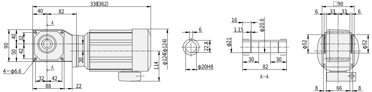
图 E140 RNYM02-1120-EP-5~15 (RNYM02-1120-EP-B-5~15)
