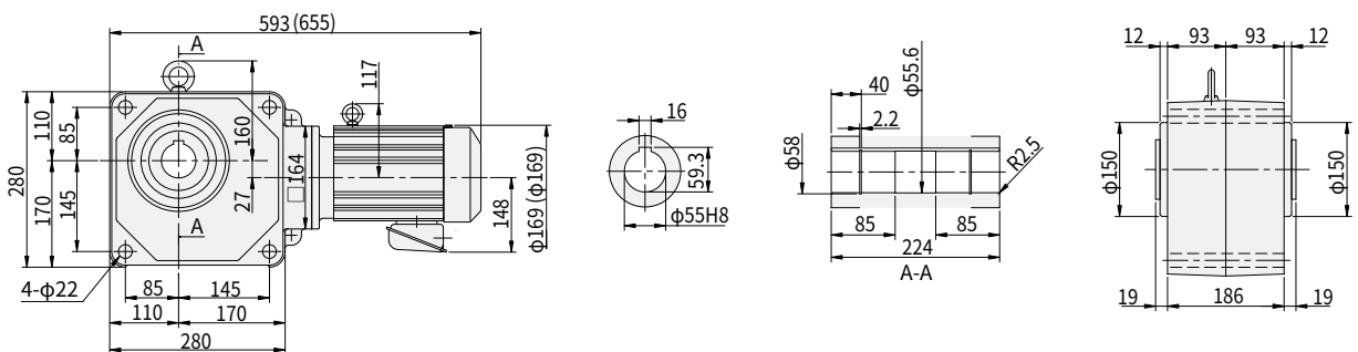
图 E71 RNYM2-1630-80~120 (RNYM2-1630-B-100~120) 重量 52kg (重量 56kg)
