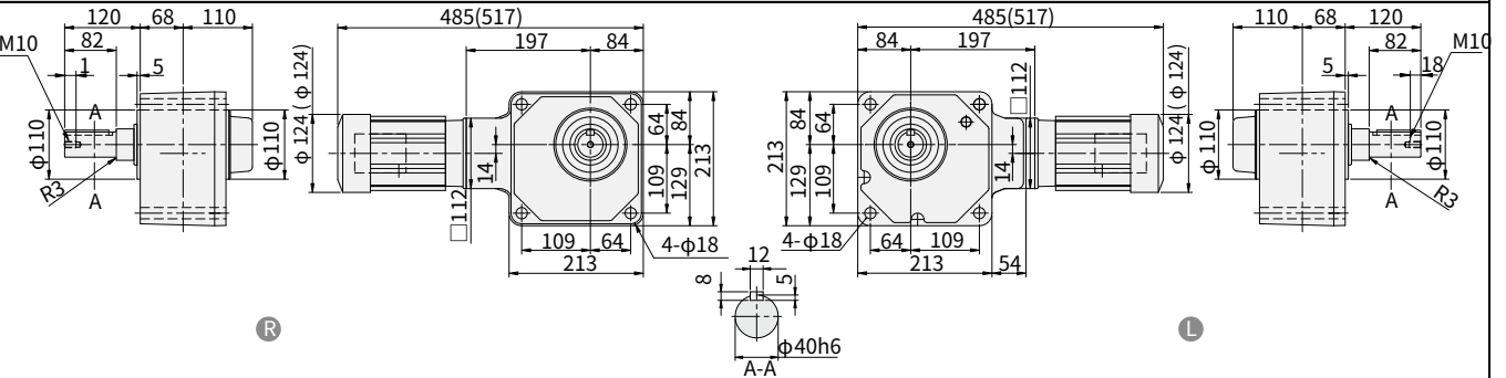
图 E306 RNFM02-1540 R -EPX1-300~600 重量 29kg · 安装本机器时请使用内六角螺钉 (M16)。 (RNFM02-1540 L -EPX1-B-300~600) (重量 30kg)
