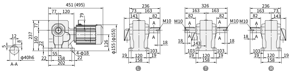
图 E403 RNHM05-55-AV-150~240 (RNHM05-55-AV-B-150~240)
