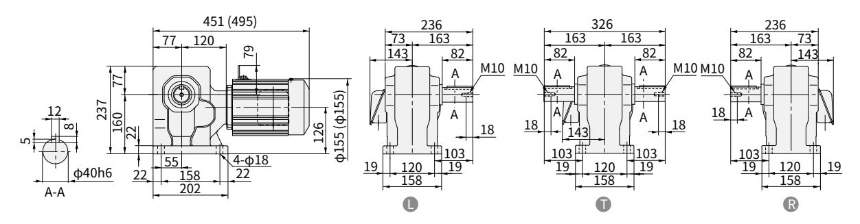
图 E429 RNHM05-55-EP-150~240 重量 25kg (RNHM05-55-EP-B-150~240) (重量 28kg)
