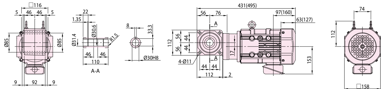
图 E166 RNYM08-1310-EP-5~10 (RNYM08-1310-EP-B-5~10)
