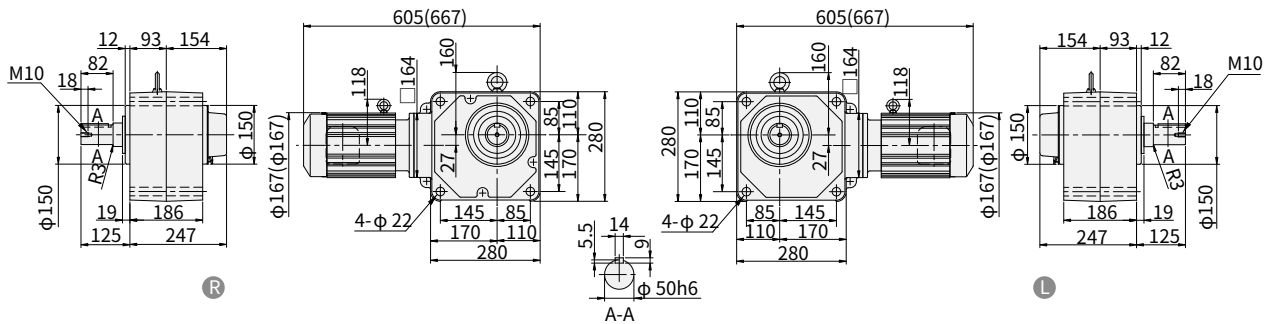
图 E269 RNFM2-1631 L R -X1-150~240 重量 58kg (RNFM2-1631 L R -X1-B-150~240) (重量 62kg) · 安装本机器时请使用内六角螺钉 (M20)。
