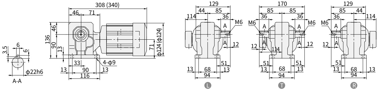
图 E410 RNHM02-270-EP-5~30 (RNHM02-270-EP-B-5~30) 重量 8.5kg (重量 10kg)
