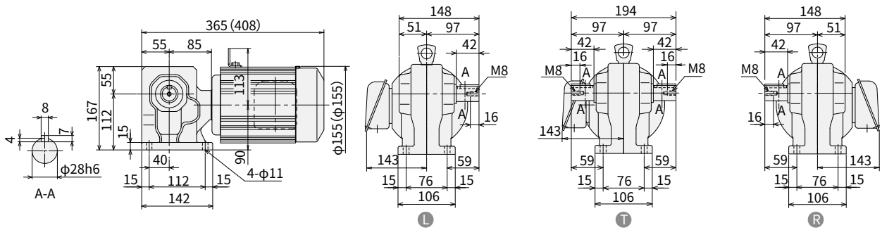
图 E426 RNHM05-370-EP-5~30 重量 13.5kg (RNHM05-370-EP-B-5~30) (重量 16.5kg)
