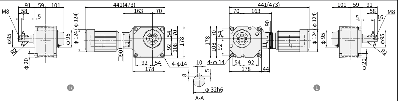
图 E307 RNFM02-1440 R -EPX1-720~1440 重量 18.5kg · 安装本机器时请使用内六角螺钉 (M12)。 (RNFM02-1440 L -EPX1-B-720~1440) (重量 19.5kg)
