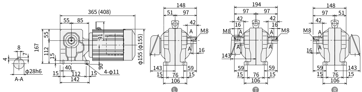
图 E369 RNHM1-370 h -5~30 重量 13.5kg (RNHM1-370 B -B-5~30) (重量 16.5kg)
