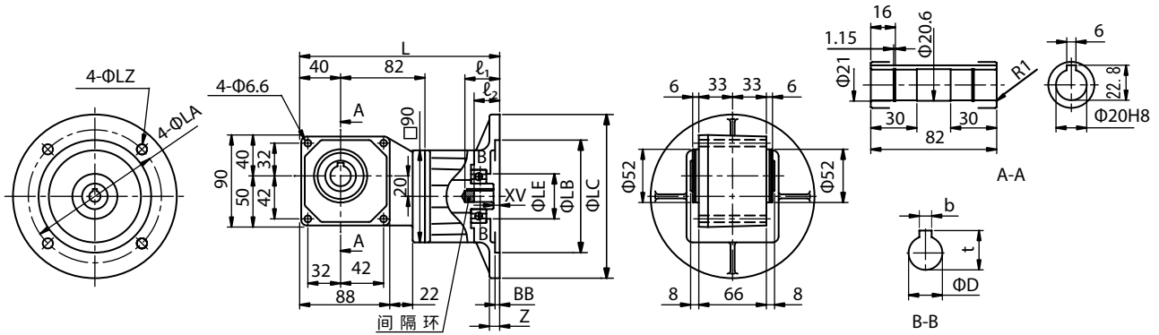
图 E404 RNYX - 1120 - [ 减速比 ]
