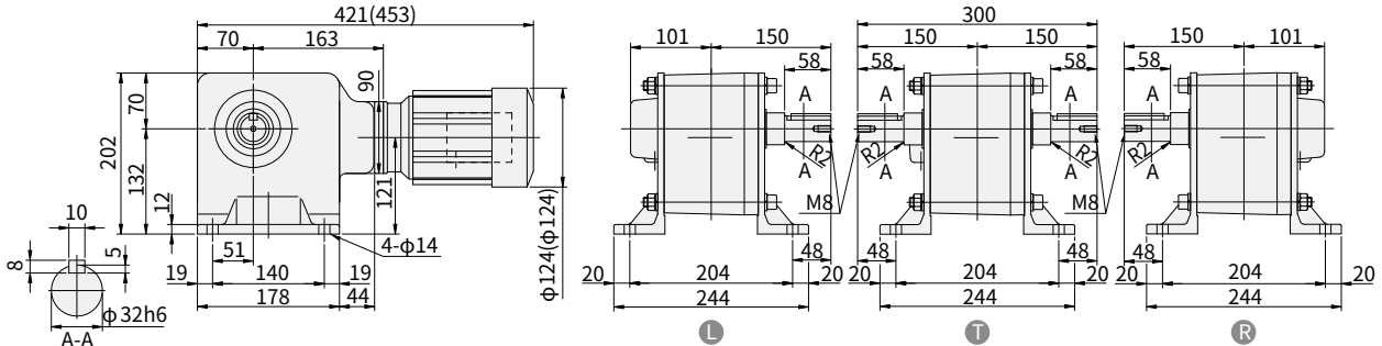
图 E389 RNHM01-1440- AVJ1-300~600 (RNHM01-1440- AVJ1-B-300~600 ) 重量 23kg (重量 24.5kg)
