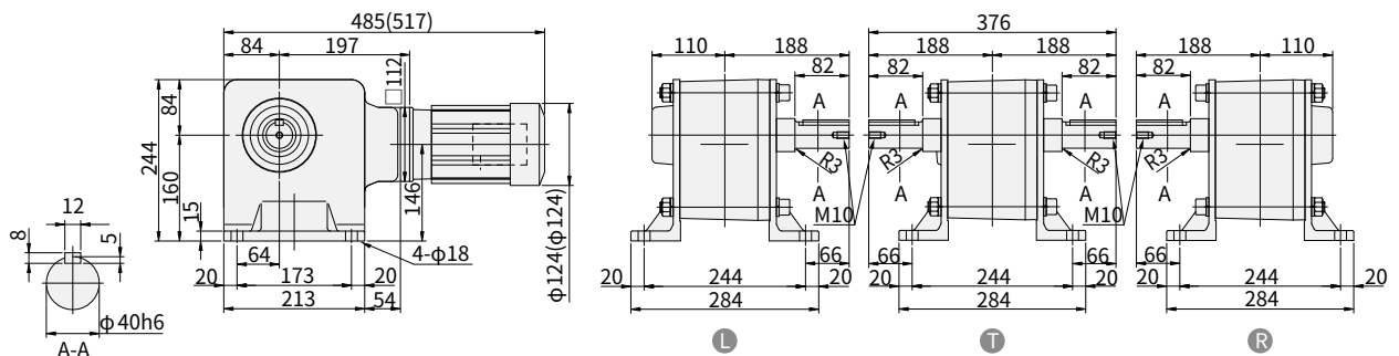
图 E399 RNHM02-1540-AVJ1-720~1440 重量 41kg (RNHM02-1540-AVJ1-B-720~1440) (重量 42kg)
