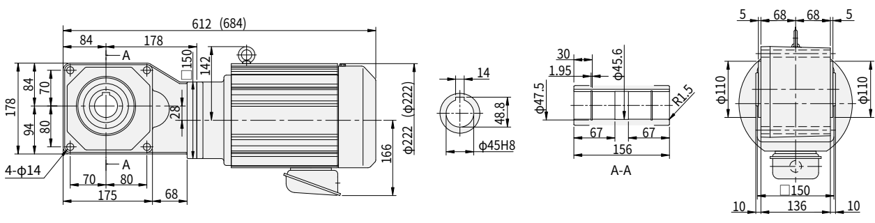
图 E133 RNYM3-1521-AV-5~25 (RNYM3-1521-AV-B-5~25) 重量 50kg (重量 61kg)
