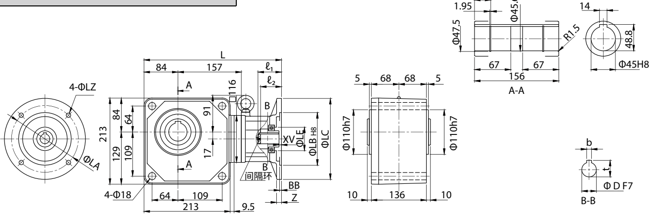
图 E414 RNYX - 1531 - [ 减速比 ]
