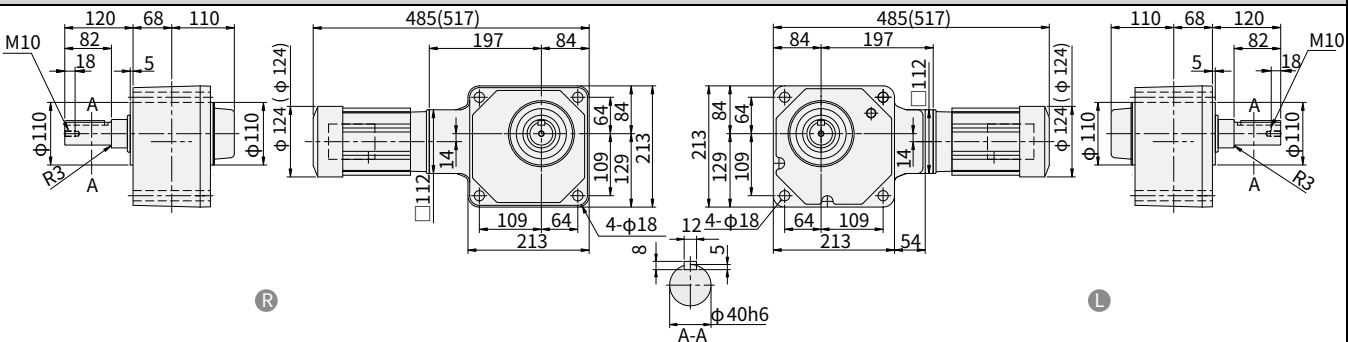
图 E316 RNFM03-1540 h -EPX1-720~1440 重量 29kg · 安装本机器时请使用内六角螺钉 (M16)。 (RNFM03-1540 h -EPX1-B-720~1440) (重量 30kg)
