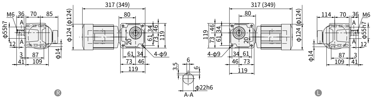
图 E244 RNFM05-270 L R -5~30 重量 9.0kg · 安装本机器时请使用内六角螺钉 (M8)。 (RNFM05-270 L R -B-5~30) (重量 10.5kg)
