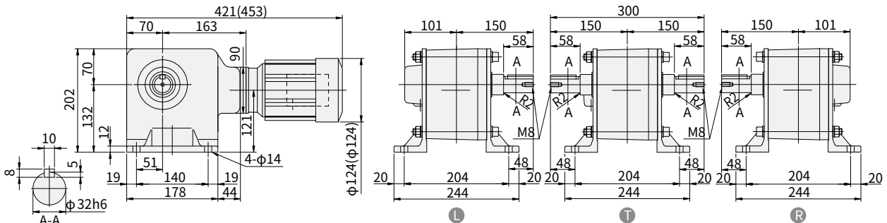
图 E391 RNHM01-1440- AVJ1-720~1440 (RNHM01-1440- AVJ1-B-720~1440 ) 重量 23kg (重量 24.5kg)
