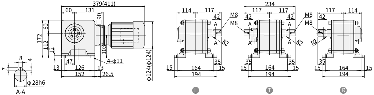
图 E388 RNHM01-1340- AVJ1-300~600 (RNHM01-1340- AVJ1-B-300~600 ) 重量 16kg (重量 17kg)
