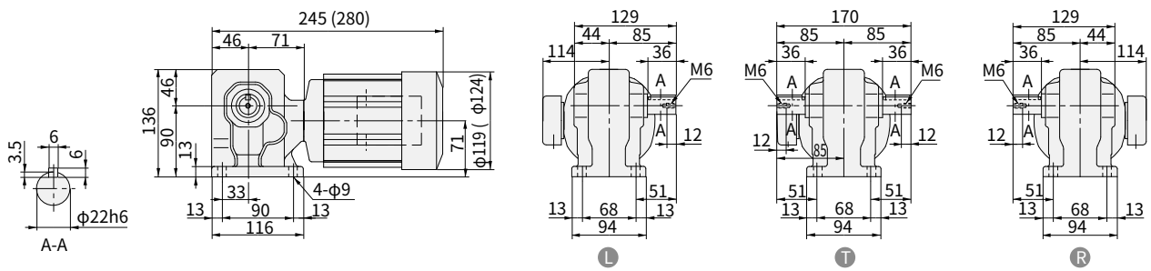
图 E344 RNHM01-25 8 -150~240 (RNHM01-25 B -150~240) 重量 6.5kg (重量 8.0kg)
