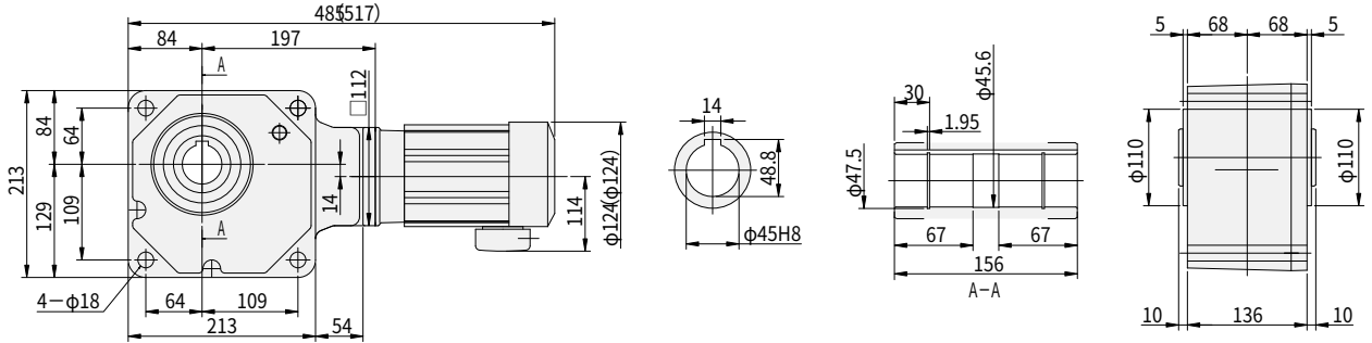
图 E116 RNYM02-1540-AV-720~1440 重量 26kg (RNYM02-1540-AV-B-720~1440) (重量 27.5kg)
