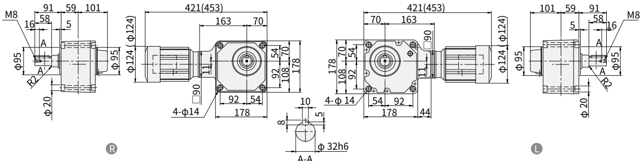
图 E237 RNFM02-1440 h -X1-600~1440 重量 17kg · 安装本机器时请使用内六角螺钉 (M12)。 (RNFM02-1440 h -X1-B-600~1440) (重量 18.5kg)
