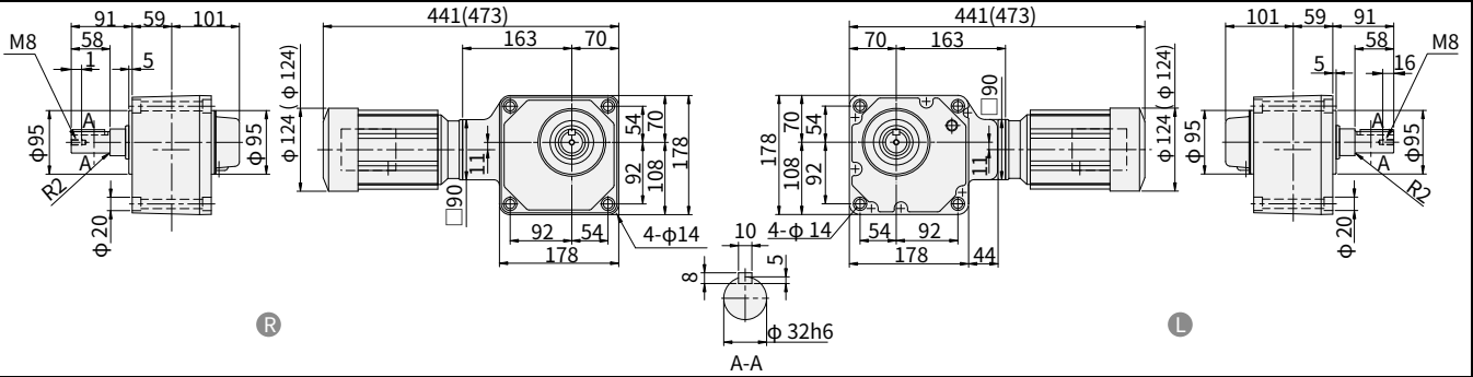
图 E305 RNFM02-1440 R -EPX1-300~600 重量 18.5kg · 安装本机器时请使用内六角螺钉 (M12)。 (RNFM02-1440 L -EPX1-B-300~600) (重量 19.5kg)
