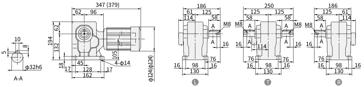
图 E420 RNHM03-40-EP-80~120 (RNHM03-40-EP-B-80~120) 重量 14kg (重量 15kg)
