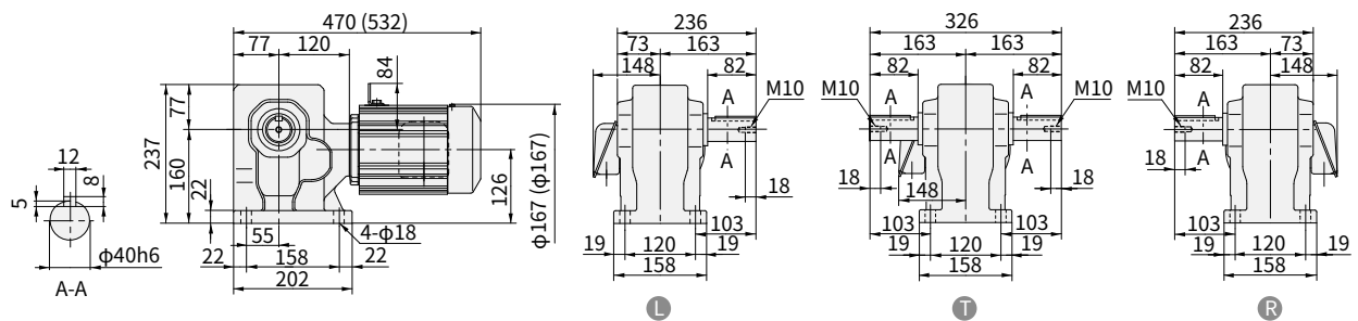
图 E377 RNHM2-53 1/2 -40~80 (RNHM2-53 1/2 -B-40~80) 重量 30kg (重量 34kg)
