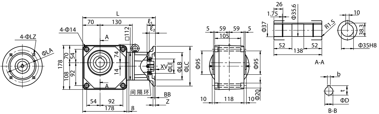
图 E411 RNYX - 1430 - [ 减速比 ]
